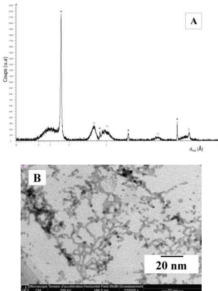
Figure III-21 : (A) Diffractogramme des rayons X (Mo K \alpha ) de l'échantillon de Pt déposé sur le support de laboratoire. Pt est représenté par \circ (fiche ASTM n°04-0802) et C par * (fiche ASTM n°26-1076). (B) Image obtenue en microscopie électronique en transmission correspondante
