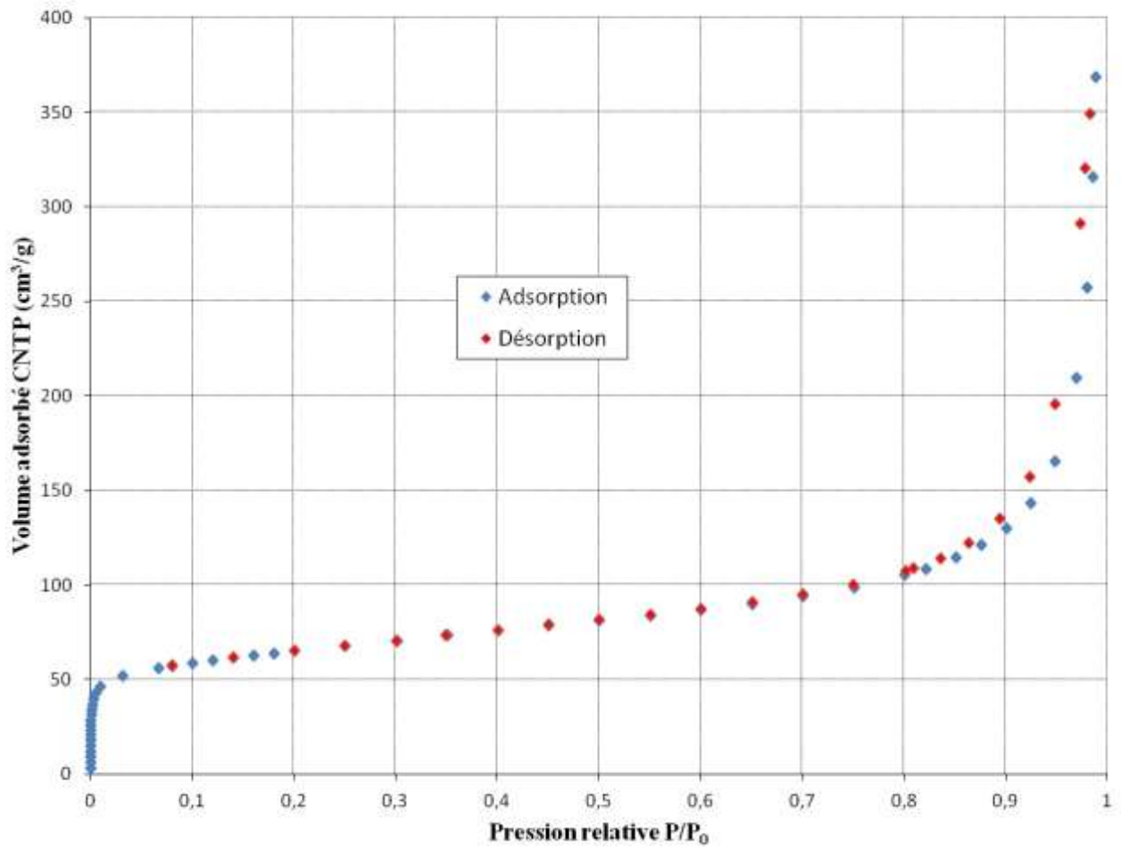
Figure II-8 : Isotherme d'adsorption-désorption de N 2 sur le Vulcan® à 77 K
