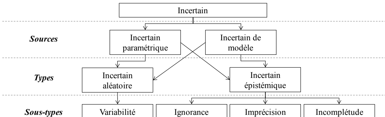
Figure 2-2. Classification de l'incertain
