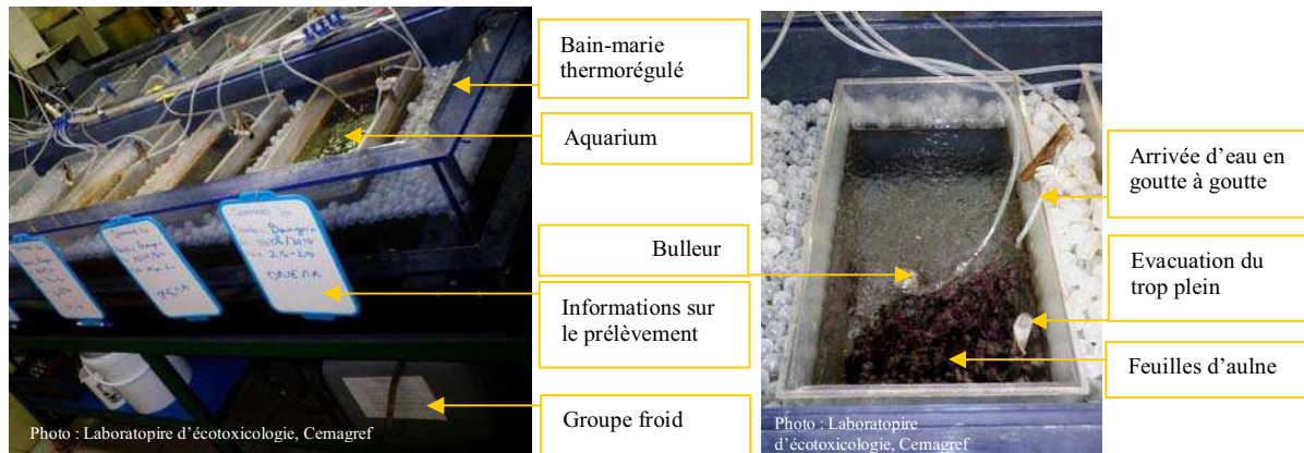
Figure II-5 : Système de stabulation des gammares au laboratoire
