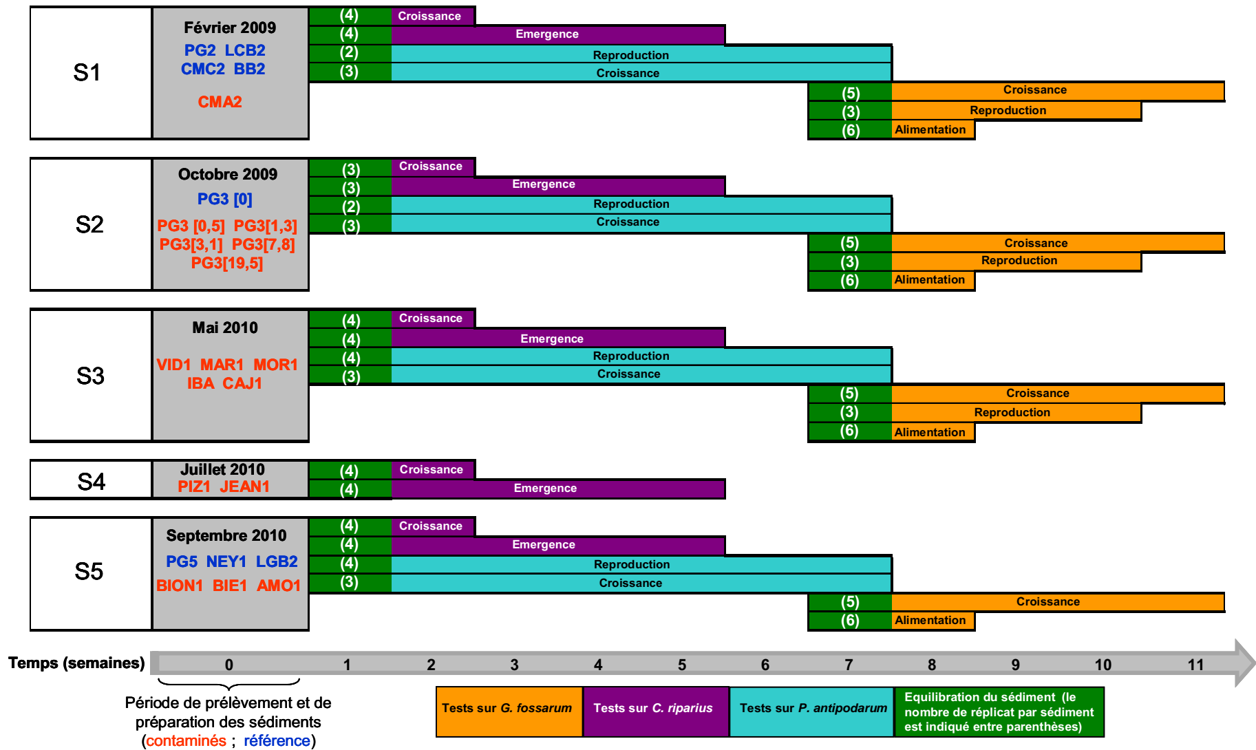
Figure III-5 : Schéma organisationnel des cinq séries d'expérimentation (S1 à S5)
