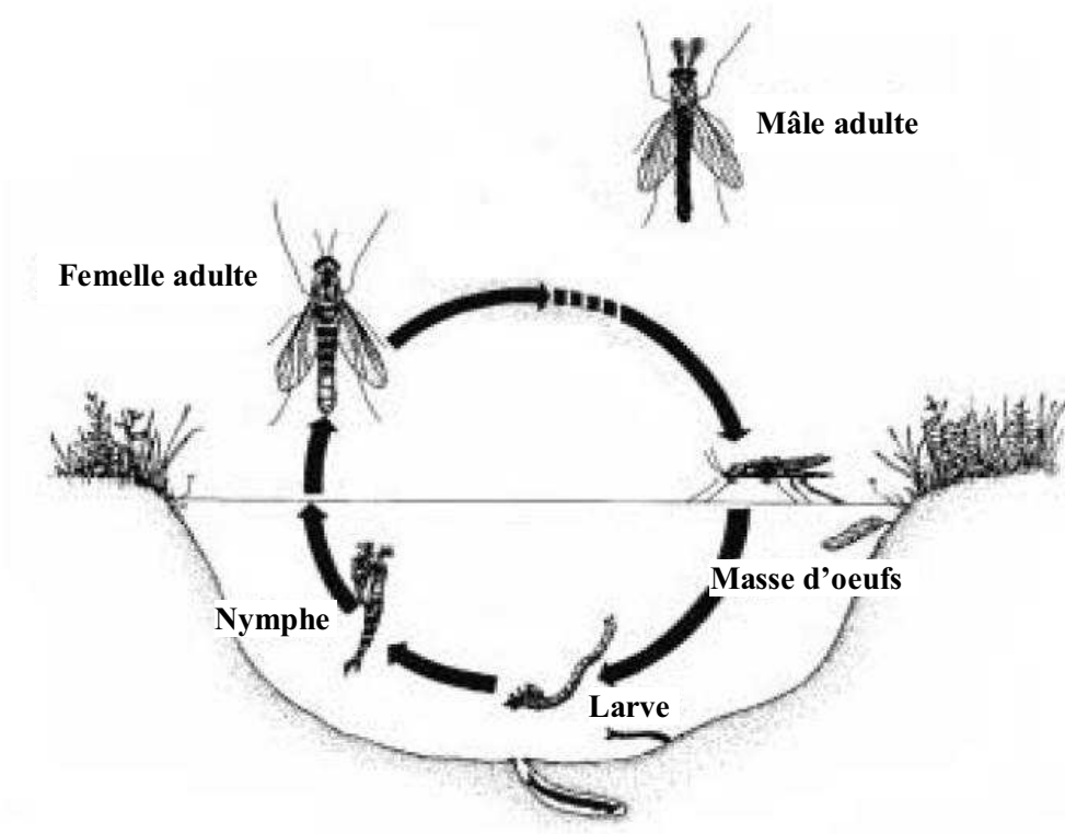
Figure I-10 : Schéma simplifié du cycle de vie de C. riparius , d'après Ducrot (2005).
