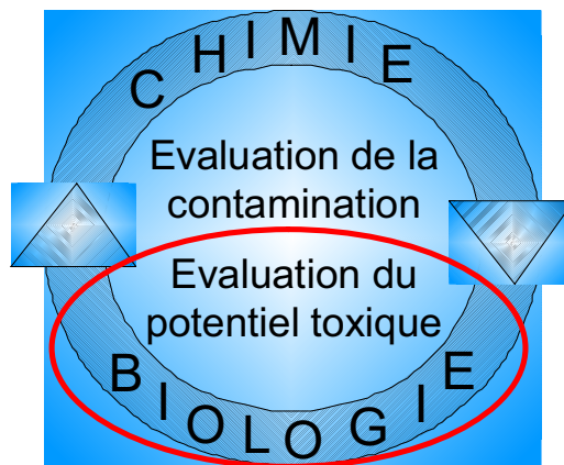
Figure III-1 : Méthode d'évaluation de la qualité des sédiments.
