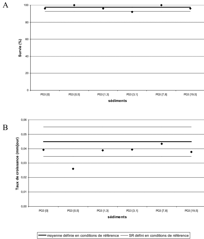
Figure V-16 : Résultats des tests de croissance des juvéniles P. antipodarum exposés aux sédiments dopés positionnés par rapport à la moyenne et aux SR minimum et maximum définis en conditions de référence. A : Taux de survie ; B : Taux de croissance.
