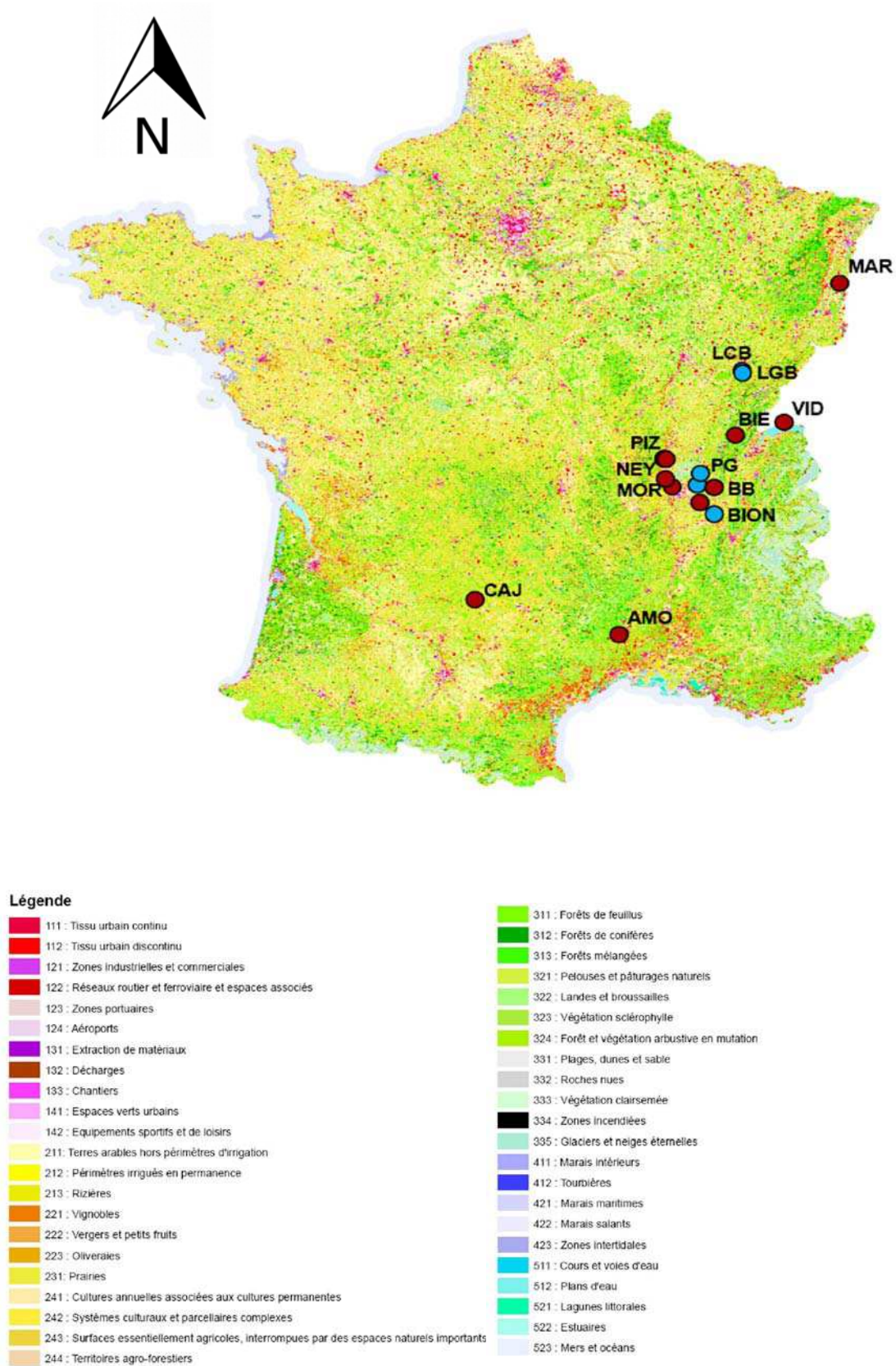
Figure III-2 : Localisation géographique des sites de prélèvement selon l'occupation des sols en France (source : Corine Land Cover, http://sd1878-2.sivit.org/ ).
