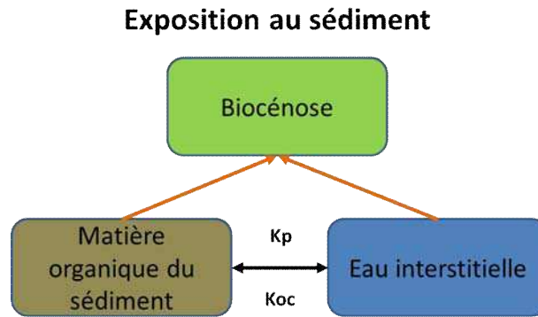
Figure I-3 : Equilibre de partition des contaminants, d'après Di Toro et al. (1991).
