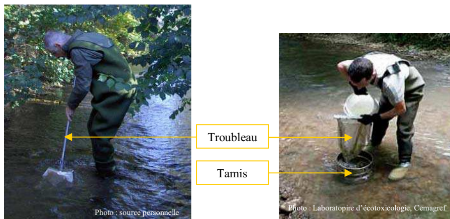
Figure II-4 : Prélèvement au troubleau et tamisage des gammarus
