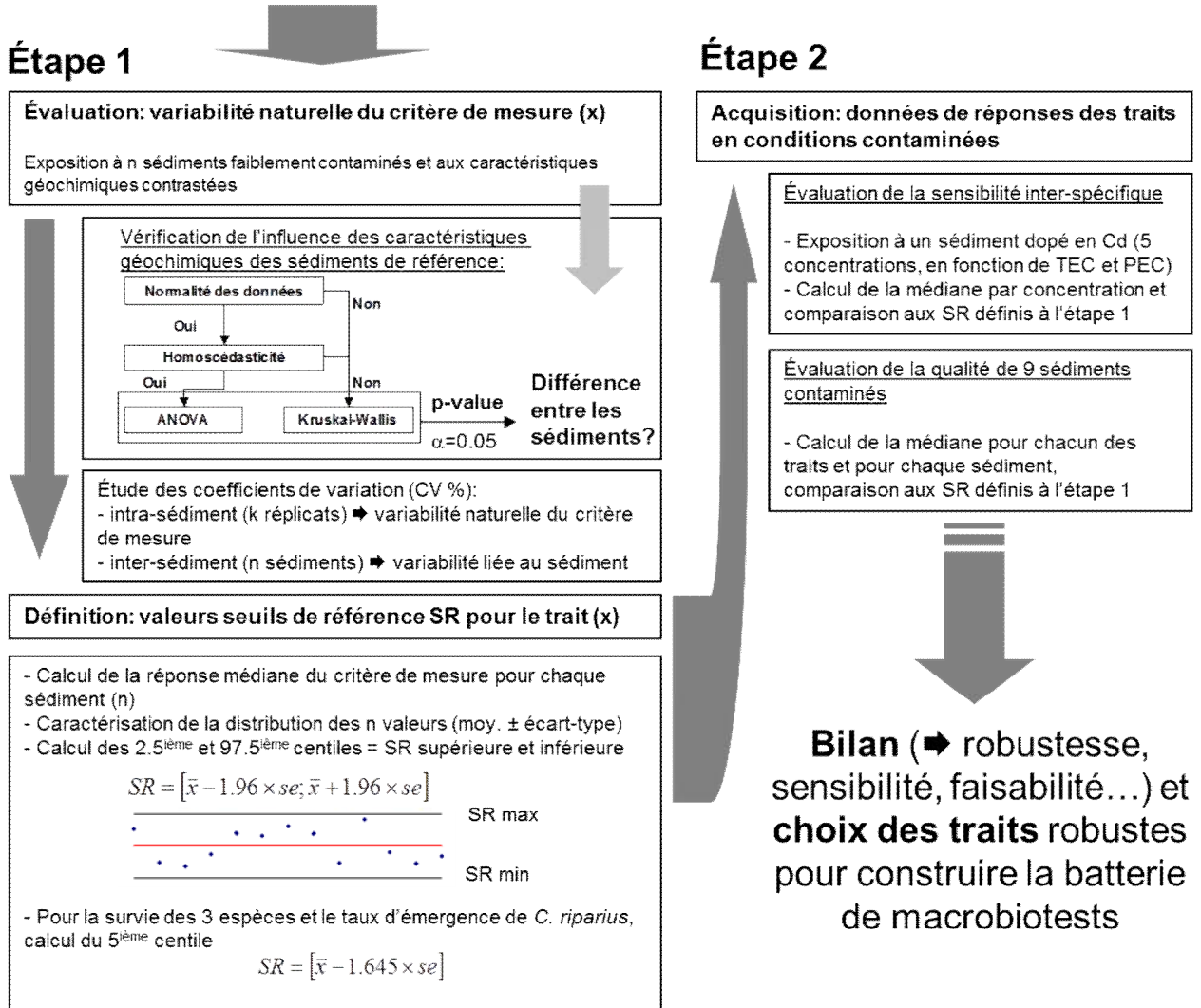
Figure II-12 : Démarche statistique employée (méthode A) pour la définition des seuils de référence (SR) en conditions de référence (étape 1) auxquels seront confrontées les réponses obtenues sur sédiments contaminés (étape 2).
