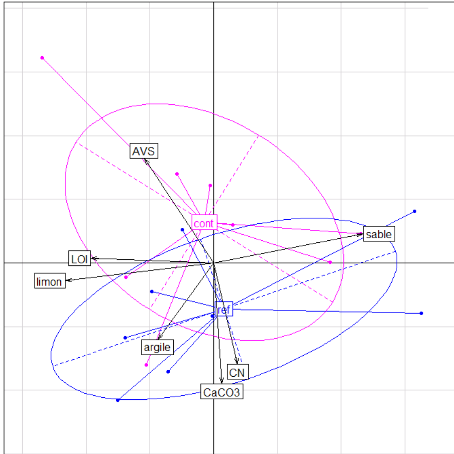
Figure III-3 : Représentation par une ACP des principales caractéristiques géochimiques (texture, AVS, LOI, C/N et carbonates) des 2 catégories de sédiments (références en bleu et contaminés en rose).
