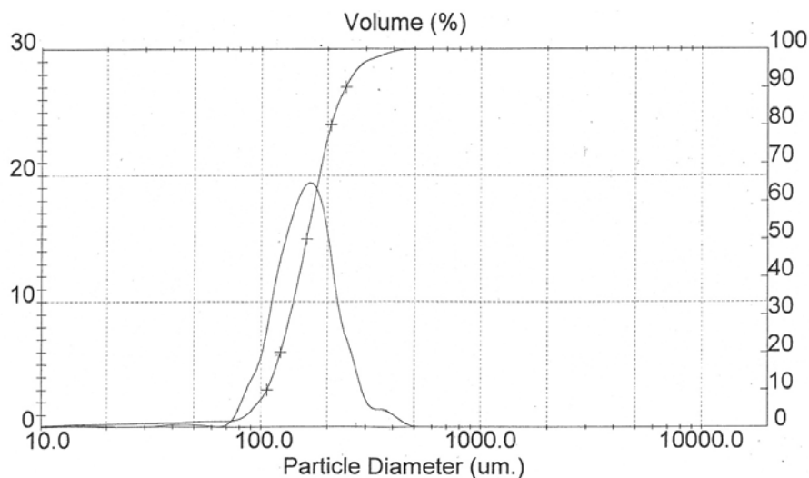
Figure II.5 – Fonctions de distribution et de répartition granulométriques en volume
