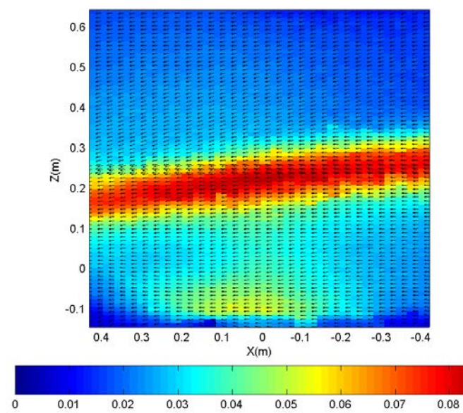
Figure VI.12 – DES, k - \epsilon réalisable, vitesse moyenne V_{xz}/R\omega (Plan Y=17\text{cm} , 500 \text{ tr.min}^{-1} )
