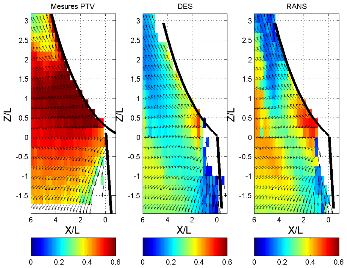
Figure VI.27 – Carte de vitesses moyennes des particules ( V_{xz}/R\omega ) obtenue par les mesures et par les différentes méthodes numériques ( 500 \text{ tr.min}^{-1} , Plan Y=6\text{mm} )
