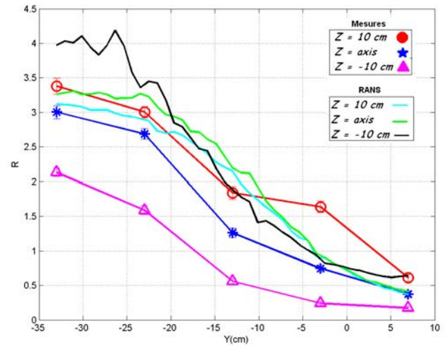
Figure VI.43 – Évolution du profil de concentration (R) suivant l'axe Y (Mesures-RANS( k - \epsilon réalisable), 500 \text{ tr.min}^{-1} , X = 50 \text{ cm} )
