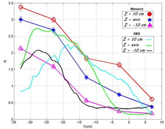
Figure VI.45 – Évolution du profil de concentration (R) suivant l'axe Y (Mesures-DES( k - \epsilon réalisable), 500 \text{ tr.min}^{-1} , X = 50 \text{ cm} )
