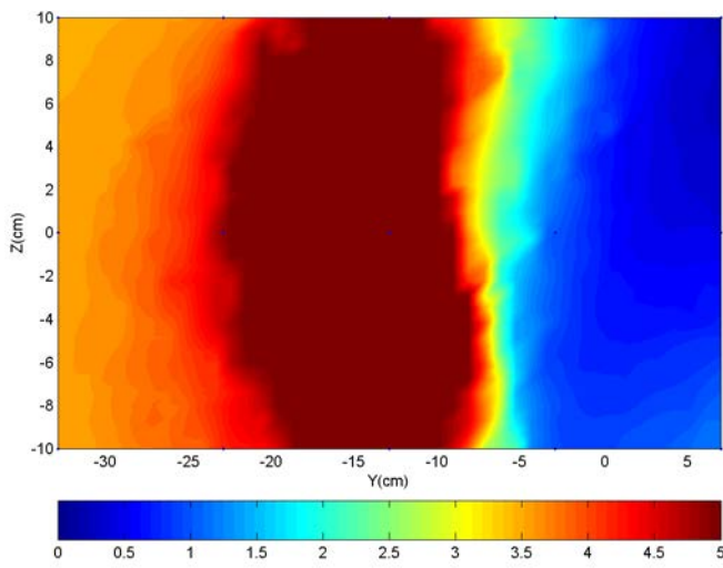
Figure VI.32 – Carte de concentration représentée par le rapport R (RANS, k - \epsilon réalisable, 500 \text{ tr.min}^{-1} , X = 25\text{cm} )
