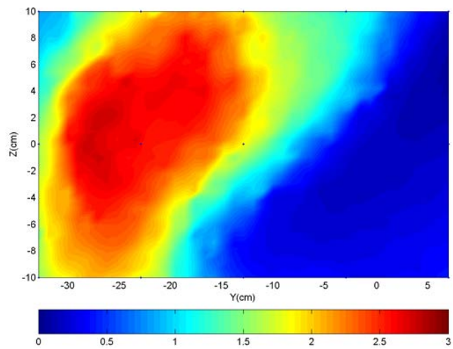
Figure VI.35 – Carte de concentration représentée par le rapport R (DES, k - \epsilon réalisable, 500 \text{ tr.min}^{-1} , X = 50\text{cm} )
