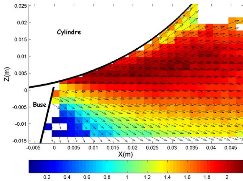
Figure VI.2 – Plan axial ( Y=0 ) : vitesse moyenne des particules ( \text{m.s}^{-1} )
