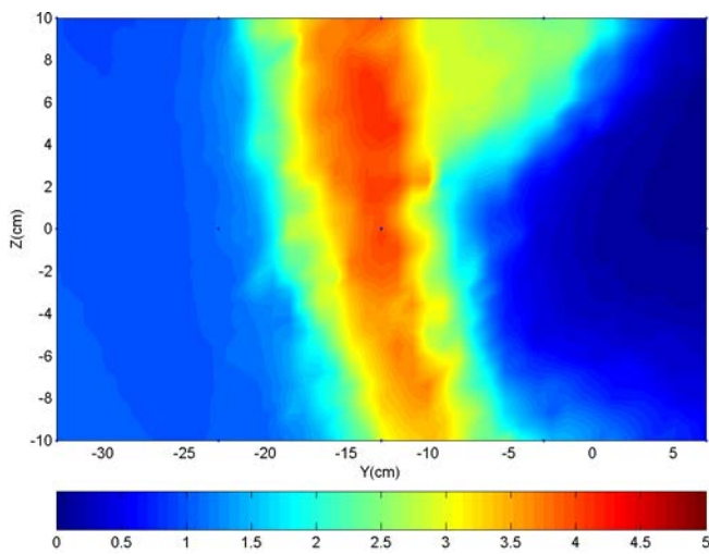
Figure VI.34 – Carte de concentration représentée par le rapport R (DES, k - \epsilon réalisable, 500 \text{ tr.min}^{-1} , X = 25\text{cm} )
