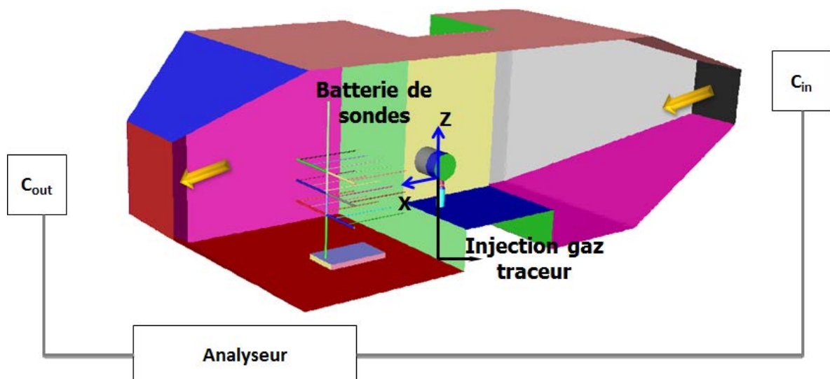
Figure IV.1 – Dispositif de traçage gazeux
