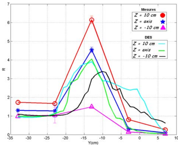
Figure VI.44 – Évolution du profil de concentration (R) suivant l'axe Y (Mesures-DES( k - \epsilon réalisable), 500 \text{ tr.min}^{-1} , X = 25 \text{ cm} )
