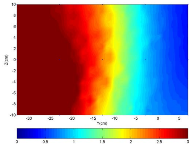
Figure VI.33 – Carte de concentration représentée par le rapport R (RANS, k - \epsilon réalisable, 500 \text{ tr.min}^{-1} , X = 50\text{cm} )
