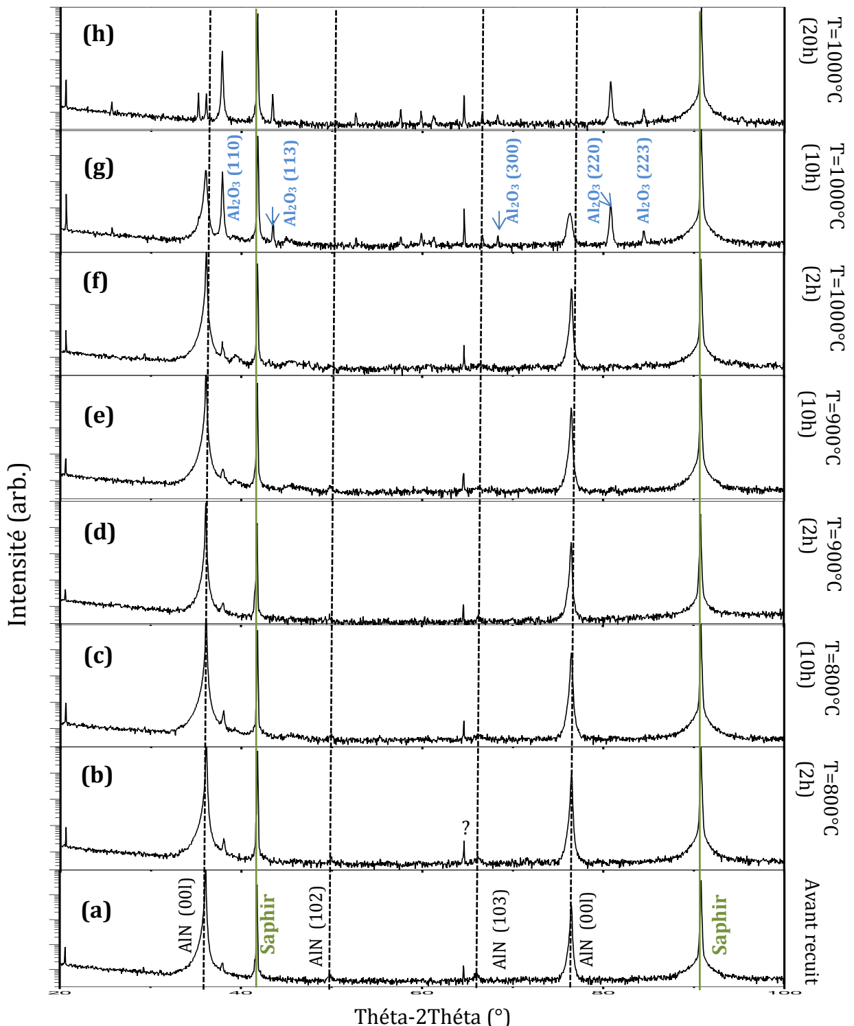
Figure IV-27: Clichés de diffraction en theta-2théta réalisés sur l'hétérostructure AlN(1 \mu m)/IDT/AlN/Saphir: (a) avant recuit (b) 800°C pendant 2h (c) 800°C pendant 10h (d) 900°C pendant 2h (e) 900°C pendant 10h (f) 1000°C pendant 2h, (g) 1000°C pendant 10h (h) 1000°C pendant 20h. Les lignes en pointillées et celles en continue vert indiquent les différentes réflexions détectées de l'AlN (Fiche JCPDS Annexe 4) et les positions des réflexions (006) et (0012) du saphir ( \alpha -Al 2 O 3 ) (Fiche JCPDS Annexe 5) respectivement.
