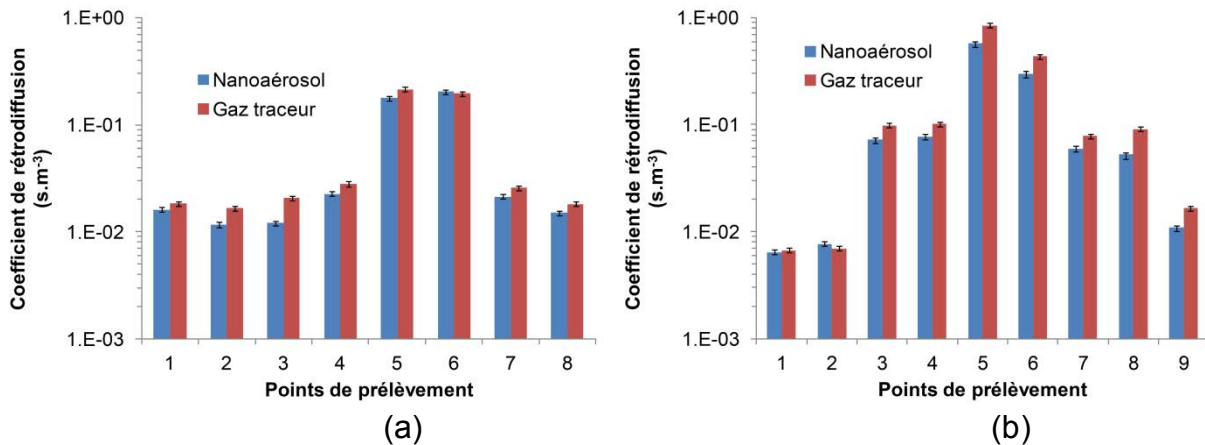
figure 2-38 : Coefficients de rétrodiffusion pour une vitesse d'aspiration v=0,4 \text{ m.s}^{-1} : (a) sans mannequin et (b) avec mannequin
