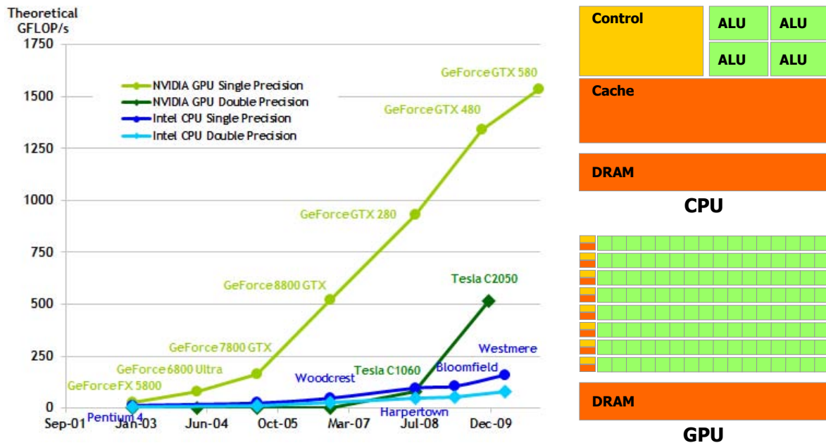
(a) Évolution de la puissance de calcul théorique.
