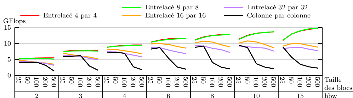
Figure 2.13 : Influence de l'entrelacement des données sur les performances. Machine test : 1 \times 4 SandyBridge – exécution parallèle CPU : SSE et OpenMP
