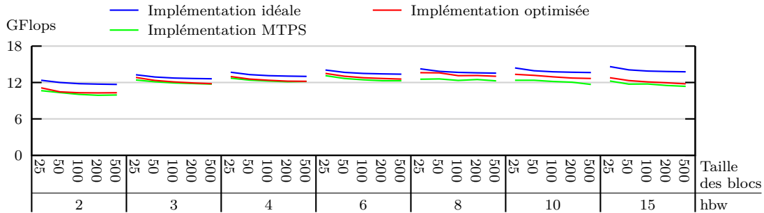
Figure 6.14 : Performances de MTPS sur Fermi.
