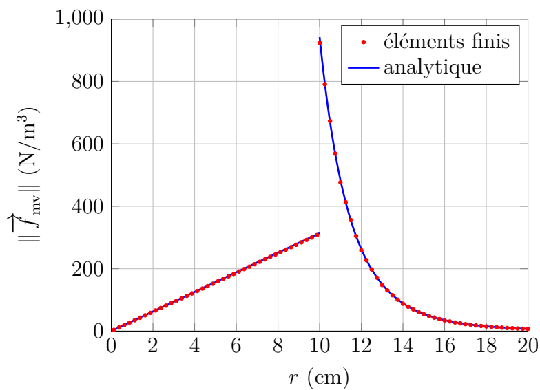
Figure 4.16 Comparaison entre les résultats de la simulation et l'expression analytique de la norme de la force volumique magnétique pour R = 10 cm et p = 2
