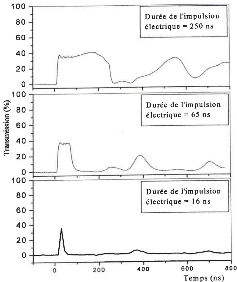
Figure 4.3: Réponse du \text{LiNbO}_3 (échantillon LNCr) à une tension impulsionnelle d'amplitude 800 V. Dépendance des résonances acoustiques en fonction de la durée de l'impulsion électrique.
