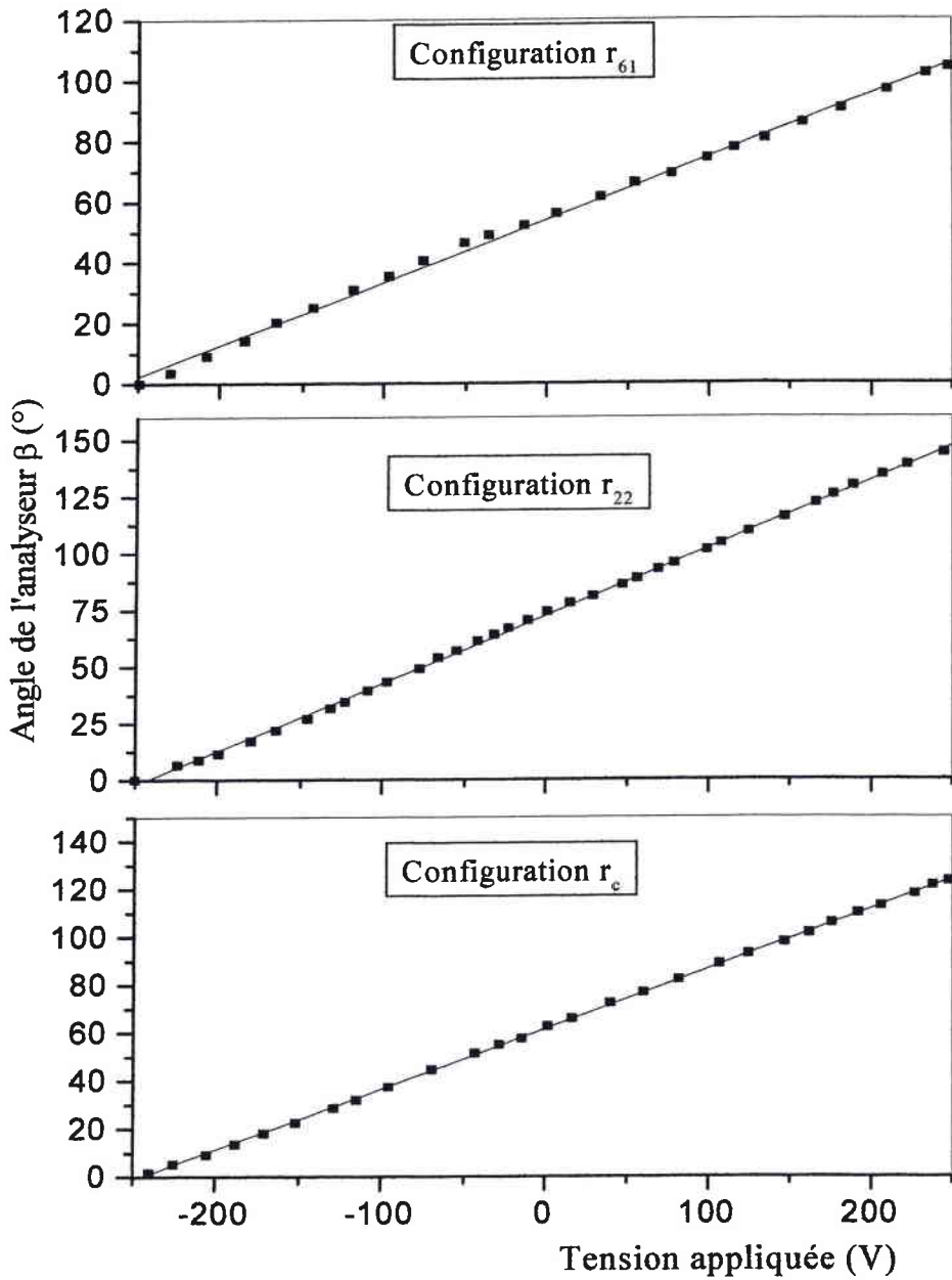
Figure 2.6: Méthode statique : Variation de l'angle \beta_{2\theta} de compensation en fonction de la tension continue V_{ac} appliquée aux cristaux LNCr_{61} , LNCr_{22} et LNCr_c dans les configurations r_{61} , r_{22} et r_c respectivement.
