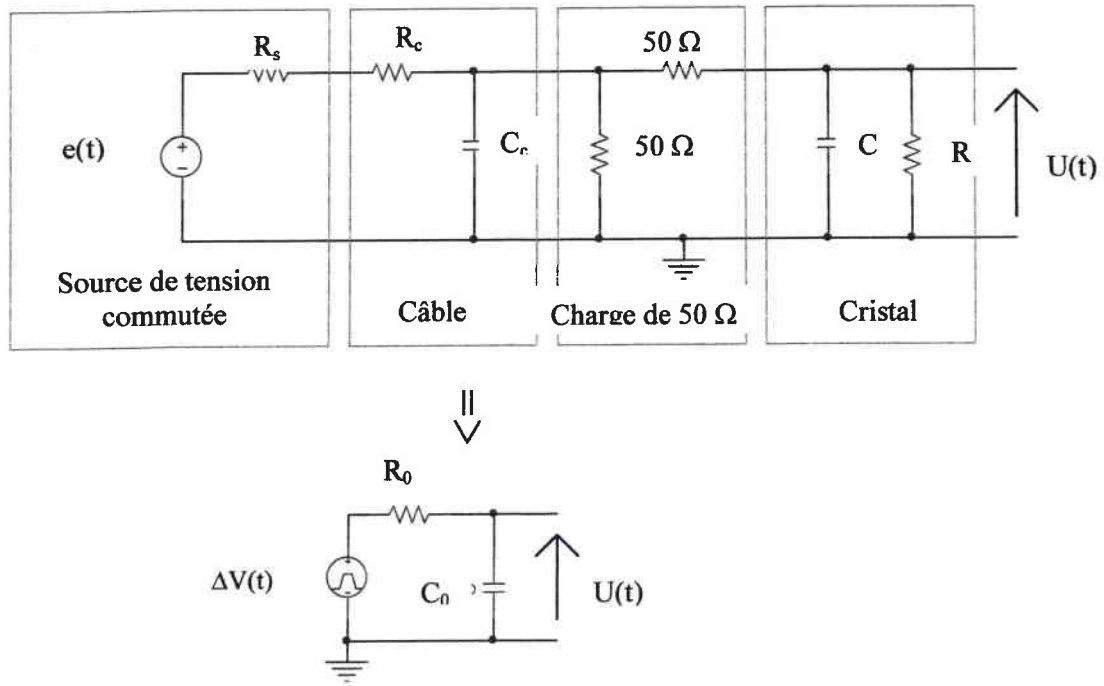
Figure 3.10: Montage électrique schématisant le cristal, les câbles et la source haute tension. En utilisant le théorème de Thévenin et en prenant en compte les effets selfiques ( L_d ), on ramène le circuit à un circuit RLC du second ordre d'amplitude \Delta V(t) et de résistance équivalente R_0 .
