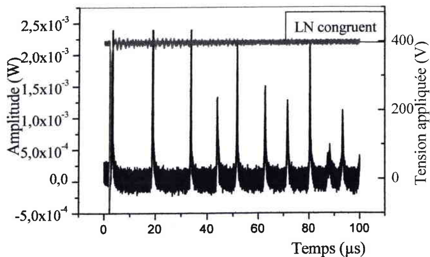
Figure 4. 12 : Rebonds provoqués par les résonances acoustiques. En rouge l'impulsion électrique de durée 150 ns. En noir les résonances acoustiques. Le taux de pompage est de 400 mW, la puissance moyenne est de 45 \mu W.
