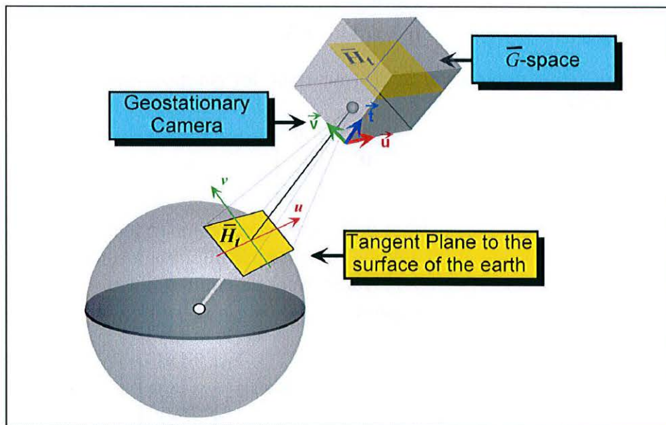
FIG. 2.3 : L'espace paramétrique \overline{G} vu comme un empilement continu d'images de l'espace de dépôt, prises depuis un satellite géostationnaire au-dessus de la zone étudiée, au cours du temps ([Mallet, 2004]).
