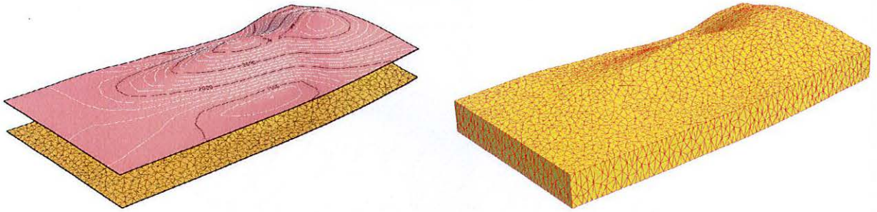
FIG. 3.14 : Modèle initial de l'anticlinal de Split Mountain, Utah (données IFP), exagération verticale \times 2 . À gauche, les deux horizons triangulés reconstitués à partir des données de terrain, avec des courbes de niveau sur l'horizon supérieur et le maillage sur l'horizon inférieur. À droite, le volume tétraédrique correspondant.
