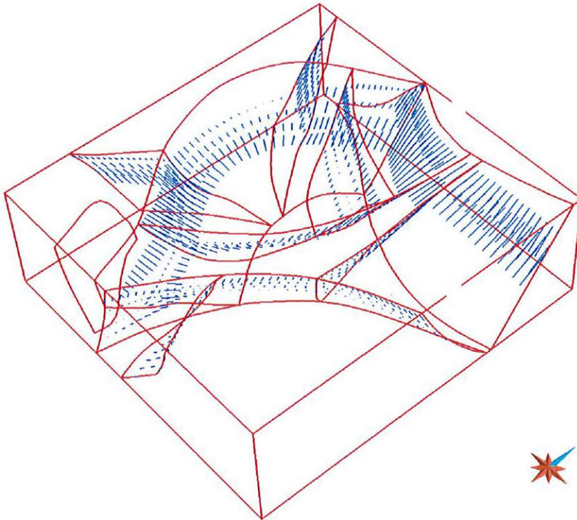
FIG. 4.9 : Ensemble de vecteurs rejet générés automatiquement à différentes valeurs de temps dans un volume tétraédrique. Le calcul par surface d'isovaleur de t génère des vecteurs rejet situés dans des plans particuliers et non pas répartis de manière homogène sur les surfaces de faille.
