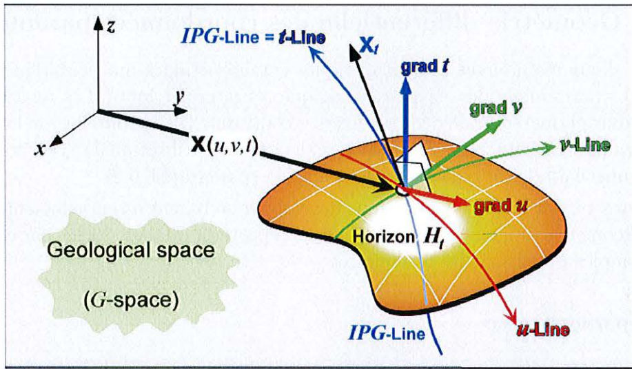
FIG. 2.6 : Repère paramétrique (x_u, x_v, x_t) de l'espace géologique. Les vecteurs x_u et x_v sont tangents à l'horizon H_t au point x et chacun des trois vecteurs est tangent à la ligne d'isovaleur correspondante ([Mallet, 2004]).
