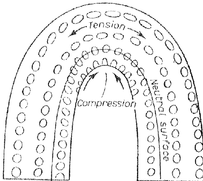
FIG. 2.11 : Définition de la fibre neutre dans une couche en pure bending. Un volume élémentaire (figuré par les cercles) situé sur cette fibre ou surface en 3D, n'est pas déformé. Les volumes au-dessus sont dilatés, ceux en dessous sont comprimés ([Hills, 1963], p. 220).
