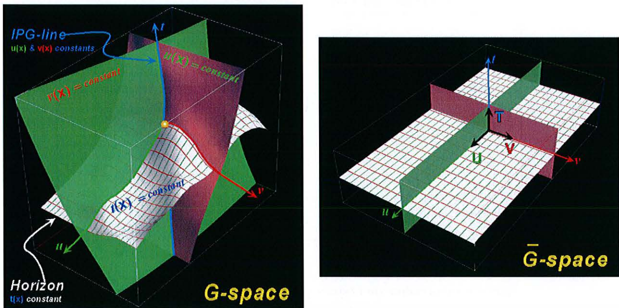
FIG. 2.5 : Lignes de paramétrisation u , v et t dans l'espace géologique. L'intersection dans l'espace géologique (à gauche) de trois surfaces d'isovaleurs de u(\mathbf{x}) (en rouge), v(\mathbf{x}) (en vert) et t(\mathbf{x}) (en blanc, les lignes rouges et vertes figurant les traces de surfaces d'isovaleurs de u et de v ) définit des lignes particulières appelées lignes- u , lignes- v et lignes- t ou lignes iso-paléo-géographiques. Dans l'espace paramétrique (à droite), ces surfaces sont planes et ces lignes sont droites, et s'intersectent à angle droit.
