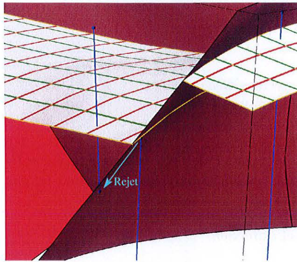
FIG. 3.10 : Fibre intersectant une faille et décalée suivant le vecteur rejet. Les fibres bleues sont extraites depuis l'horizon de référence sur lequel une paramétrisation initiale a été définie (lignes rouges et vertes). À droite, une autre fibre, non affectée par les failles.
