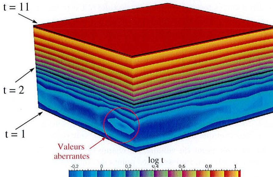
FIG. 3.2 : Influence des valeurs initiales t_i sur le calcul du temps. Des valeurs de t constantes ( t_0 = 1 , t_1 = 2 et t_2 = 11 ) ont été affectées sur trois horizons parallèles, H_0 , H_1 et H_2 , puis le temps a été interpolé dans le volume. Le temps, représenté ici en échelle logarithmique pour mieux mettre en évidence les variations, est erroné entre H_0 et H_1 , car il n'est pas toujours croissant (en particulier dans le cercle rouge). Cette erreur est engendrée par le trop grand écart entre \Delta t_0 et \Delta t_1 pour des couples d'horizons séparés de la même distance \Delta h .
