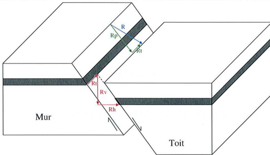
FIG. 4.1 : Modélisation d'un vecteur rejet (en bleu), à l'aide de deux composantes R_p et R_t (en vert) ou de trois composantes R_t , R_v et R_h (en rouge).
