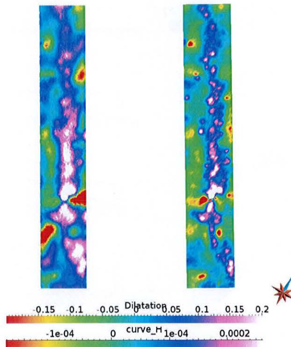
FIG. 5.13 : Comparaison de la dilatation \theta et de la courbure moyenne. À gauche, vue en carte de la dilatation sur le volume, à droite, vue en carte de la courbure gaussienne moyenne sur l'horizon supérieur du modèle. La similarité entre les deux images correspond bien au modèle théorique de déformation en pure bending.
