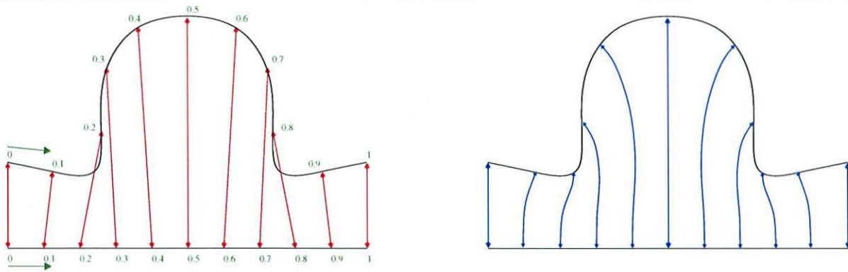
FIG. 4.4 : Vue en coupe de l'association de deux lèvres de faille par des rejets. À gauche, en reliant par un segment des points désignés par les mêmes coordonnées paramétriques (en vert), certains vecteurs rejet peuvent croiser les horizons. À droite, une solution plus réaliste où les rejets sont tracés en suivant les courbures des deux lèvres.
