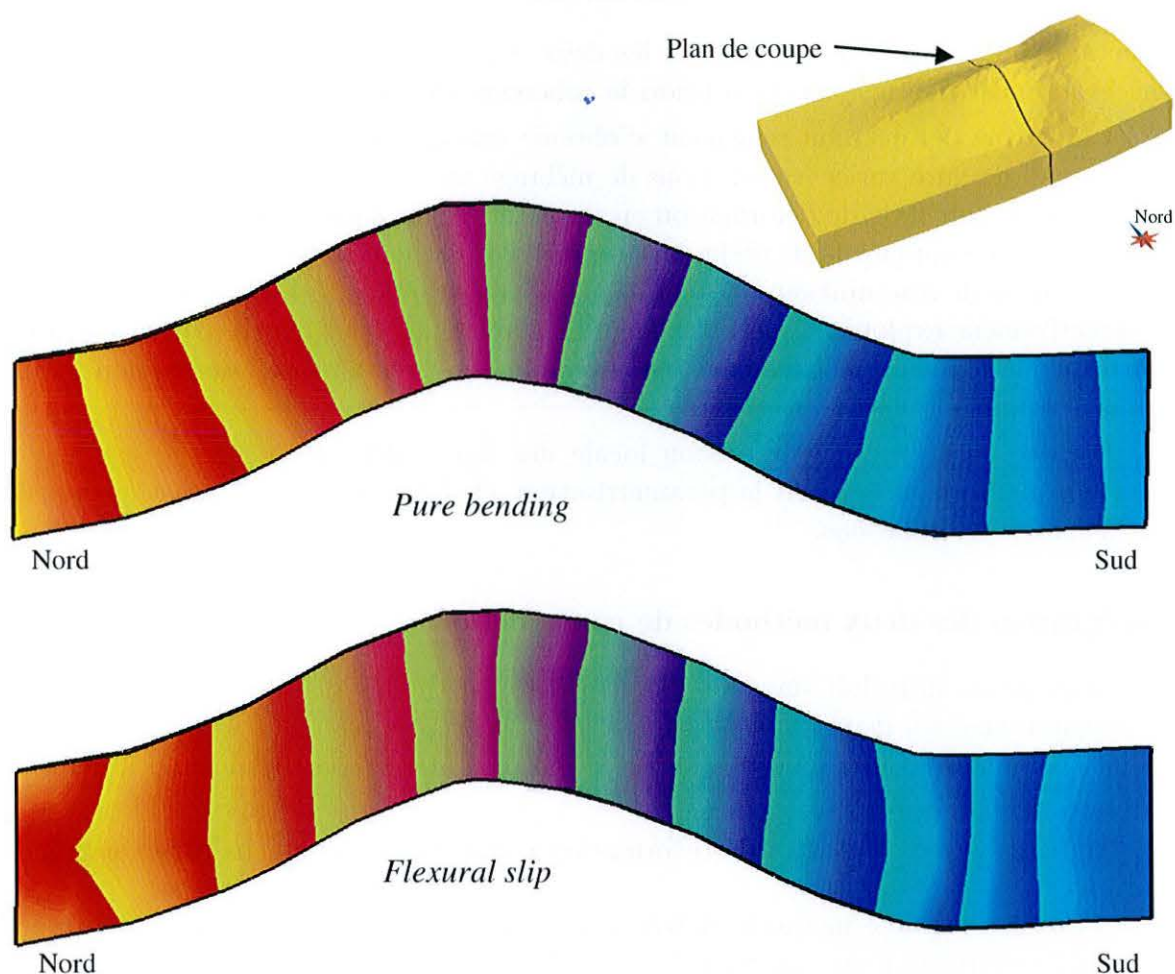
FIG. 3.20 : Comparaison en coupe (exagération verticale \times 2 ) entre les deux contraintes de paramétrisation globale. En haut, la paramétrisation obtenue par orthogonalité 3D, en bas par conformal mapping étendu. Les lignes sont similaires à celles observées suivant les styles de déformation (figures 2.10 et 2.12).
