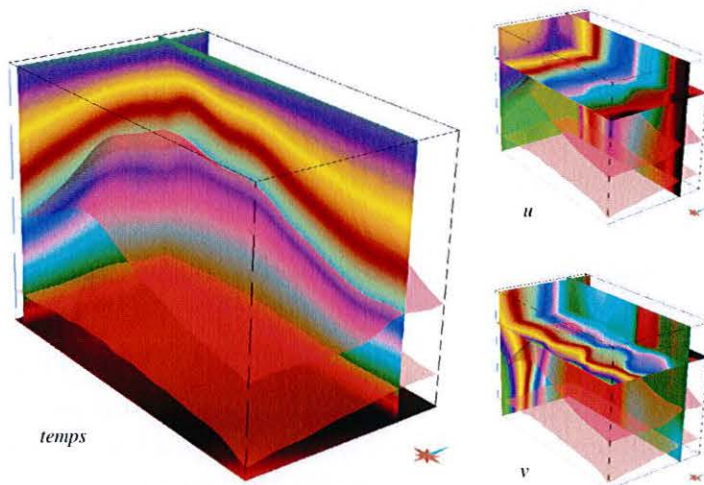
FIG. 3.11 : Contrôle de la densité du champ de fibres par réinitialisation de l'extraction sur chaque horizon. Depuis l'horizon de référence porteur de la paramétrisation 2D (en rouge, au milieu), des fibres sont extraites dans chaque direction jusqu'à l'horizon suivant. La paramétrisation (u, v) est alors interpolée sur cet horizon, avant d'en extraire un nouveau champ de fibres. Le volume est ainsi couvert par une densité de fibres constante (comparer avec la figure 3.8).
