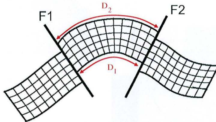
FIG. 1.11 : Vue en coupe d'une grille stratigraphique coupée par deux failles et induisant une erreur dans le calcul des distances. Les longueurs réelles d_1 et d_2 sont différentes, mais sont représentées dans la grille par le même nombre de cellules : elles sont donc considérées comme identiques si une modélisation de propriété est faite suivant cette grille.
