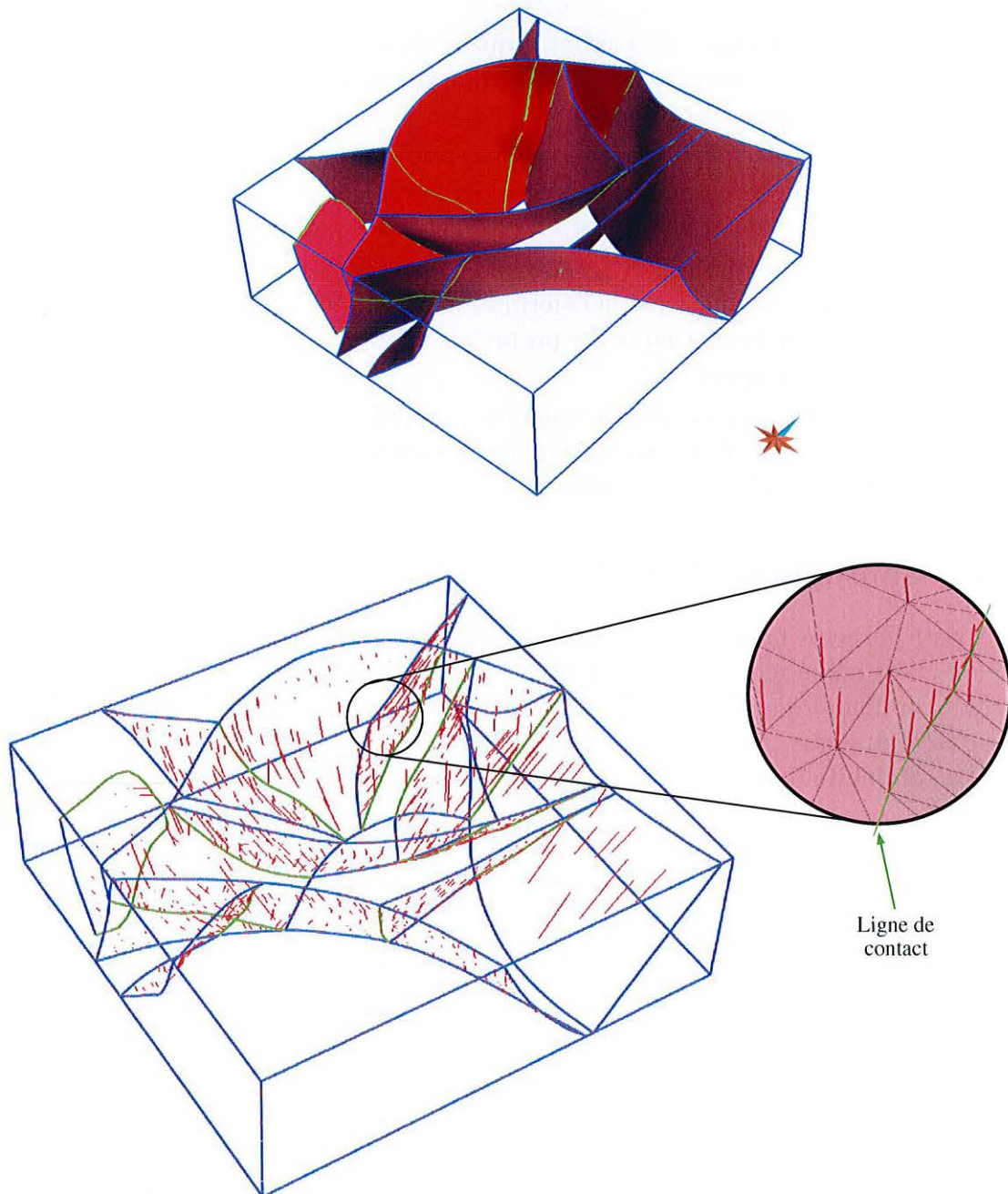
FIG. 4.12 : Exemple d'un modèle surfacique représentant un réseau de failles avec le Soft Frame Model associé (en haut) et vecteurs rejet calculés en 3D (en bas). Le détail permet de vérifier la présence d'un vecteur rejet à chaque nœud de la surface de faille. Le long de la ligne de contact entre failles (en vert), plusieurs rejets sont calculés sur chaque partie de faille touchant cette ligne. Les rejets sont ici indépendants de tout horizon.
