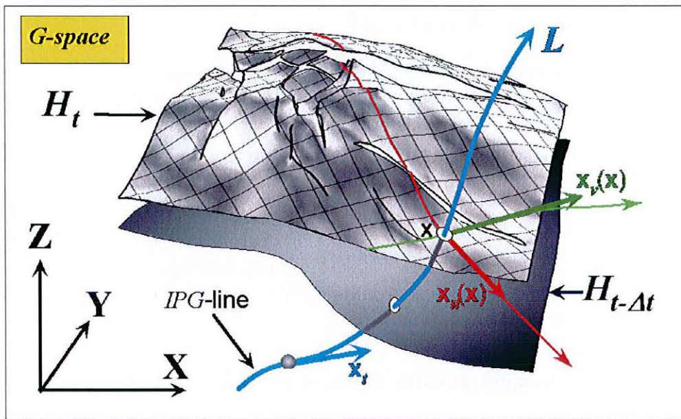
FIG. 2.9 : Intégration d'un horizon de référence et d'une ligne IPG dans la construction d'un modèle GeoChron. Quelle que soit la méthode de construction, les valeurs de t doivent être constantes sur chaque horizon et les valeurs de (u, v) doivent être constantes le long d'une ligne IPG ([Mallet, 2004]).
