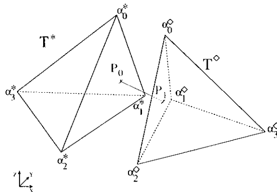
FIG. 4.13 : Notations utilisées pour décrire un vecteur rejet reliant deux points P_0 et P_1 situés dans deux tétraèdres T^* et T^\diamond de part et d'autre d'une faille.
