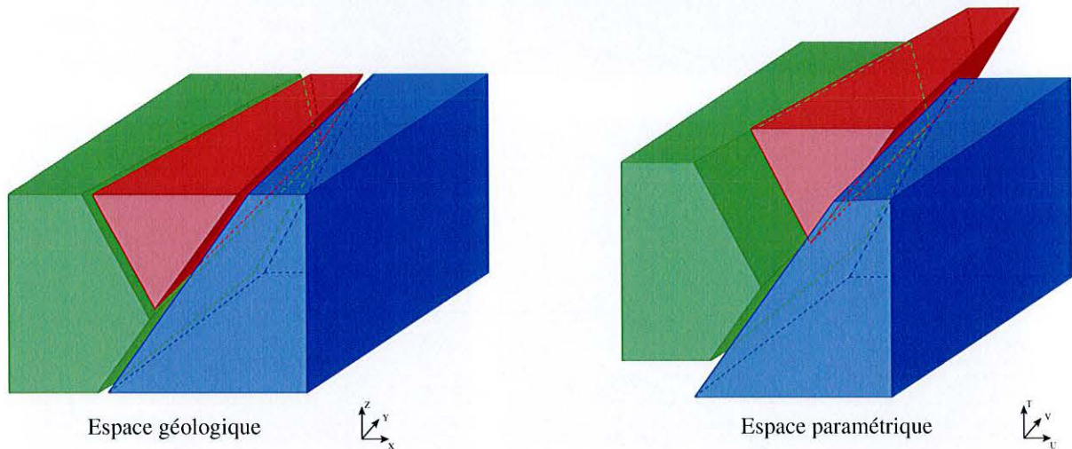
FIG. 4.20 : Vue en coupe d'une faille en Y. À gauche, dans l'espace géologique, les traits de couleur figurent des isovaleurs du temps c'est-à-dire des horizons. À droite, la même coupe vue dans l'espace paramétrique en supposant que l'on est dans un plan d'isovaleur de u ou de v . L'apparition de vides indique que cette hypothèse est fautive. Une explication possible, en trois dimensions, est fournie dans la figure 4.21.
