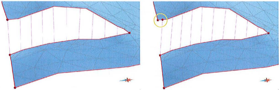
FIG. 4.3 : Installation de rejets sur une surface, le long d'une faille coupant le bord du domaine d'étude. À gauche, les lèvres de faille sont associées suivant leur paramétrisation 1D, les rejets sont erronés car les deux extrémités de bordure de gauche correspondent au bord du modèle et n'ont aucune réalité géologique. À droite, les lèvres sont associées suivant la distance curvilinéaire depuis l'extrémité de bordure interne, les rejets ne vont plus jusqu'au bord du modèle mais sont corrects.
