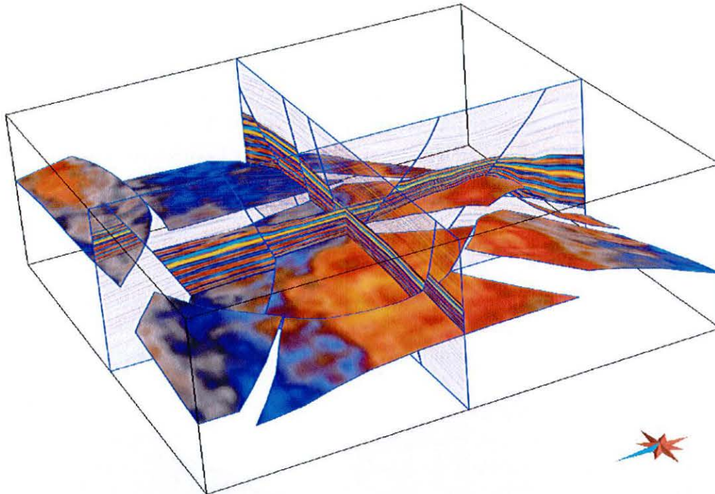
FIG. 5.18 : Visualisation de l'amplitude sismique correspondant à une couche géologique particulière. L'existence de la paramétrisation permet de définir une couche géologique dans l'espace \bar{G} entre deux surfaces d'isovaleur du paramètre t . Un masque de transparence est alors appliqué à tous les terrains en dehors de cette couche qui apparaît clairement dans l'espace géologique (d'après les travaux de T. Frank, [Frank, 2005]).
