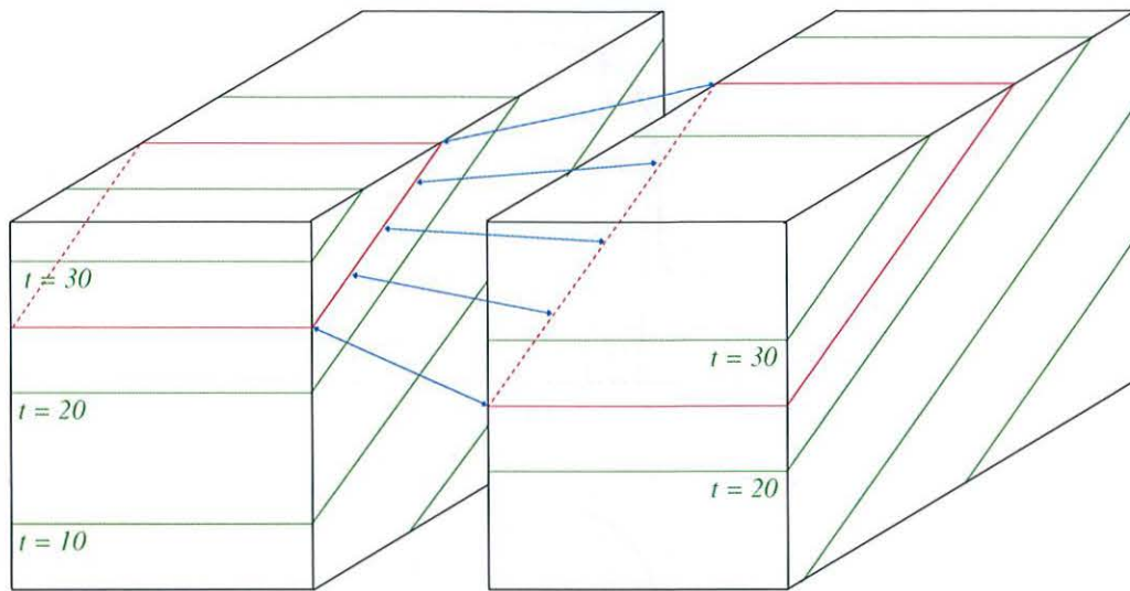
FIG. 4.10 : L'association automatique des bords logiques peut parfois conduire à des incohérences sur les bords du modèle. Ici, les deux bords de la surface d'isovaleur rouge t = 25 ont des longueurs très différentes à cause de leur intersection avec les limites du modèle mais ils coupent les mêmes arêtes du volume : ils sont donc abusivement associés.
