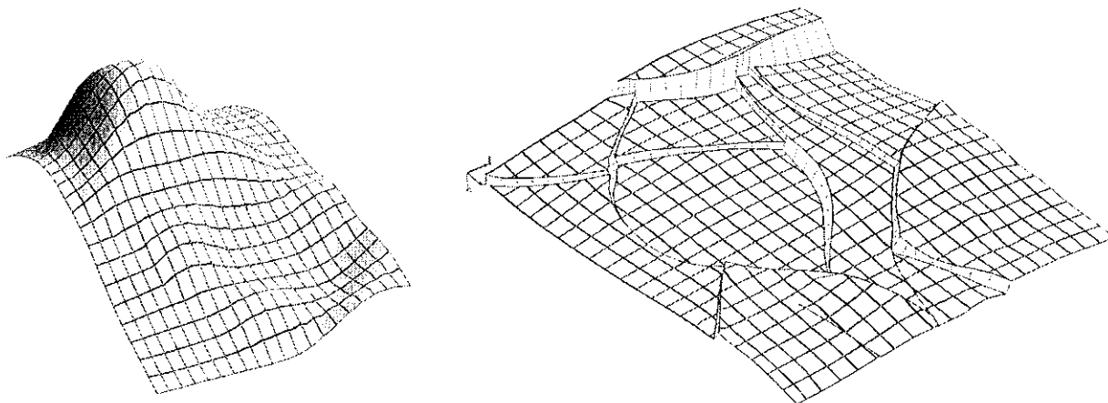
FIG. 3.3 : Paramétrisation 2D par conformal mapping de surfaces triangulées. La paramétrisation est figurée par les lignes d'isovaleurs de u (en rouge) et de v (en vert). À gauche, exemple d'une surface fortement plissée, noter les distorsions des lignes dans les zones non dépliables et de forte courbure. À droite, exemple d'une surface faillée, la paramétrisation est mise en cohérence entre les différents blocs grâce aux liens vectoriels (traits oranges, voir chapitre 4 pour plus de détails).
