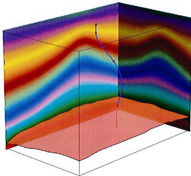
FIG. 3.13 : Ligne IPG (en bleu) extraite dans un volume paramétrisé depuis un horizon donné. Le paramètre temps est affiché sur le volume correspondant au modèle de la figure 3.11. Les points rouges le long de la ligne IPG représentent les intersections avec les horizons qui ont servi à construire le modèle, dont un seul est représenté ici (en transparence).
