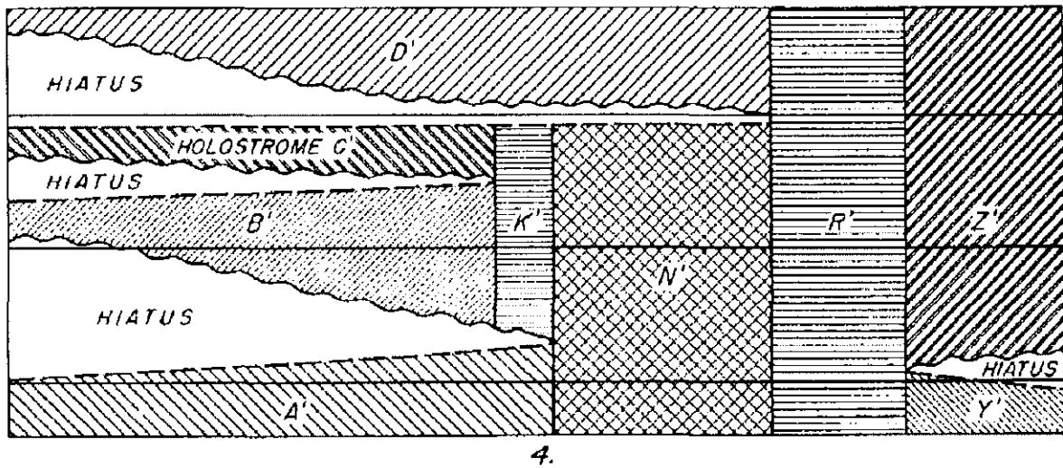
FIG. 2.8 : Diagramme de time stratigraphy ou de Wheeler ([Wheeler, 1958]). En haut, coupe simplifiée entre le Pacifique et les Montagnes Rocheuses, au 40 ème parallèle, montrant les principales séquences et inconformités (base du Mississippien supérieur et limite Trias-Jurassique). Au milieu, diagramme de time stratigraphy de la formation C, illustrant les principales composantes d'un diagramme de Wheeler. En bas, diagramme de Wheeler complet correspondant à la coupe, l'axe vertical du diagramme correspond à l'âge de dépôt des terrains et les différentes surfaces remarquables sont représentées sous forme de lignes horizontales, à temps constant. Noter la présence de zones de non dépôt (hiatus).
