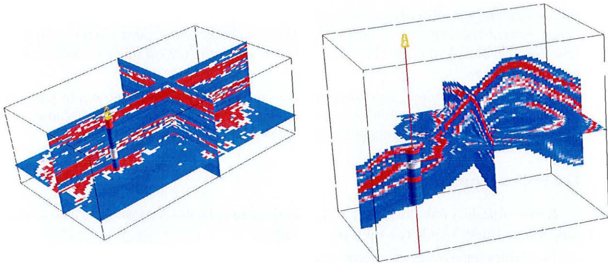
FIG. 3.5 : Visualisation d'une simulation de propriété pétrophysique sur une grille structurée régulière de l'espace géologique. À gauche, une propriété a été simulée à partir des données de puits, dans l'espace paramétrique. À droite, cette propriété est peinte sur le modèle géologique, en respectant la paramétrisation (voir paragraphe 5.1 pour la méthode de transfert).
