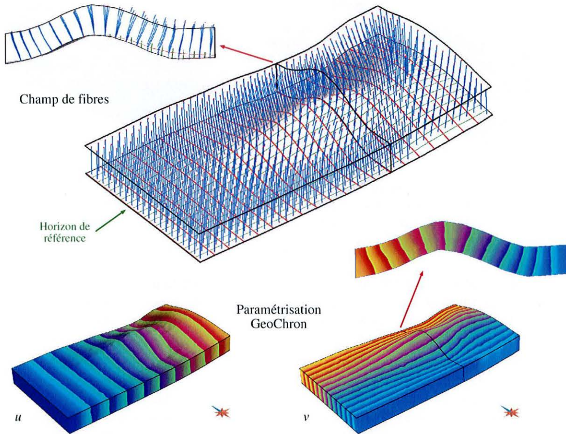
FIG. 3.19 : Paramétrisation du modèle de Split Mountain par la méthode des fibres (exagération verticale \times 2 ). En haut, champ de fibres extraites depuis l'horizon de référence. La coupe montre la courbure des fibres au centre du pli. En bas, paramétrisation GeoChron correspondante (seuls (u, v) sont représentés, t étant calculé indépendamment de la méthode de construction). La coupe dans la paramétrisation indique un style en pure bending (voir figure 3.20).
