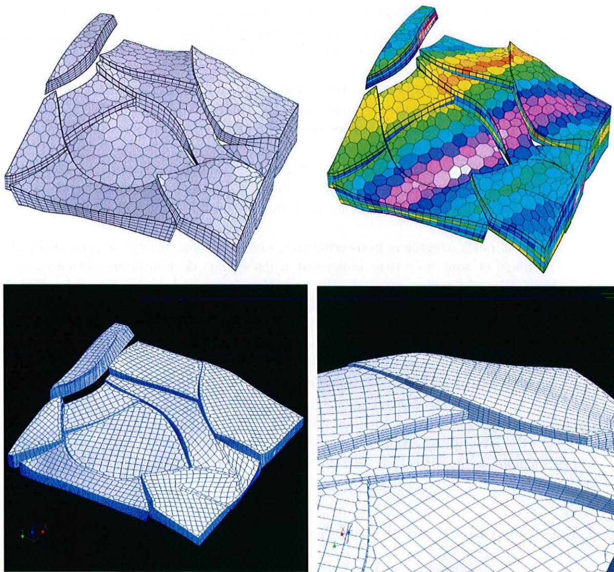
FIG. 1.2 : En haut, grille semi-structurée construite par extrusion régulière depuis une surface polygonale (à droite, la grille a été peinte avec une propriété définie dans chaque cellule). En bas, grille hybride, structurée au milieu des blocs et non-structurée au voisinage des failles ([Lepage, 2003], p. 187).
