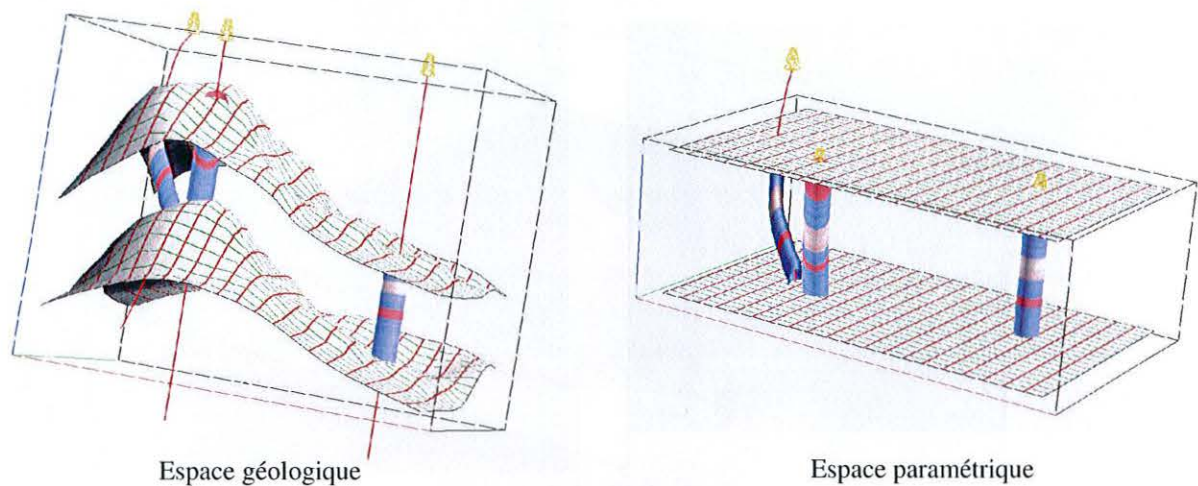
FIG. 5.1 : Transfert de données de l'espace géologique vers l'espace paramétrique. À gauche, trois puits traversant un modèle GeoChron défini dans le volume. Les deux horizons portent la trace du système de coordonnées paléo-géographiques (u, v) . À droite, les mêmes puits visualisés dans l'espace \bar{G} où les horizons sont mis à plat.
