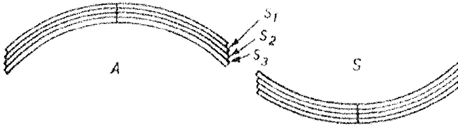
FIG. 2.12 : Déformation d'une couche par glissement banc sur banc (flexural slip), dans un anticlinal (A) et dans un synclinal voisin (S). Chaque sous-couche S_1, S_2, S_3 \dots garde sa longueur d'origine après déformation ([Hills, 1963], p. 222).
