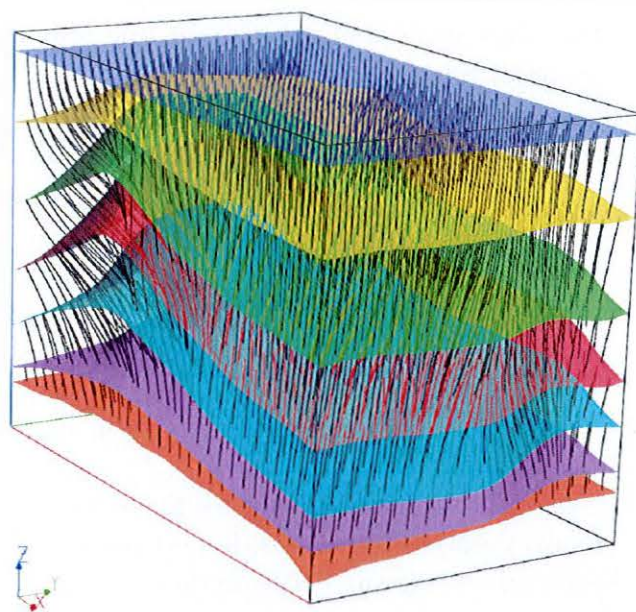
FIG. 3.11 : Contrôle de la densité du champ de fibres par réinitialisation de l'extraction sur chaque horizon. Depuis l'horizon de référence porteur de la paramétrisation 2D (en rouge, au milieu), des fibres sont extraites dans chaque direction jusqu'à l'horizon suivant. La paramétrisation (u, v) est alors interpolée sur cet horizon, avant d'en extraire un nouveau champ de fibres. Le volume est ainsi couvert par une densité de fibres constante (comparer avec la figure 3.8).
