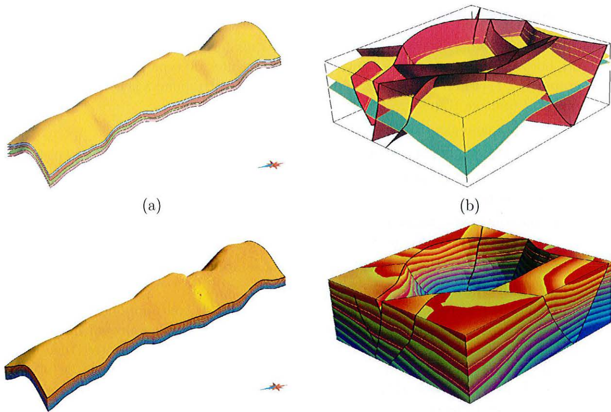
FIG. 3.1 : Exemples de construction de la composante t de la paramétrisation. En haut, le modèle surfacique, en bas, le temps calculé sur un volume tétraédrique. (a) : exemple non faillé (données Chevron). (b) : modèle faillé (données Total).
