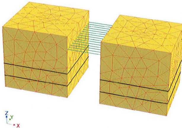
FIG. 4.16 : Modèle synthétique illustrant l'influence des rejets dans le calcul de la paramétrisation. Les deux cubes sont reliés par une série de vecteurs rejet (en vert). On impose des points de contrôle sur u et v sur la totalité des deux surfaces indiquées en noir. La paramétrisation initiale est telle que u = x , v = y et t = z .
