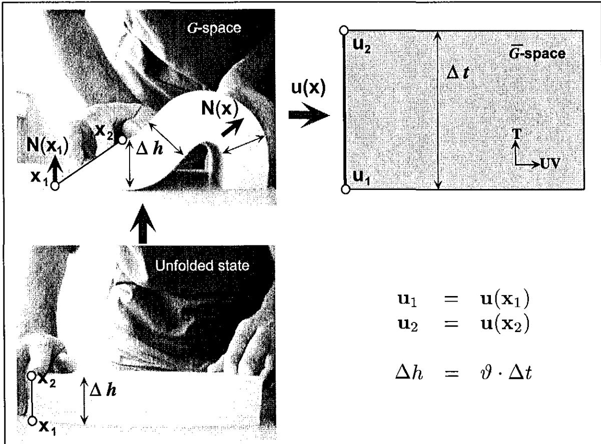
FIG. 2.7 : Un livre plié vu comme un analogue à la déformation d'une couche géologique, permettant d'établir la correspondance entre une couche réelle (en haut à gauche) et l'intervalle de temps correspondant dans l'espace paramétrique (en haut à droite). Le style de déformation est ici du flexural slip (voir plus loin), qui met en évidence la différence entre l'épaisseur réelle \Delta h de la couche, constante quel que soit l'état, et la longueur suivant une ligne- t reliant x_1 et x_2 . Ces deux longueurs sont les mêmes dans l'état déplié (en bas à gauche) ([Mallet, 2004]).
