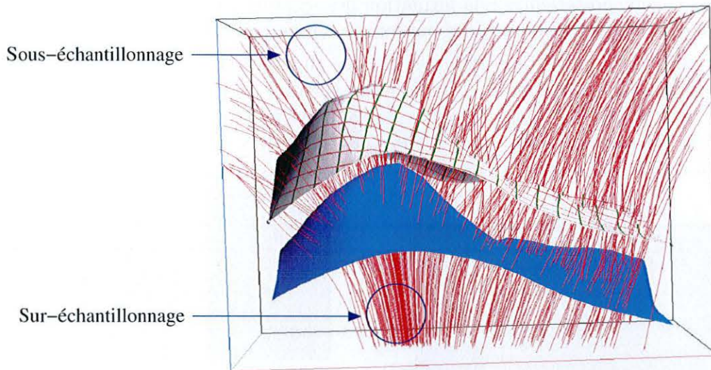
FIG. 3.8 : Champ de fibres extraites depuis un horizon de référence par la méthode de Runge-Kutta. Une paramétrisation par conformal mapping (représentée par les lignes d'iso-valeur de u et v rouges et vertes) est calculée sur l'horizon de référence (en haut) et sera propagée dans le volume le long des fibres. La densité des fibres est très variable suivant la position dans le volume et dépend de la courbure de l'horizon de référence.
