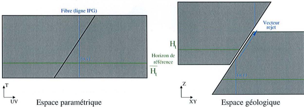
FIG. 3.9 : Principe de tracé des fibres au travers d'une faille. À gauche, une fibre (en bleu) extraite en un point (u, v) sur l'horizon de référence H_t ( \bar{H}_t ) dans l'espace paramétrique, en vert) apparaît dans l'espace paramétrique comme une ligne verticale, car c'est une ligne IPG. Son image dans l'espace géologique (à droite) est quant à elle décalée suivant le rejet de la faille.
