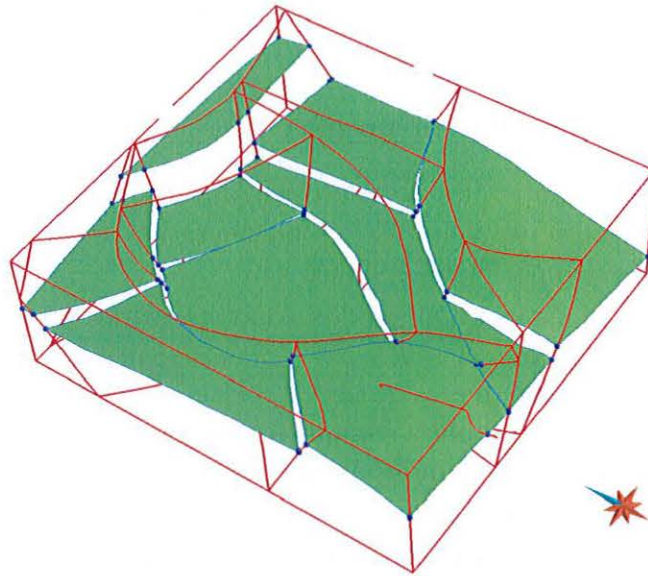
FIG. 4.7 : Surface d'isovaleur extraite depuis un volume tétraédrique et sur laquelle des extrémités de bordure (boules bleues) ont été installées automatiquement. Toutes les extrémités de bordure sont situées sur des arêtes du modèle (en rouge) et les extrémités situées sur la même arête sont associées.
