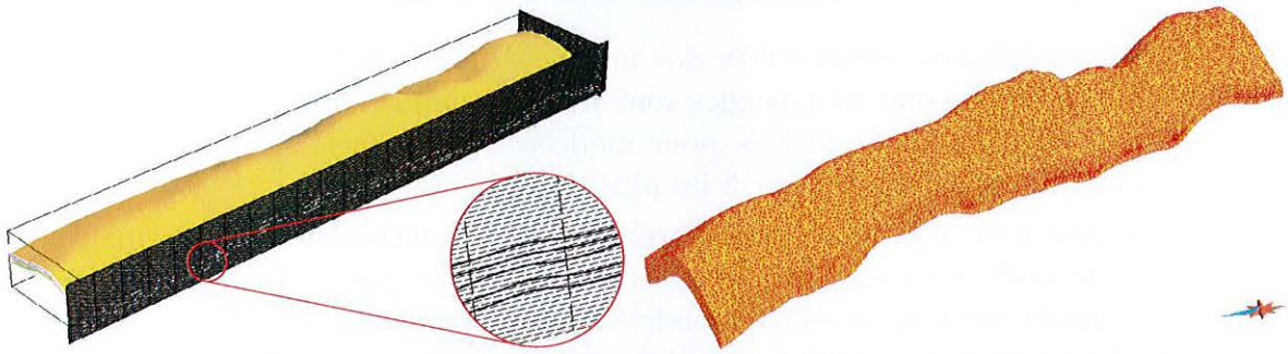
FIG. 3.6 : Modèle surfacique englobé dans un maillage structuré régulier (un « Voxet », à gauche) et dans un maillage tétraédrique non structuré (à droite). Pour garder un faible nombre de cellules au total (ici, de l'ordre de 10 000), les cellules de la grille régulière sont d'amplitudes très différentes verticalement et horizontalement, comme le montre le détail du cercle rouge, ce qui induit des erreurs de calcul. Un modèle aussi fin dans toutes les directions aurait de l'ordre du million de cellules. En comparaison, le modèle tétraédrique permet d'obtenir la même résolution, en se limitant au strict volume d'intérêt, avec environ 12 000 tétraèdres (données Chevron).
