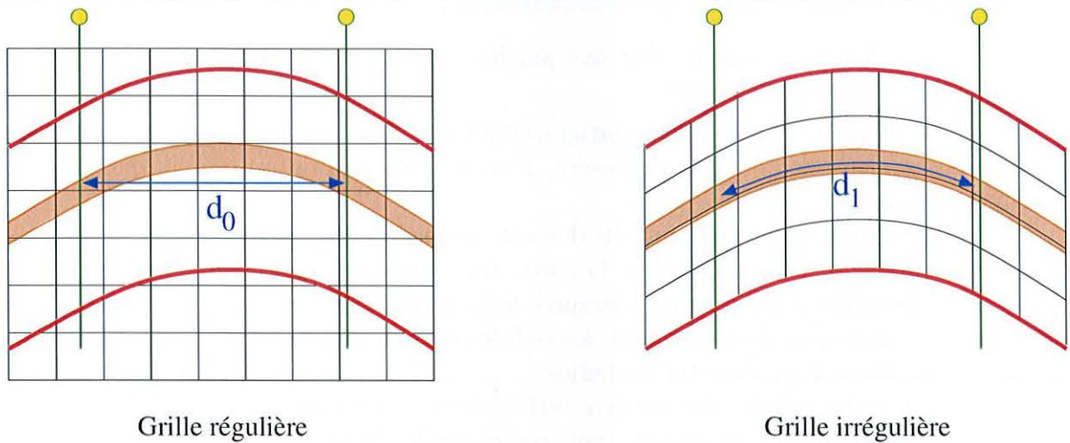
FIG. 1.7 : Longueur d'une couche (en marron) mesurée entre deux puits (en vert) dans une grille régulière (à gauche) et dans un grille irrégulière (à droite) adaptée à la stratigraphie définie par les horizons majeurs rouges. Les deux distances d_0 et d_1 sont calculées en suivant les maillages, mais d_1 est géologiquement plus réaliste pour modéliser des relations au sein de la couche.
