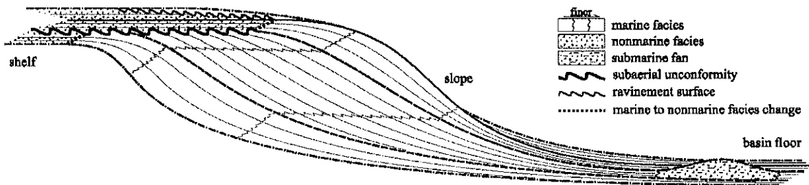
FIG. 2.2 : Variation latérale de faciès au sein d'une même couche le long d'une marge de bassin. Pendant la même durée, différents faciès (en nuances de gris) se sont déposés suivant la distalité, entre deux limites de séquences majeures. Les limites de faciès sont ici très différentes des surfaces isochrones (les limites de séquence). Noter aussi que l'épaisseur déposée varie fortement suivant les endroits au sein d'une même séquence ([Catuneanu et al., 1998]).
