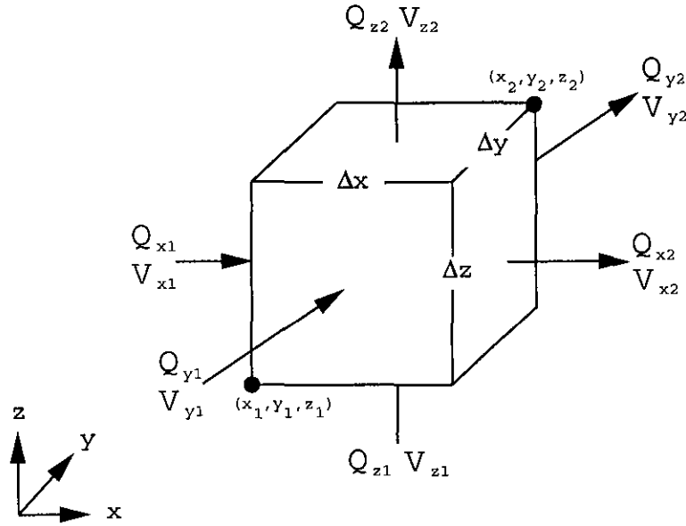
FIG. 3.7 : Notations utilisées dans le cadre de la méthode de tracé de particules de Pollock. Les Q_{x_1} \dots se réfèrent au débit au travers des faces ([Voillemont, 2001], p. 36).
