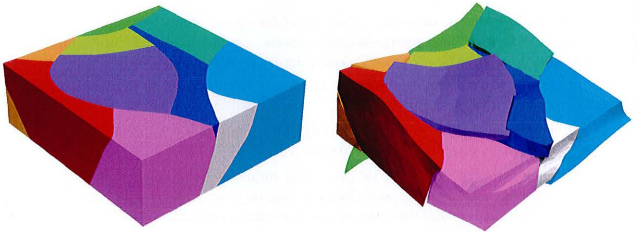
FIG. 4.15 : Visualisation d'un volume tétraédrisé dans l'espace paramétrique. À gauche, le volume dans l'espace géologique, à droite, le même volume déplacé dans l'espace paramétrique (chaque couleur indique un bloc de faille). Ici, comme aucun vecteur rejet n'a encore été appliqué, les blocs se recouvrent ou laissent des vides dans l'espace paramétrique.
