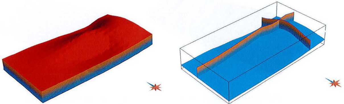
FIG. 3.15 : Calcul du paramètre t sur le modèle de Split Mountain, Utah (exagération verticale \times 2 ). Un temps constant a été affecté à chacun des horizons de la figure 3.14. À gauche, le volume tétraédrique peint avec le temps, à droite, deux coupes verticales dans le modèle et une surface d'isovaleur de t mettant en évidence la courbure du modèle.
