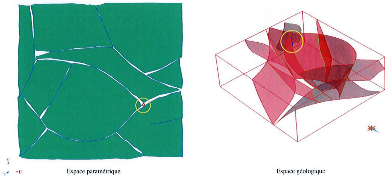
FIG. 4.19 : Désignation manuelle d'un rejet dans l'espace paramétrique. À gauche, vue en plan d'une section du volume tétraédrisé dans l'espace paramétrique. Trois rejets (traits rouges) sont ajoutés. À droite, ces rejets sont automatiquement reportés dans l'espace géologique. Comme ils sont situés à la jonction de deux failles, les trois rejets sont confondus et sont sur la ligne d'intersection de ces deux failles.
