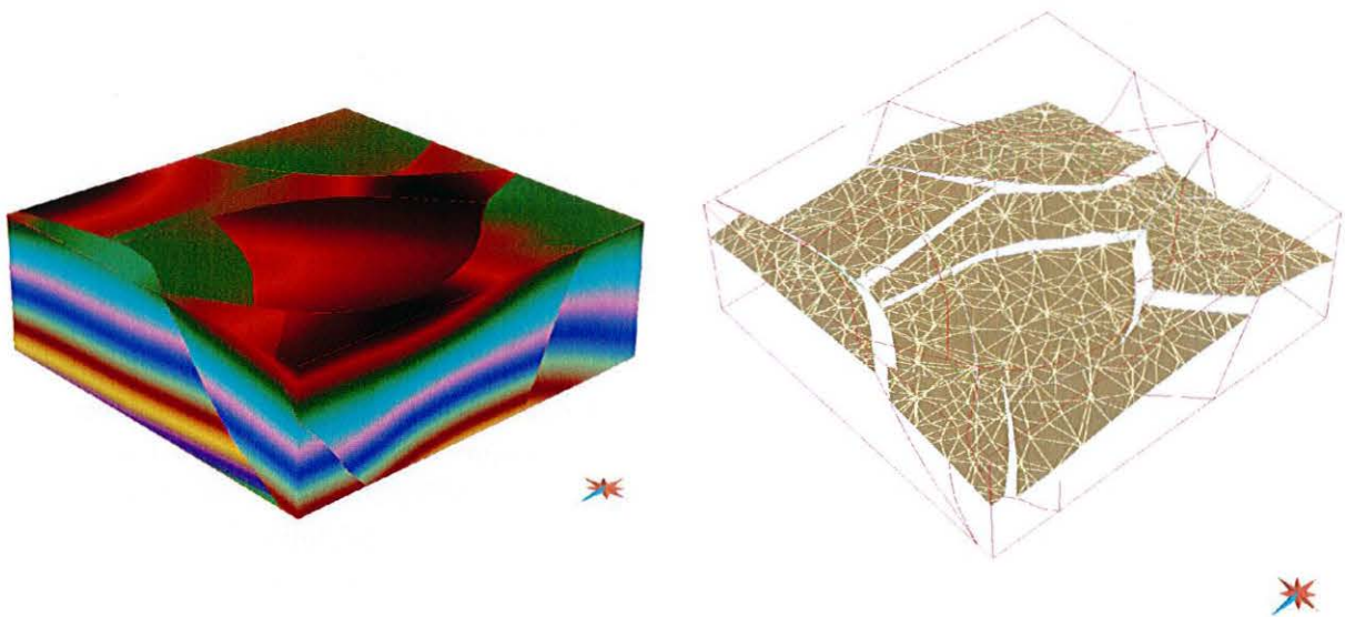
FIG. 4.6 : Extraction d'une surface d'isovaleur. À gauche, volume tétraédrique peint avec la propriété temps définie aux nœuds; à droite, surface d'isovaleur triangulée extraite de ce volume (les lignes rouges figurent les lignes radiales du Soft Frame Model c'est-à-dire les traces des failles dans le modèle).
