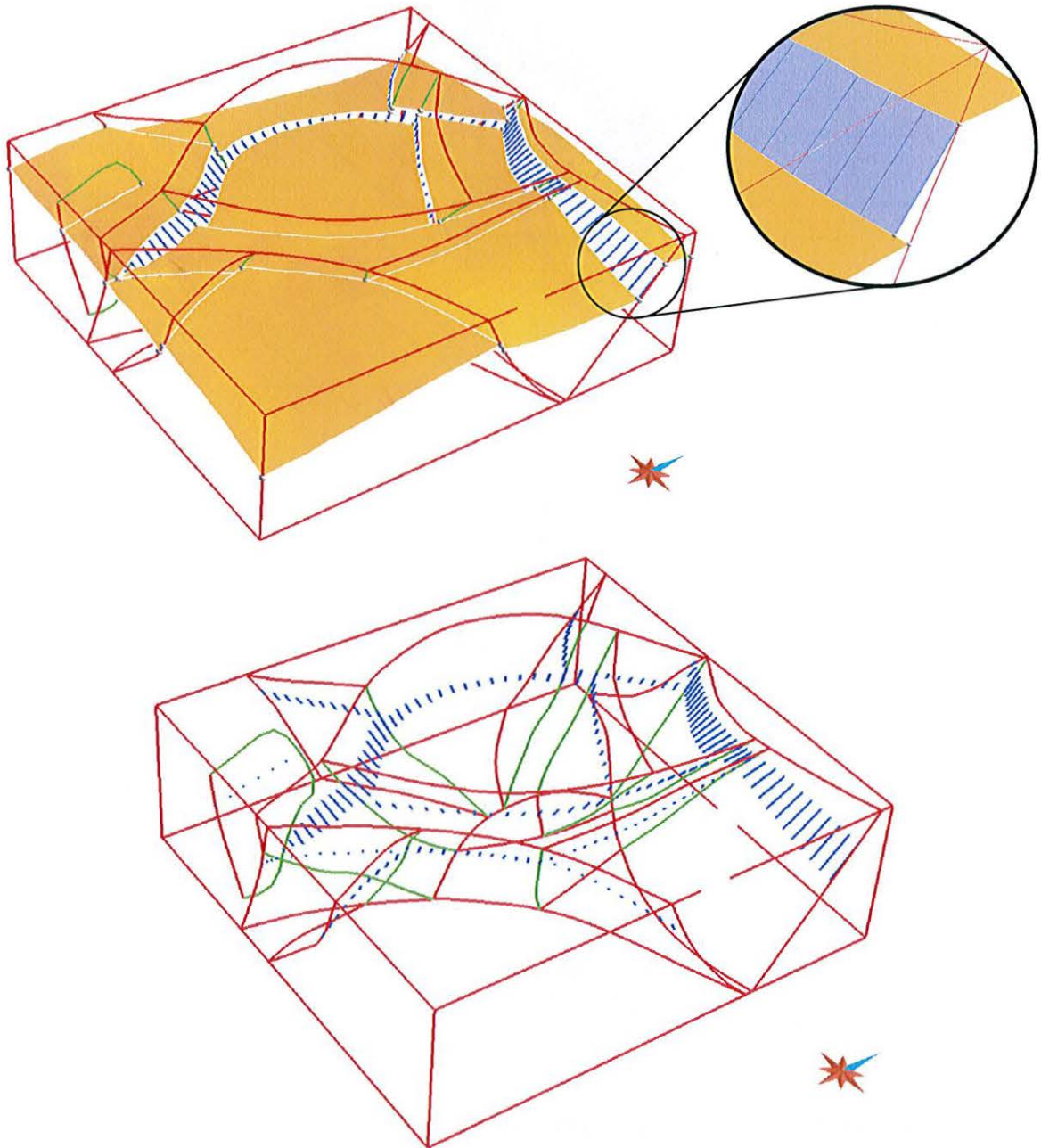
FIG. 4.8 : En haut, calcul des rejets sur une surface d'isovaleur et, en bas, copie de ces rejets dans le volume tétraédrisé. Noter que, pour les lèvres de faille qui touchent le bord du modèle (dans le cercle, par exemple), l'appariement s'est fait suivant la distance curvilinéaire le long de la lèvre et non pas suivant la paramétrisation 1D des deux lèvres.
