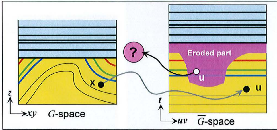
FIG. 2.4 : Coupe verticale illustrant la correspondance entre G et \overline{G} , en présence de zones d'érosion. Certains points de l'espace paramétrique n'ont pas de correspondance dans l'espace géologique initial ([Mallet, 2004]).
