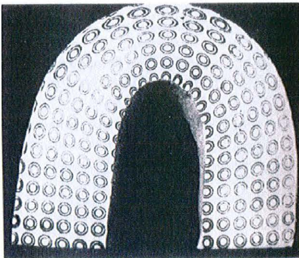
FIG. 2.10 : Déformation d'une couche par flexure simple (pure bending) d'une plaque homogène. À gauche, coupe dans un analogue d'un pli, illustrant la différence de déformation suivant la position dans le pli. À droite, vue en trois dimensions d'un pli réel. Noter la forme en « selle de cheval » le long de l'axe du pli ([Hills, 1963], pp. 86 et 222).
