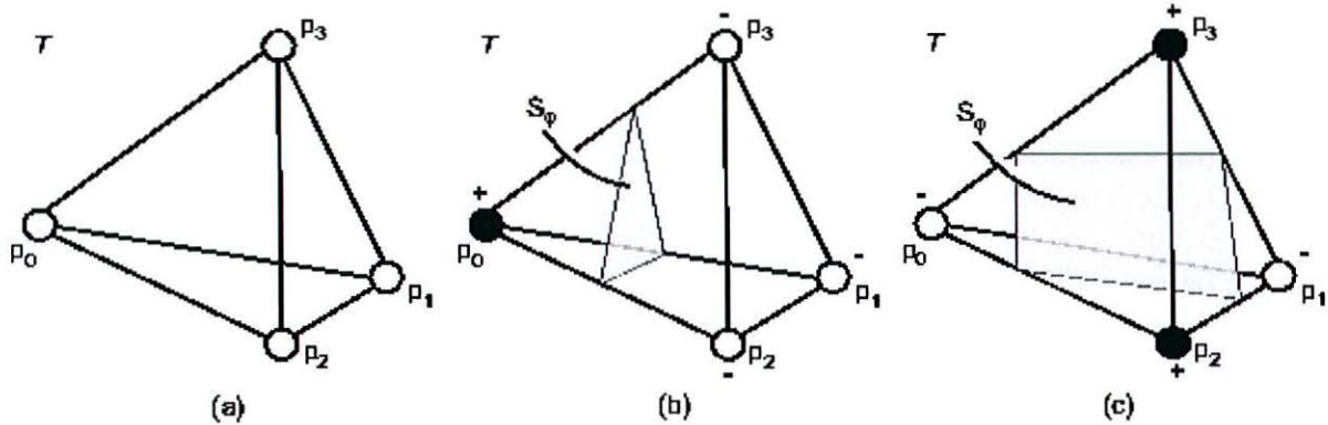
FIG. 4.5 : Tétraèdre T traversé par une surface d'isovaleur S_{\varphi_0} d'une propriété \varphi définie aux nœuds de ce tétraèdre ([Frank, 2004]). (a) Les valeurs de \varphi aux nœuds de T sont soit toutes supérieures à \varphi_0 , soit inférieures, \{S_{\varphi} \cap T\} = \emptyset . (b) Un des nœuds a une valeur de \varphi supérieure à \varphi_0 , les trois autres ont des valeurs inférieures (ou le contraire), \{S_{\varphi} \cap T\} est composé d'un seul triangle. (c) Deux nœuds ont des valeurs supérieures à \varphi_0 , deux ont des valeurs inférieures, \{S_{\varphi} \cap T\} contient deux triangles.
