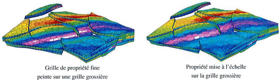
FIG. 5.9 : Exemple d’upsampling d’une propriété sur une grille polyédrique. À gauche, une simulation stochastique de propriété réalisée sur une grille fine dans l’espace paramétrique est peinte sur une grille polyédrique adaptée aux écoulements, dans l’espace géologique. À droite, la propriété a été mise à l’échelle (par une simple moyenne arithmétique) de la grille grossière (d’après [Grosse, 2002]).
