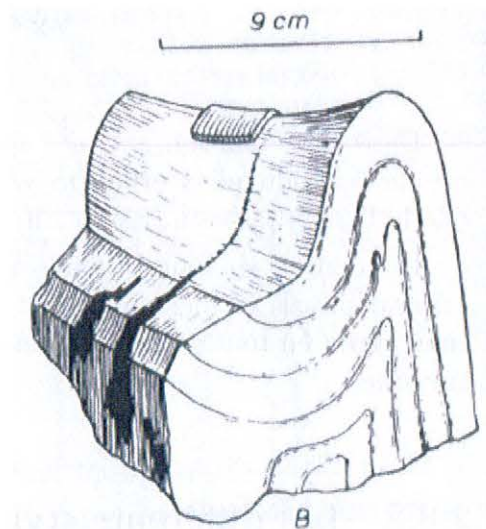
FIG. 2.10 : Déformation d'une couche par flexure simple (pure bending) d'une plaque homogène. À gauche, coupe dans un analogue d'un pli, illustrant la différence de déformation suivant la position dans le pli. À droite, vue en trois dimensions d'un pli réel. Noter la forme en « selle de cheval » le long de l'axe du pli ([Hills, 1963], pp. 86 et 222).
