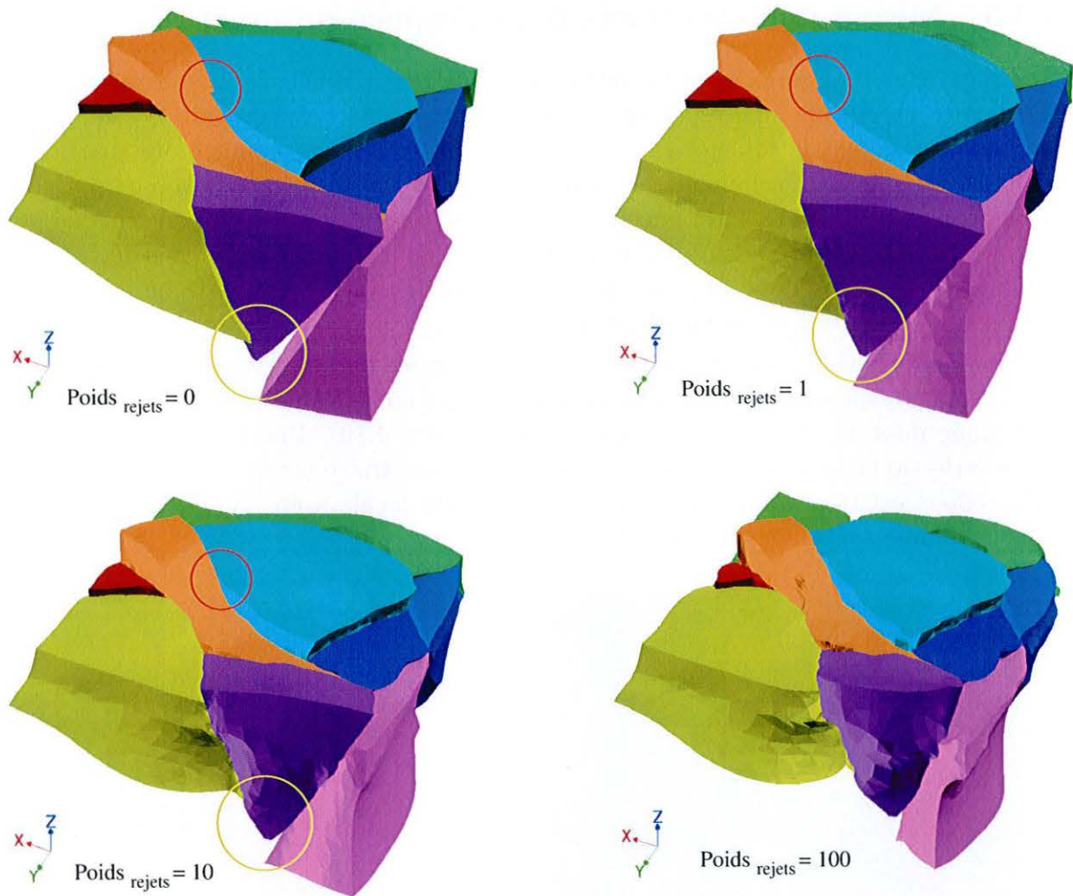
FIG. 4.18 : Influence du poids de la contrainte de continuité sur la paramétrisation (volumes affichés dans l'espace paramétrique). En haut à gauche, aucune contrainte de continuité n'est imposée. Les blocs ne sont pas en cohérence, certains se recouvrent (cercle rouge) et d'autres sont trop écartés (cercle jaune). En haut à droite, la contrainte de continuité est utilisée avec un poids égal à celui des autres contraintes. Dans le cercle jaune, les blocs sont presque en cohérence mais le recouvrement du cercle rouge est toujours présent. En bas à gauche, avec un poids relatif de 10, le recouvrement du cercle rouge est corrigé mais des effets de contraction du modèle commencent à apparaître. Enfin, en bas à droite, avec un poids relatif de 100, les contacts sont tous respectés mais le modèle est abusivement contracté autour des failles.
