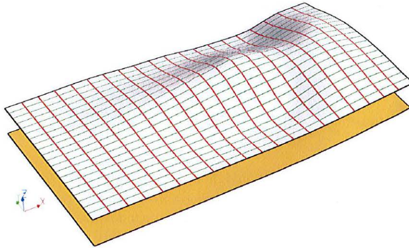
FIG. 3.16 : Paramétrisation de l'horizon de référence du modèle de Split Mountain, Utah. Les lignes rouges et vertes figurent des isovalues de u et v (exagération verticale \times 2 ).
