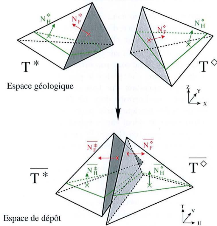
FIG. 4.14 : Deux tétraèdres de part et d'autre d'une faille, reliés par un vecteur rejet, à leur position géologique actuelle (en haut) et dans leur position au moment du dépôt (en bas). Les surfaces d'isovaleur du temps (en vert) sont alors toutes les deux horizontales et les faces communes (en grisé) sont en contact.
