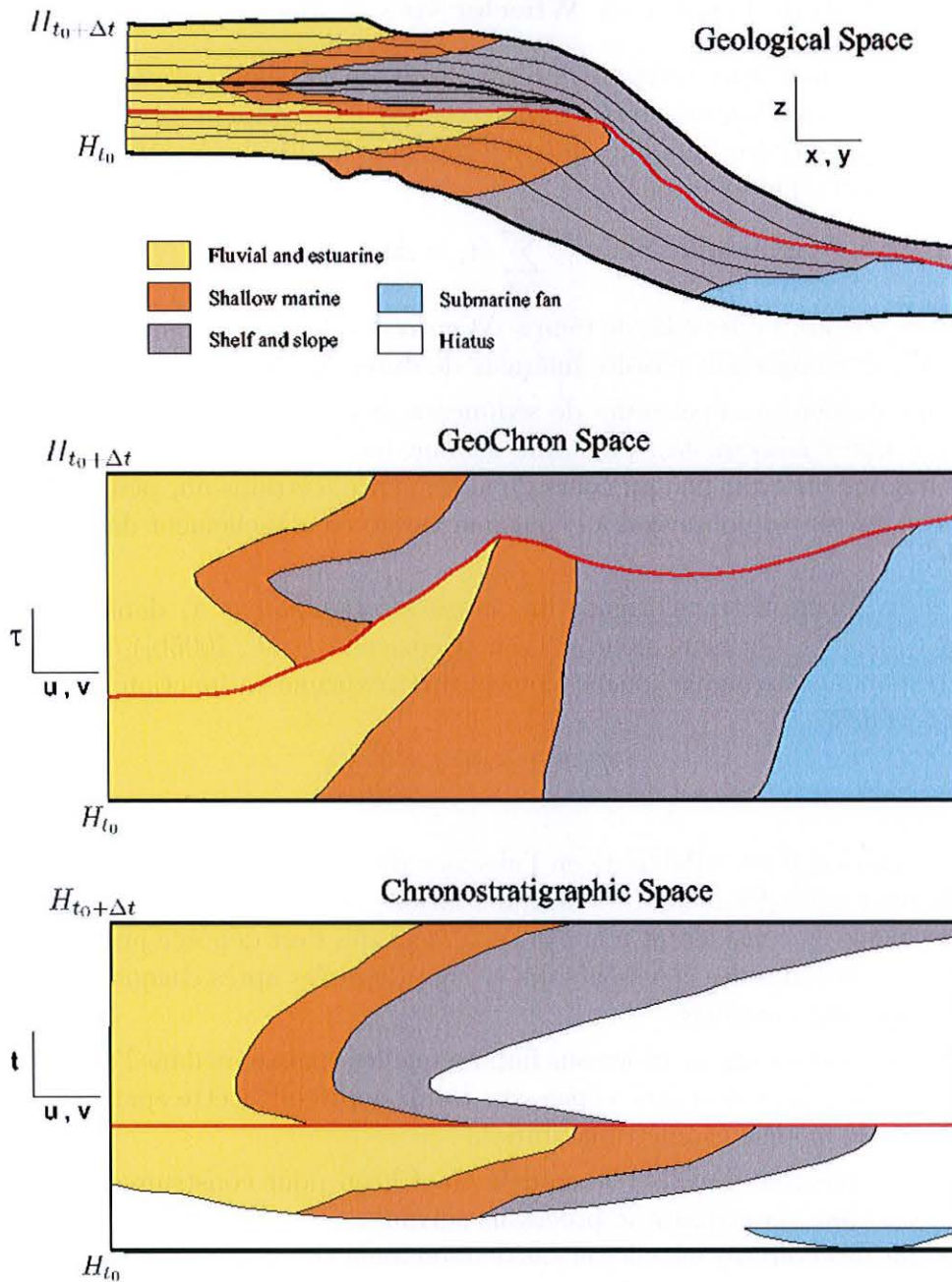
FIG. 5.7 : Correspondance entre l'espace géologique (en haut), l'espace paramétrique \bar{G} (au milieu) et l'espace de Wheeler (en bas) construits à partir des deux surfaces limitant une séquence majeure. L'isochrone intermédiaire (en rouge) est transformée en une ligne horizontale dans l'espace de Wheeler, mais pas dans l'espace paramétrique. Noter la présence de vides dans l'espace de Wheeler qui sont absents dans l'espace paramétrique. On vérifie aussi ici l'importance de choisir des surfaces isochrones et non pas des limites de faciès pour construire la paramétrisation GeoChron ([Kedzierski et al., 2005b]).
