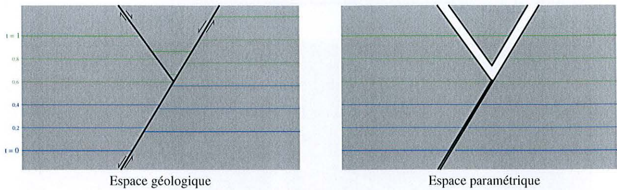
FIG. 4.20 : Vue en coupe d'une faille en Y. À gauche, dans l'espace géologique, les traits de couleur figurent des isovaleurs du temps c'est-à-dire des horizons. À droite, la même coupe vue dans l'espace paramétrique en supposant que l'on est dans un plan d'isovaleur de u ou de v . L'apparition de vides indique que cette hypothèse est fautive. Une explication possible, en trois dimensions, est fournie dans la figure 4.21.
