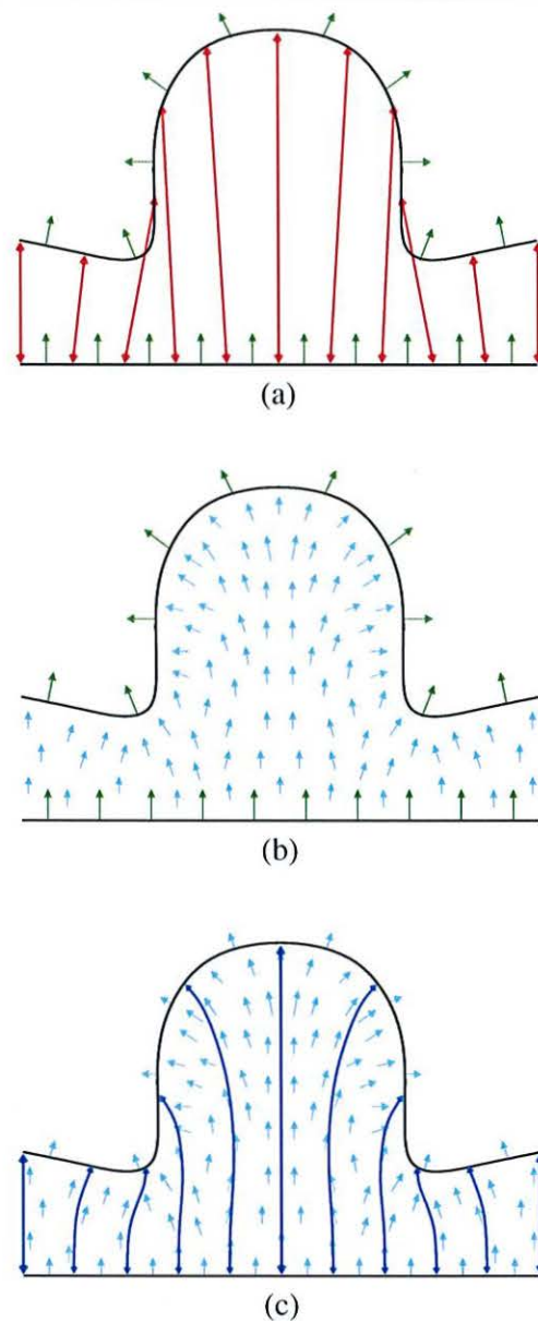
FIG. 4.11 : Vue en coupe de deux lèvres de faille. (a) Les rejets calculés en utilisant la paramétrisation 1D des lèvres de faille peuvent croiser les horizons. (b) Champ de vecteurs interpolé entre les deux lèvres à partir de la normale à ces lèvres en tout point. (c) Trajectoire des rejets extraits en suivant le champ de vecteurs.
