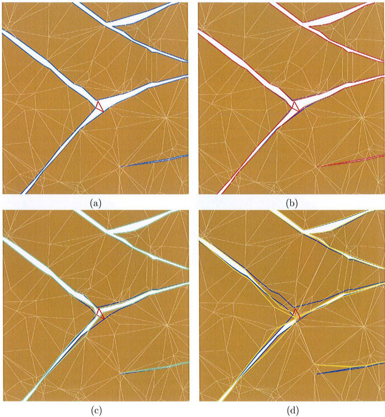
FIG. 4.22 : Section horizontale (vue en plan) dans l'espace paramétrique. (a) Section initiale. Des rejets (en rouge) sont ajoutés manuellement. Les bords de la section initiale (en bleu) sont toujours laissés pour comparaison. (b) Réinterpolation de u et de v en affectant le même poids à la contrainte de continuité liée aux nouveaux rejets qu'aux autres contraintes. Les bords de la nouvelle section sont en rouge. (c) Réinterpolation de u et de v avec un poids relatif de 10, les bords sont en vert. (d) Réinterpolation de u et de v avec un poids relatif de 100, les bords sont en jaune.
