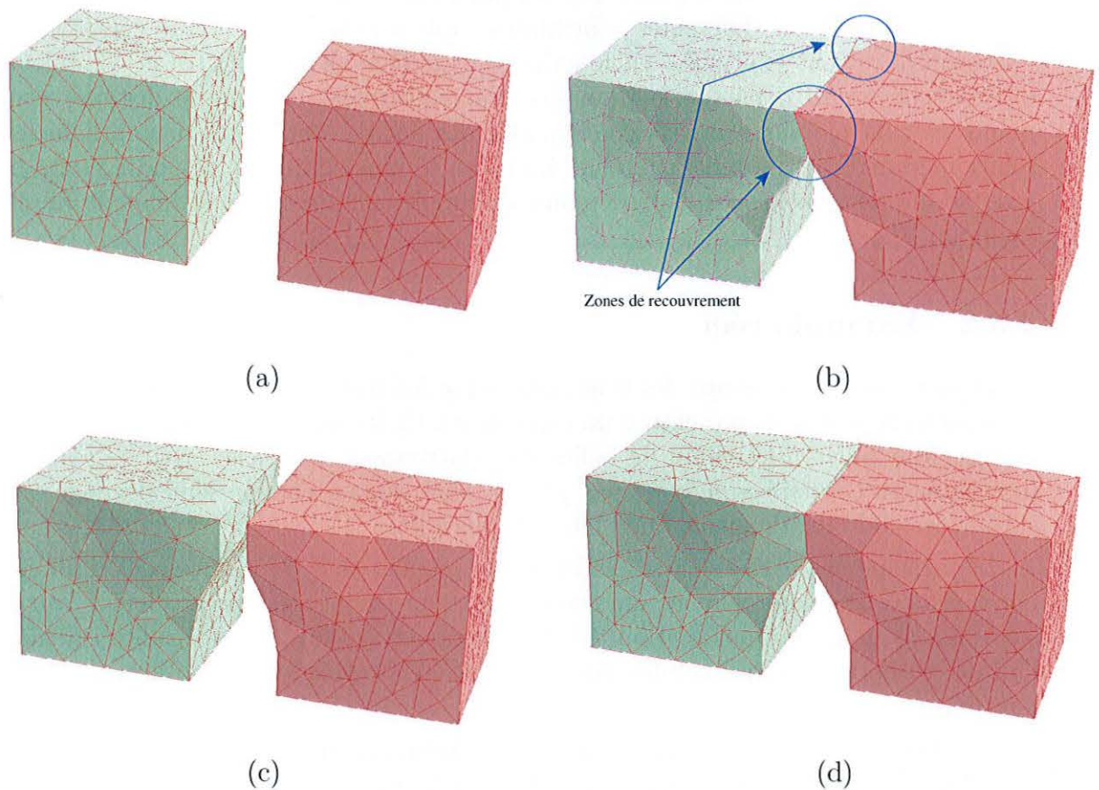
FIG. 4.17 : Le modèle synthétique dans l'espace paramétrique (u, v, t) après interpolation de u et de v . (a) Sans aucune contrainte liée aux rejets; (b) la contrainte de continuité C_0 est ajoutée, noter le recouvrement entre les deux blocs; (c) avec la contrainte de continuité C_1 , les tétraèdres de part et d'autre prennent la même orientation; (d) lorsqu'on augmente le poids de la contrainte de continuité, on obtient une correspondance parfaite.
