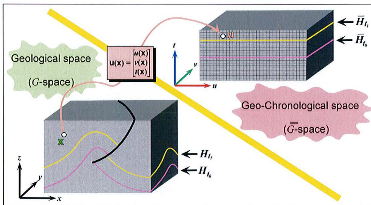
FIG. 2.1 : Schéma de principe de l'espace GeoChron. En bas, un modèle géologique G , avec des horizons H_{t_0} et H_{t_1} plissés et faillés. En haut, les images de ces horizons dans l'espace paramétrique \bar{G} sont des surfaces planes non faillées ([Mallet, 2004]).
