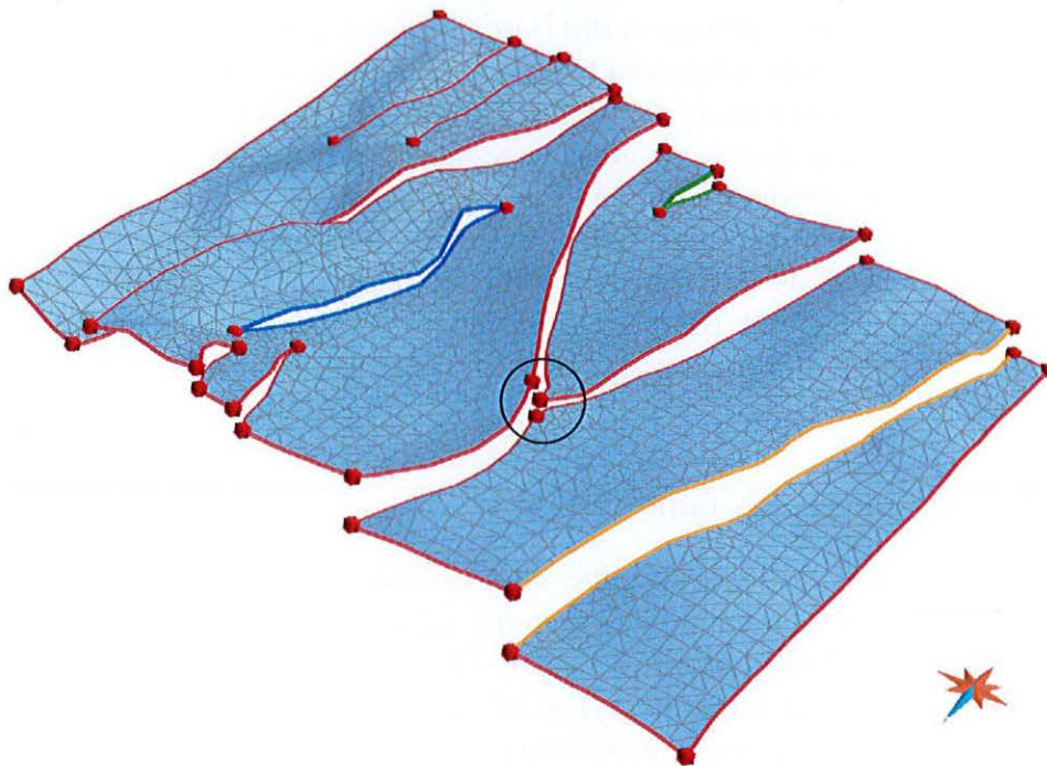
FIG. 4.2 : Modèle macro-topologique d'une surface triangulée. Les extrémités de bordure sont figurées par les boules rouges, les bords logiques par les traits de couleur. En bleu, deux bords logiques correspondant à une faille entièrement incluse dans le domaine d'étude, qui partagent les mêmes extrémités. En vert, une faille touchant une limite du domaine d'étude, avec deux extrémités sur cette limite. En orange, une faille touchant deux limites du domaine d'étude. Le cercle noir indique un endroit où il est nécessaire d'ajouter des extrémités de bordure au milieu des traces de failles, afin d'assurer la cohérence des bords logiques de part et d'autre de la faille.
