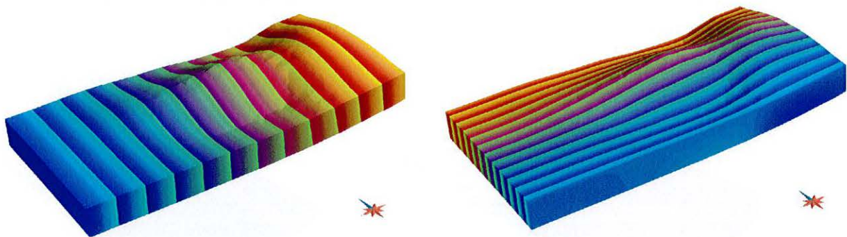
FIG. 3.17 : Paramétrisation (u, v) obtenue par la contrainte d'orthogonalité 3D (à gauche, u(\mathbf{x}) , à droite v(\mathbf{x}) ), exagération verticale \times 2 . Les lignes de couleur représentent des lignes d'isovalues. Ces lignes sont équidistantes sur l'horizon de référence (figure 3.16).
