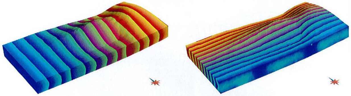
FIG. 3.18 : Paramétrisation (u, v) obtenue par la contrainte de conformal mapping étendu (à gauche, u(\mathbf{x}) , à droite v(\mathbf{x}) ), exagération verticale \times 2 . Les lignes de couleur représentent des lignes d'isovaleurs. Ces lignes sont équidistantes sur l'horizon de référence (figure 3.16).
