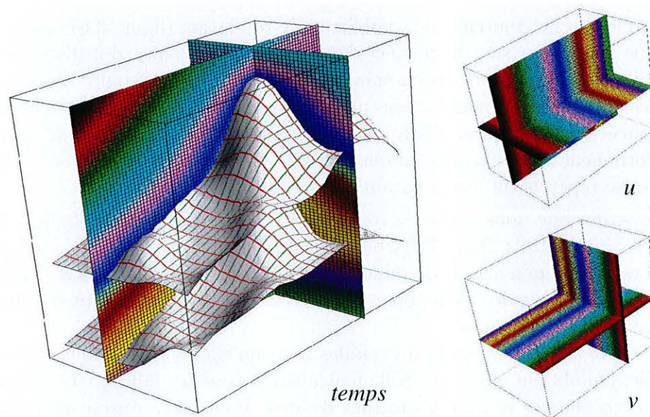
FIG. 3.4 : Paramétrisation GeoChron calculée sur une grille structurée régulière (« Voxet »). À gauche, les deux horizons initiaux, peints avec des lignes d'isovaleur de u et v ainsi que le paramètre t dans le volume ; à droite, les composantes u et v dans le volume. L'horizon du bas a été utilisé comme horizon de référence pour (u, v) .
