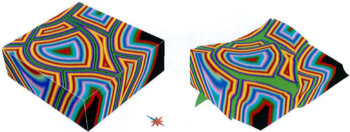
FIG. 5.3 : Carte de distance aux failles dans l'espace géologique (à gauche) correspondant au réseau de failles de la figure 1.6 et dans l'espace paramétrique (à droite). Une altération du cube de propriété pétrophysique de la figure 5.2 en fonction de cette carte de distance permet de prendre en compte l'influence des volumes de faille (d'après les travaux de T. Frank [Frank, 2005]).
