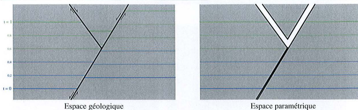
FIG. 4.20 : Vue en coupe d'une faille en Y. À gauche, dans l'espace géologique, les traits de couleur figurent des isovaleurs du temps c'est-à-dire des horizons. À droite, la même coupe vue dans l'espace paramétrique en supposant que l'on est dans un plan d'isovaleur de u ou de v . L'apparition de vides indique que cette hypothèse est fautive. Une explication possible, en trois dimensions, est fournie dans la figure 4.21.
