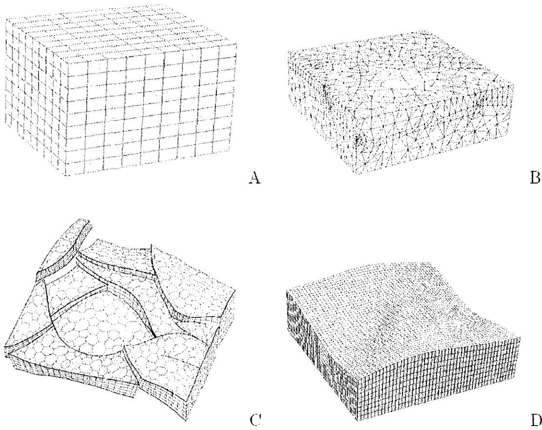
FIG. 1.3 : Exemples de différents types de maillages. A : maillage régulier structuré (« boîte à sucre »); B : maillage non structuré irrégulier à base de tétraèdres; C : maillage semi-structuré (formé par empilement structuré de couches non-structurées) irrégulier; D : maillage structuré irrégulier, à base d'hexaèdres (« grille stratigraphique ») ([Souche, 2005], p. 29).
