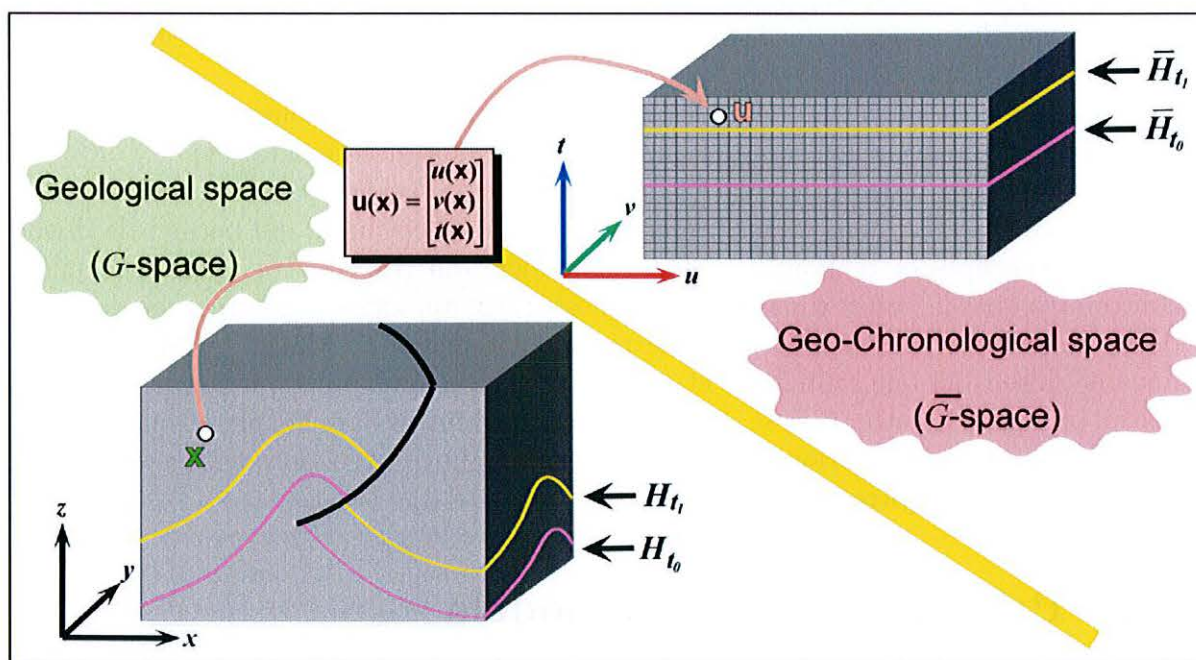
FIG. 2.1 : Schéma de principe de l'espace GeoChron. En bas, un modèle géologique G , avec des horizons H_{t_0} et H_{t_1} plissé et faillés. En haut, les images de ces horizons dans l'espace paramétrique \bar{G} sont des surfaces planes non faillées ([Mallet, 2004]).
