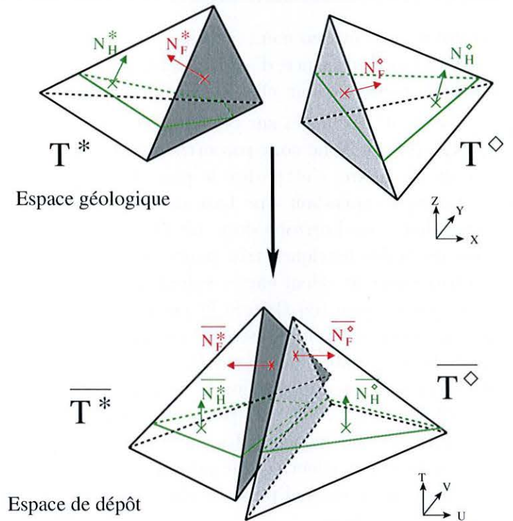
FIG. 4.14 : Deux tétraèdres de part et d'autre d'une faille, reliés par un vecteur rejet, à leur position géologique actuelle (en haut) et dans leur position au moment du dépôt (en bas). Les surfaces d'isovaleur du temps (en vert) sont alors toutes les deux horizontales et les faces communes (en grisé) sont en contact.
