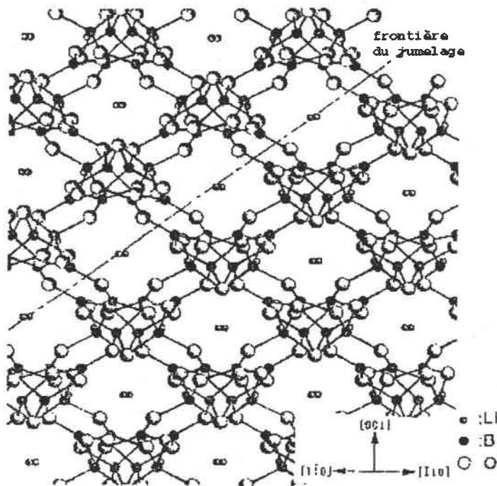
Figure 3 : projection le long de [110] montrant la frontière de jumelage [5].
