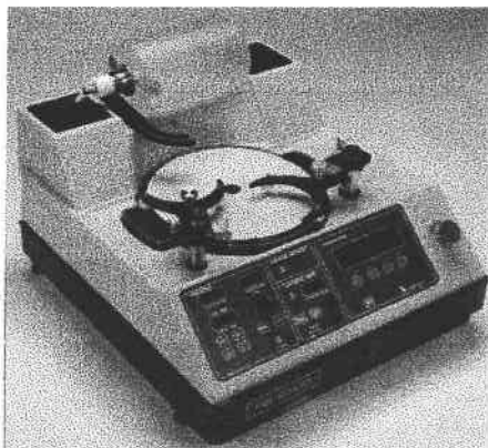
Figure 3 : à gauche : Logitech PM4, à droite : Piston.
