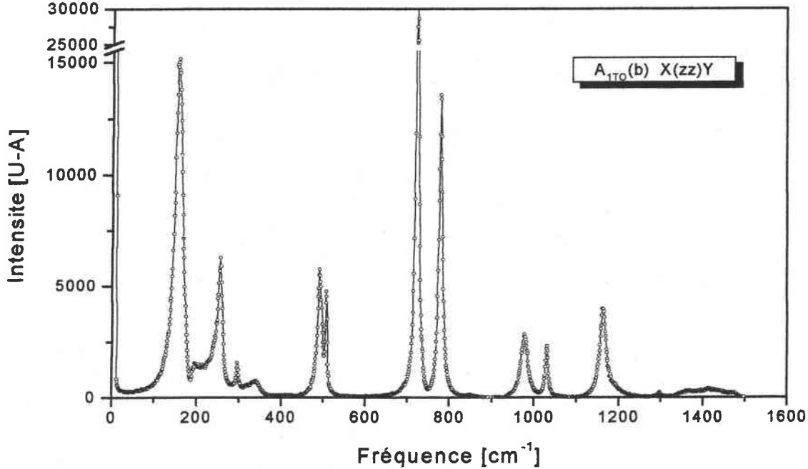
Figure C-9 : Le spectre des modes A_{1TO}(b) .
