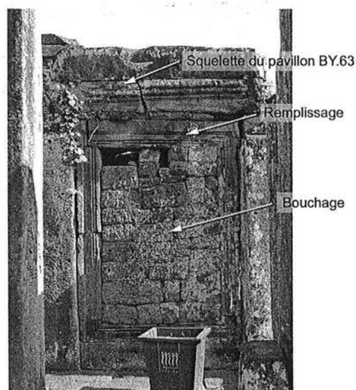
Ph. 34 : Exemple de remplissage périphérique au pavillon BY.63
