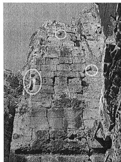
Ph. 75 : Face Est de la tour BY.11 présentant des logements de crampons
