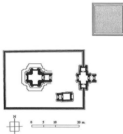
Fig. 10 : Plan générique des chapelles des hôpitaux de Jayavarman VII
