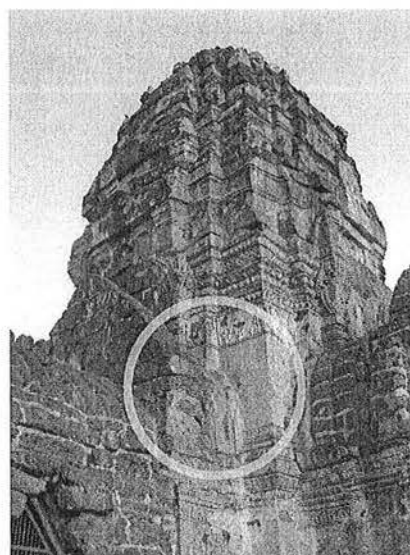
Ph. 32 : Exemple de superstructure présentant des traces d'enduit au Prang Sam Yod (Lopburi, Thaïlande)
