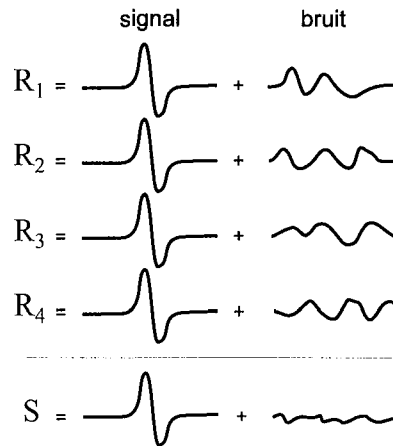
FIG. 2.31 – Principe de la sommation : le signal réfléchi au même point du sous-sol mais enregistré sur des récepteurs R_1, R_2, R_3, R_4 voisins passe par des chemins voisins mais différents dans le sous-sol. En sommant les signaux captés, les signaux cohérents s'additionnent tandis que les bruits aléatoires s'annulent mutuellement.
