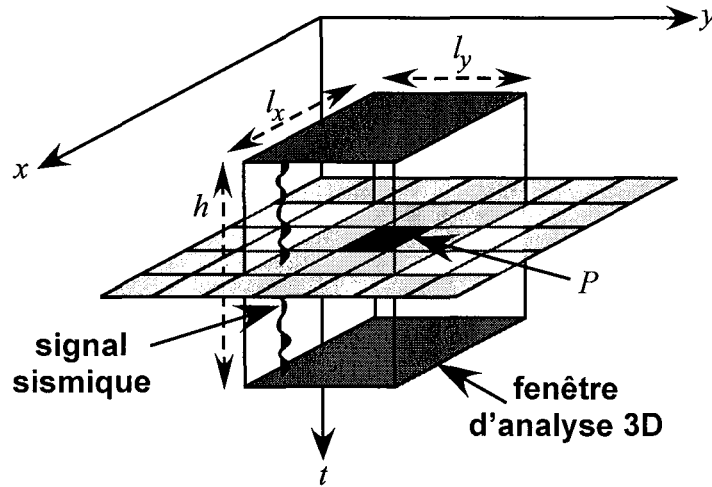
FIG. 2.11 – Fenêtre de calcul pour les attributs géométriques. L'attribut calculé au point P d'un cube sismique nécessite de connaître les valeurs du signal sur un groupe de traces directement voisines de ce point. En général, l_x et l_y sont identiques, et égaux à 3. L'attribut est souvent calculé au moyen de 9 traces sismiques. La hauteur h sur laquelle les traces sont considérées est variable, mais identique pour toutes les traces de la fenêtre.
