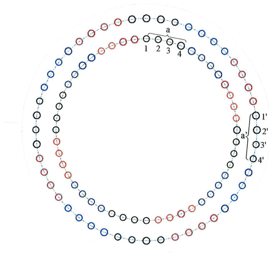
Fig.V.1. Sorties des bobines élémentaires sur le bornier
