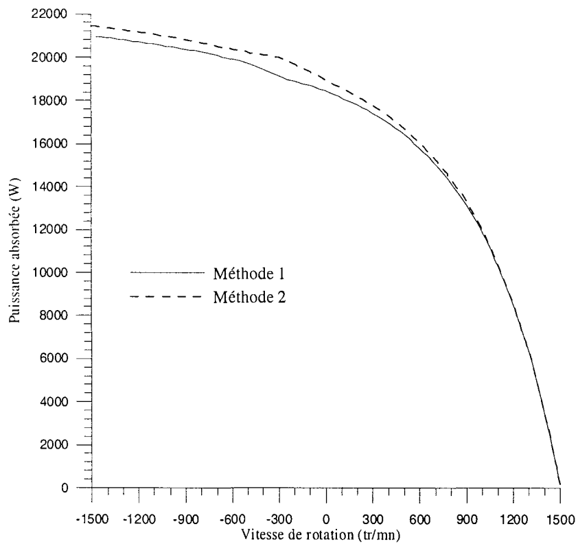
Fig.II.12. Puissance absorbée
