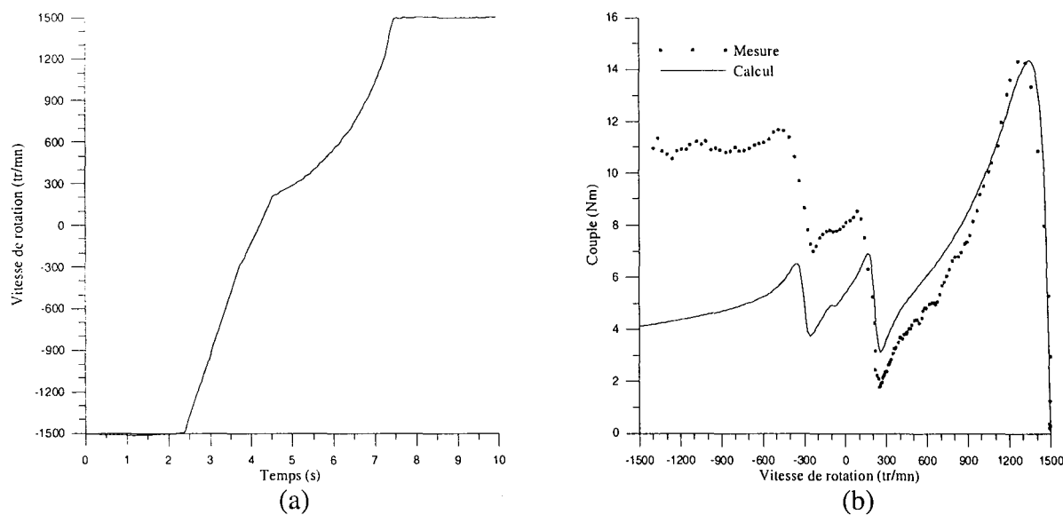
Fig.V.12. Vitesse mesurée (a) et comparaison des couples mesuré et calculé (b) (bobines B2 et B3 manquantes)
