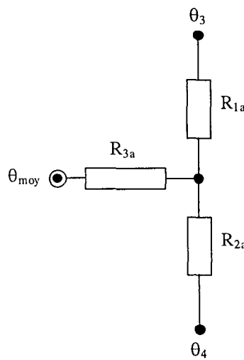
Fig.IV.7.Circuit thermique équivalent dans la direction axiale
