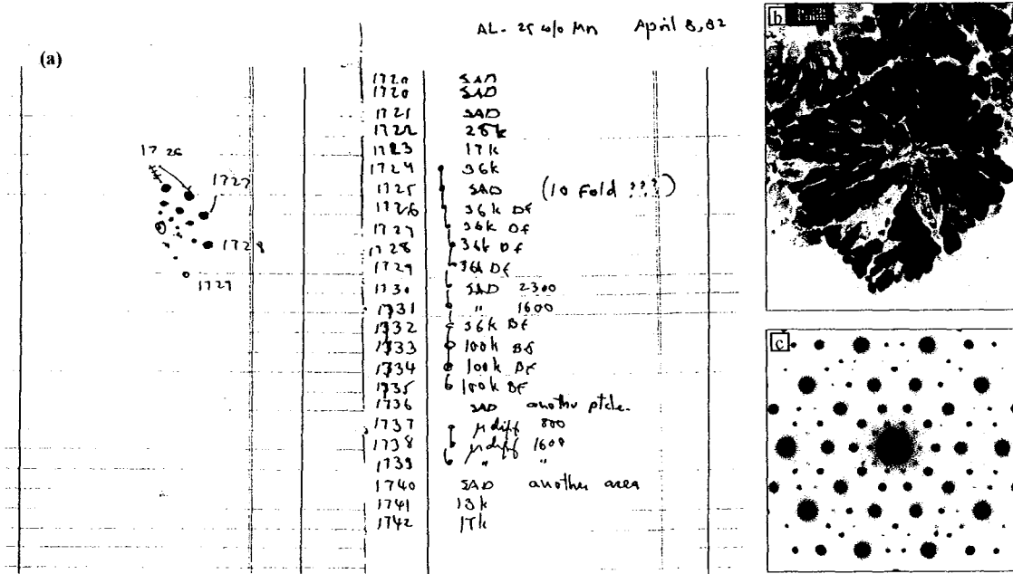
Figure I.1 : La découverte de Shechtman, sur un alliage AlMn hypertempéré. Extrait du cahier de laboratoire (a), négatif du cliché d'une particule icosaédrique (b) et négatif du diagramme de diffraction correspondant (c) (d'après [Shechtman-1997])
