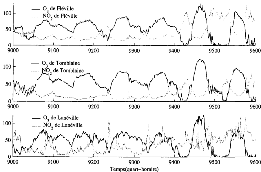
Figure 5.7 – Concentration d’ozone et de \text{NO}_2 des sites de Fléville, Tomblaine et Lunéville.
