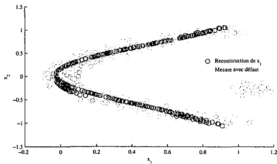
Figure 4.25 – Mesures et reconstruction de la courbe de l'exemple 2 avec un défaut sur x_1
