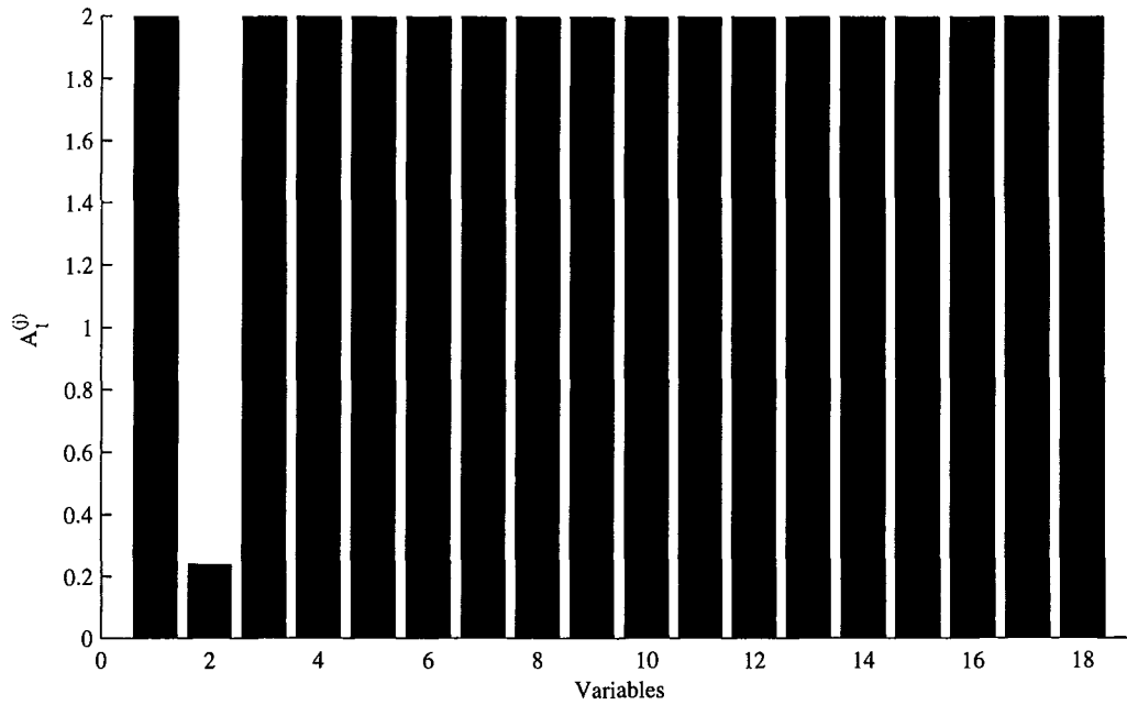
Figure 5.27 – Localisation par l'indice A_2^{(j)} calculé après la reconstruction de la j^{\text{eme}} variable.
