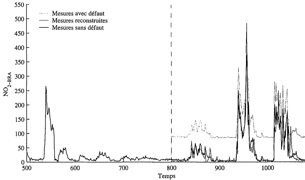
Figure 5.29 – Reconstruction de la variable en défaut du dioxyde d'azote de Brabois \text{NO}_2\text{-BRA} .
