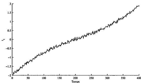
Figure 4.17 – Evolution de la première composante principale non-linéaire obtenue avec le réseau de neurones à cinq couches
