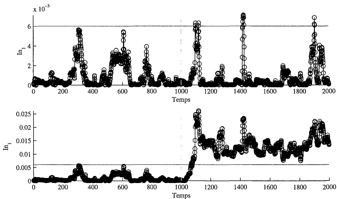
Figure 3.18 – Evolution de l'indice de détection In_1 en absence et en présence de défaut
