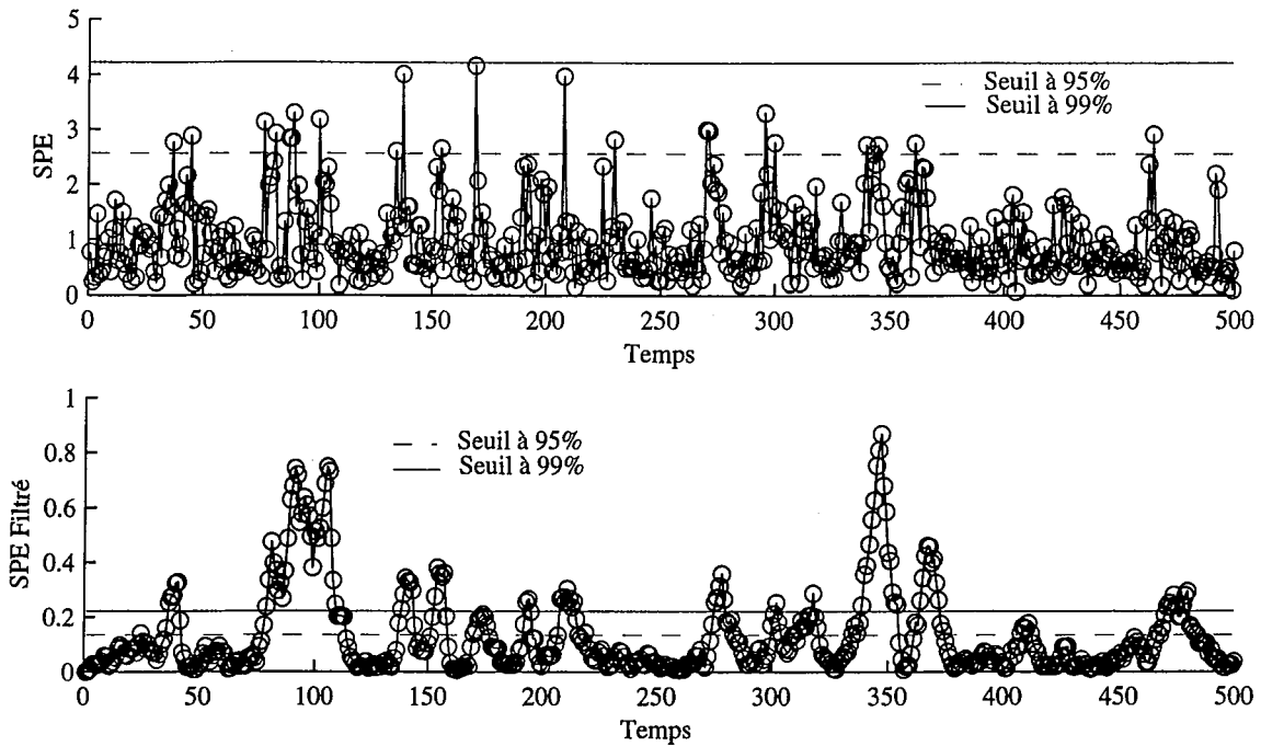
Figure 3.8 – Evolution du SPE et SPE filtré en absence de défaut (cas de l'exemple 2)
