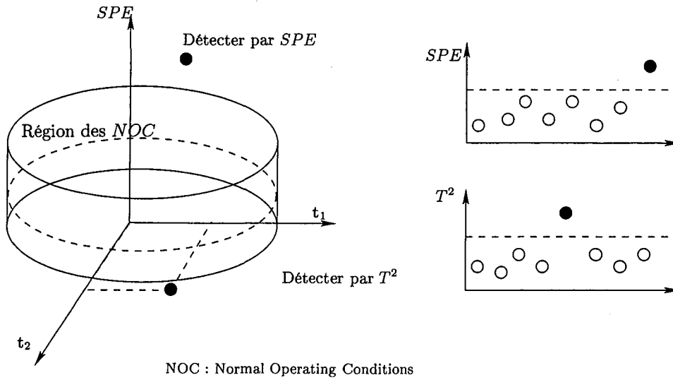
Figure 3.4 – Illustration graphique de la détection de défaut par les deux statistiques SPE et T^2
