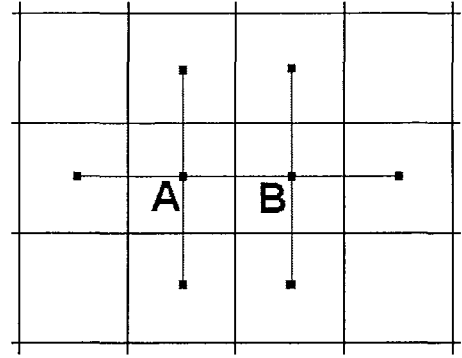
Fig. 6.1.2. Discretisation du front dans le domaine maillé
