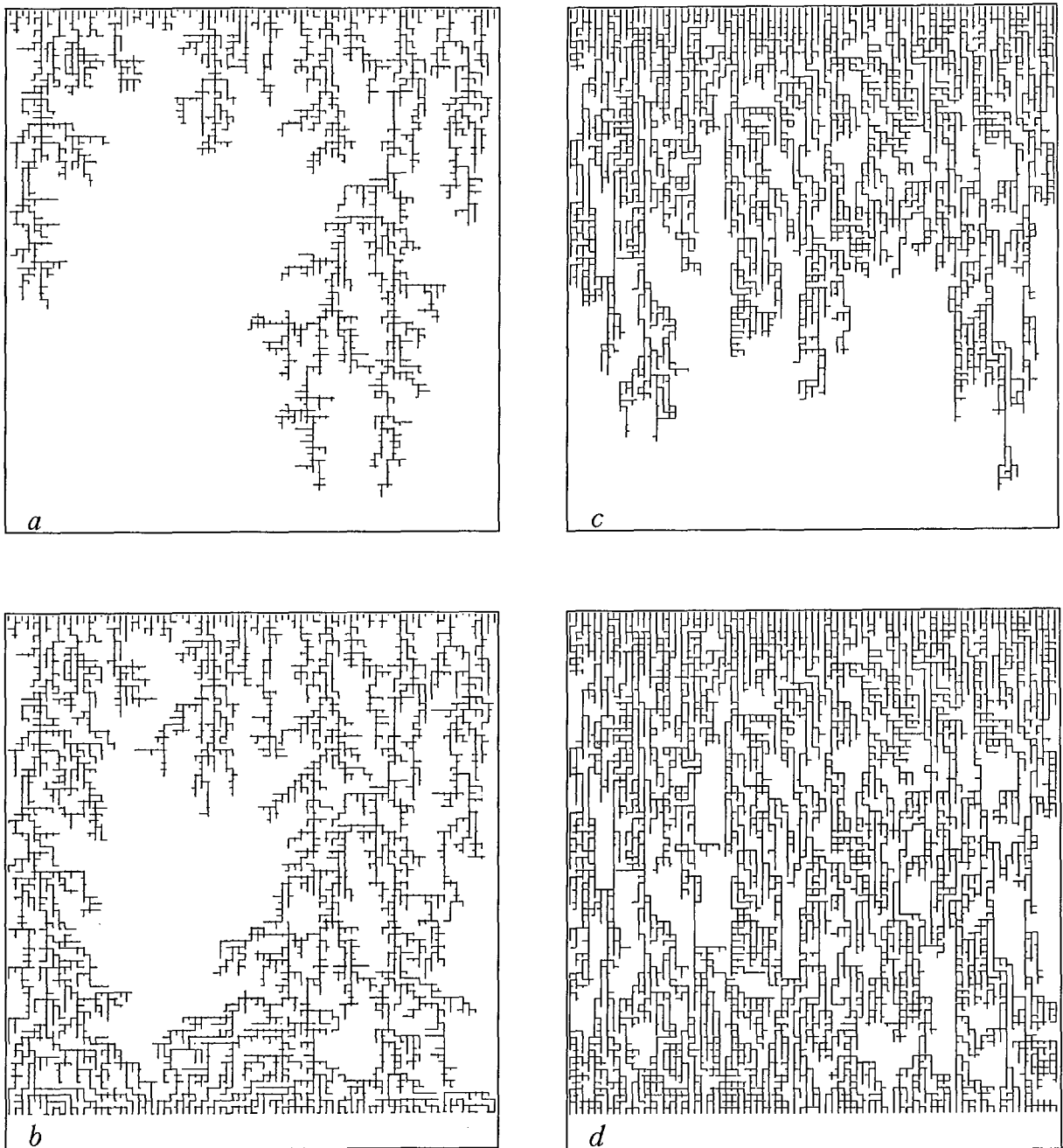
Fig. 4.1.3. Structure du cluster dans le cas 2D pour Ca=10^{10} et deux valeurs de \bar{\mu} : \bar{\mu}=0.01 (a, b) et \bar{\mu}=100 (c, d). Avant percolation (a, c) et après stabilisation complète (b, d)
