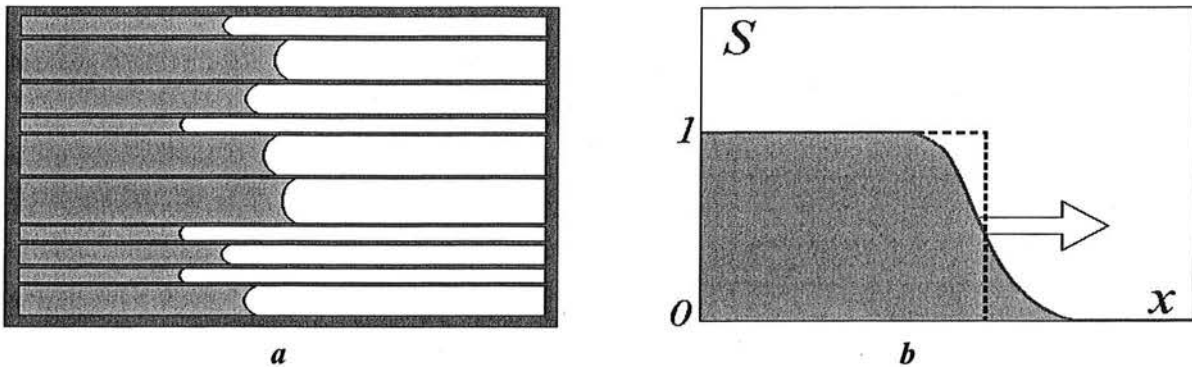
Fig. 2.2.2. Configuration de phases lors d'une imbibition en milieu hétérogène (a) et le profil de saturation de la phase déplaçante (b)
