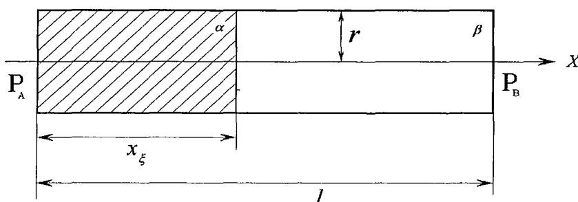
Fig. 3.2.1. Schéma du capillaire avec un ménisque : \alpha est la phase déplacante, \beta est la phase déplacée
