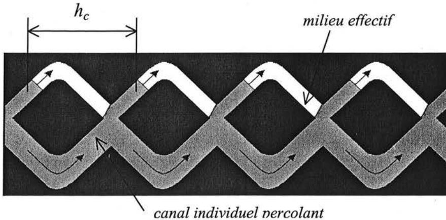
Fig. 2.3.7. Mécanisme de duplication des fronts mobiles
