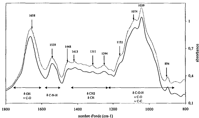
Figure III.20 : spectres FTIR originaux de la fraction de pentosanes (pentosanes : 40%, amidon : 15%, protéines : 29%, eau : 7%) bruts et secs dans des comprimés de KBr (--- Pentosane brut, — Pentosane sec). Les positions des bandes ( \text{cm}^{-1} ) indiquées sur les spectres correspondent à l'échantillon brut. Les spectres ont été réalisés en transmission, au moyen d'un spectromètre à transformée de Fourier.
