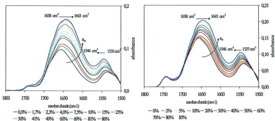
Figure III. 42 : spectres FTIR lissés et corrigés en ligne de base des bandes amide I et II d'un dépôt de la farine en équilibre à différentes a_w comprises entre 0 et 0,86.
