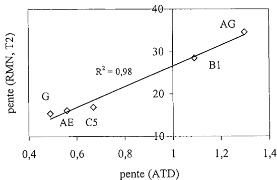
Figure III. 51 : comparaison des pentes de la droite « % eau congelable = f (% eau totales » obtenue à partir des résultats d'analyse thermique différentielle, et de la droite « T2 = f (% eau totales » obtenue par RMN du proton basse résolution (20MHz). Gamme d'hydratation étudiée : 40 – 80 % m.s. d'eau totale.
