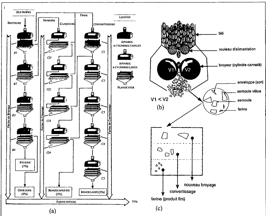
Figure I. 2 : (a) exemple de diagramme de mouture d'une minoterie industrielle. Schéma de fonctionnement d'un broyeur à cylindre (b) et d'un plansichter (c), d'après FEILLET [2000].
