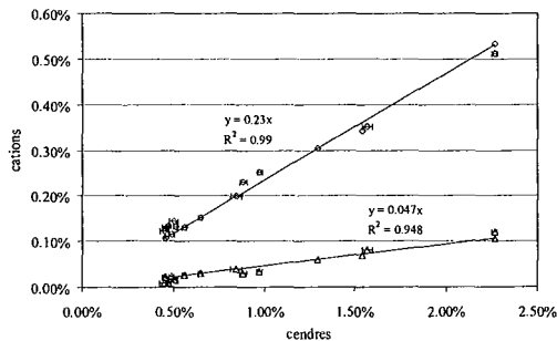
Figure III. 2 : relation entre la teneur en cendres sur les concentrations en K et Mg des farines mesurées par spectroscopie d'absorption atomique. \diamond : K, \Delta : Mg.
