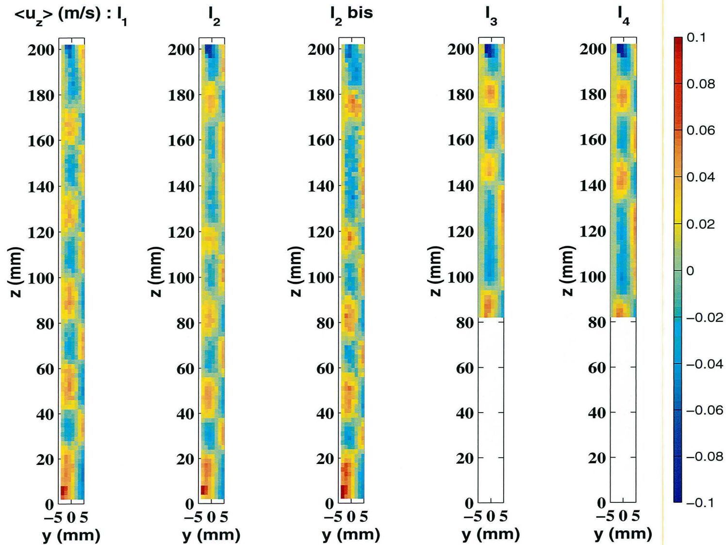
FIG. 4.16 - N = 300tr/min . Vitesse axiale \langle u_z \rangle en m \cdot s^{-1} . y = r - 48(mm) . Le cylindre intérieur est à gauche y = -7mm .
