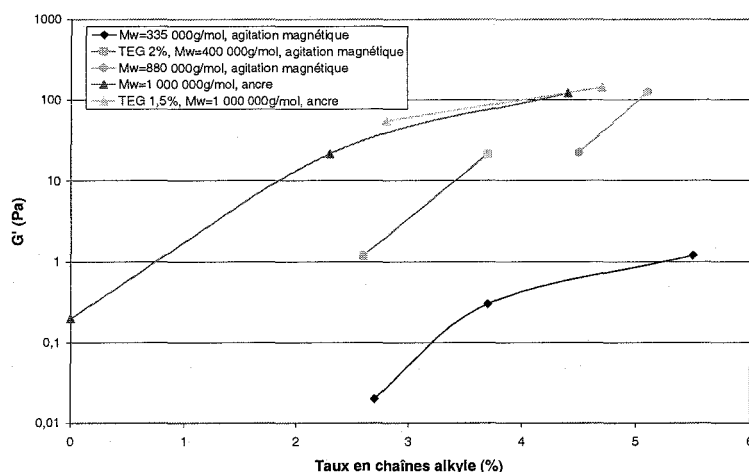
Figure 21 : Variation de G' en fonction du taux en C_{12} et du mode opératoire ( 10 \text{ g.L}^{-1} dans \text{NaCl } 0,15 \text{ mol.L}^{-1} , 37^\circ\text{C} , mesuré à une contrainte de 1 \text{ Pa} et à une fréquence de 1 \text{ rad.s}^{-1} )
