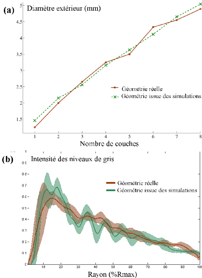
Illustration III 22: Comparaison entre les géométries d'une matrice réelle (8 couches, d_{\text{libre}}=200 \mu\text{m} , h=100 \text{mm} ) et de la configuration initiale correspondante. (a) Comparaison entre les diamètres extérieurs moyens (b) Distribution des fibres dans les sections des matrices.
