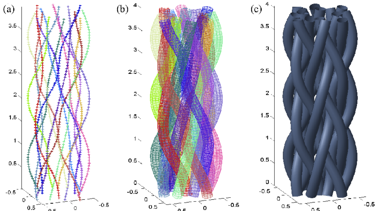
Illustration III 3: (a) Détermination des trajectoires à partir de la cinématique des fibres durant le tressage. (b) Création de tubes sous l'hypothèse de rayon constant. (c) Géométrie finale.
