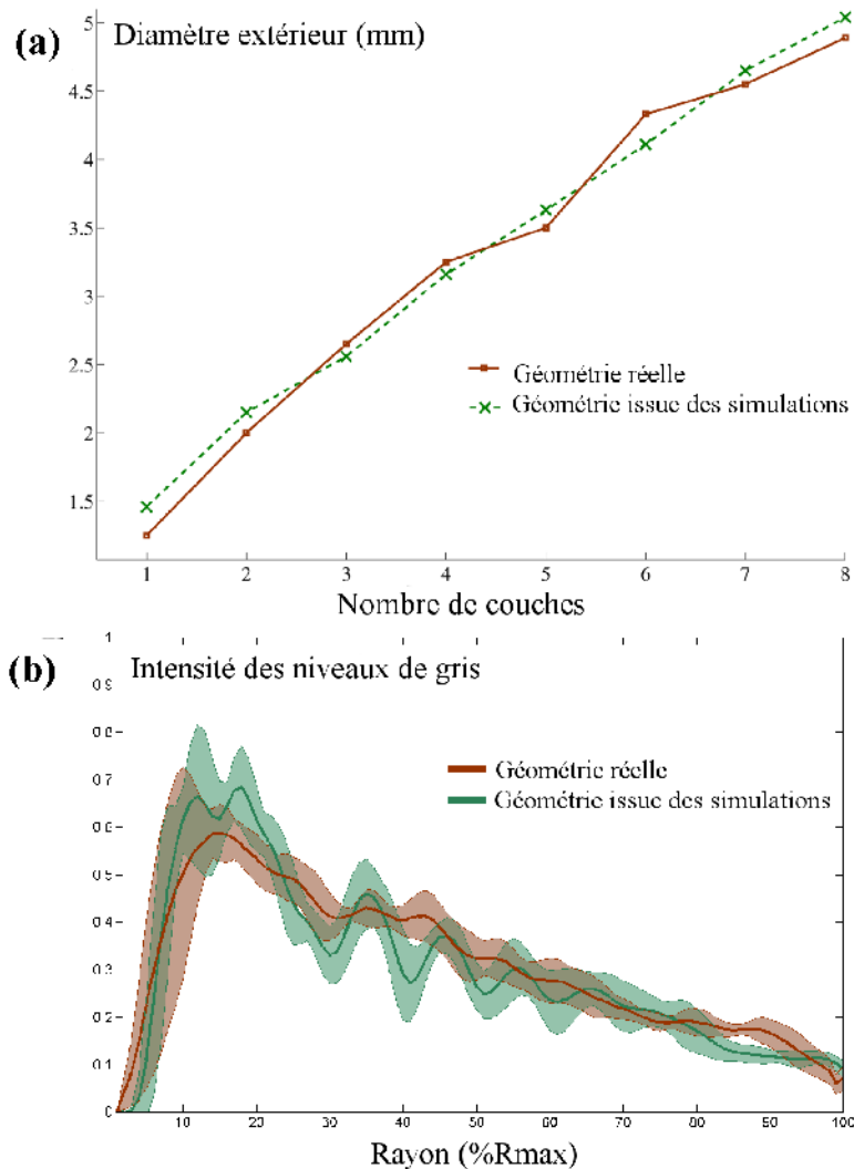
Illustration III 22: Comparaison entre les géométries d'une matrice réelle (8 couches, d_{\text{libre}}=200 \mu\text{m} , h=100 \text{ mm} ) et de la configuration initiale correspondante. (a) Comparaison entre les diamètres extérieurs moyens (b) Distribution des fibres dans les sections des matrices.
