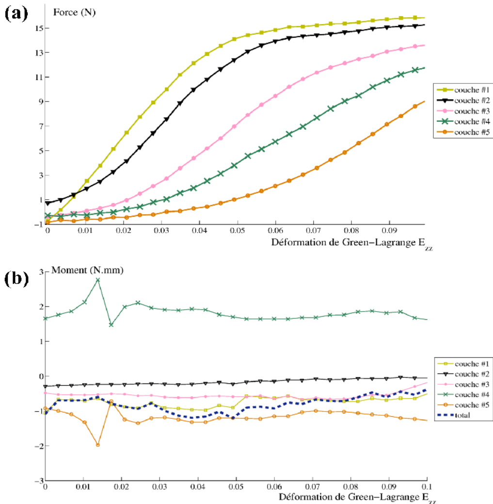
Illustration III 18: (a) Efforts et (b) moments dans chaque couche en fonction de la déformation de Green-Lagrange F_{zz} pour la simulation d'un essai de traction ( F_{zz}=0.01 ) sur une matrice de cinq couches. Les couches sont numérotées du centre à la périphérie de la matrice.
