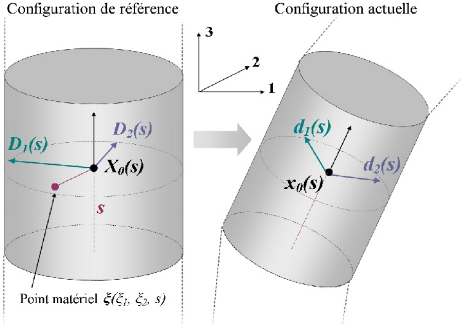
Illustration III 13: Vecteurs directeurs D_1 et D_2 dans une section quelconque d'abscisse curviligne s pour les configurations de référence et actuelle.
