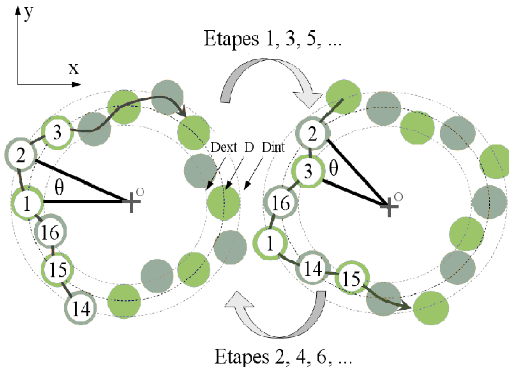
Illustration III 2: Cinématique du procédé de tressage. Entre chaque étape successive, chaque groupe de fibres (dont certaines ici sont numérotées) alterne entre les diamètres D_{int} , D et D_{ext} , et tourne d'un angle \pm\theta .
