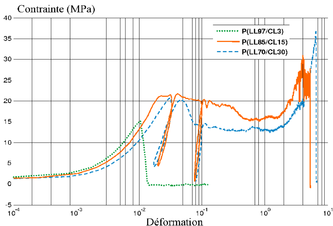
Illustration II 6: Réponses typiques en traction des fibres de P(LL97/CL3), P(LL85/CL15) et P(LL70/CL30) (échelle semi-logarithmique)
