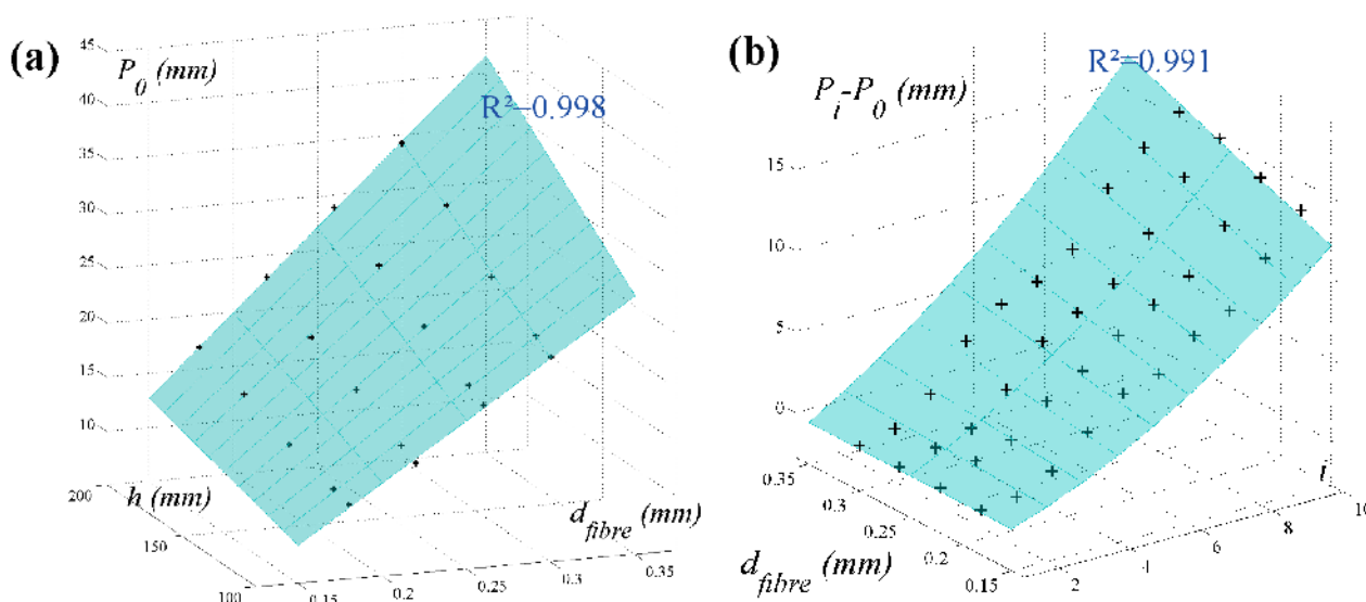
Illustration 9: Surfaces des moindres carrés utilisées pour modéliser (a) le pas de tressage initial P_0 de la première couche (b) l'évolution du pas de tressage en fonction du nombre de couches.
