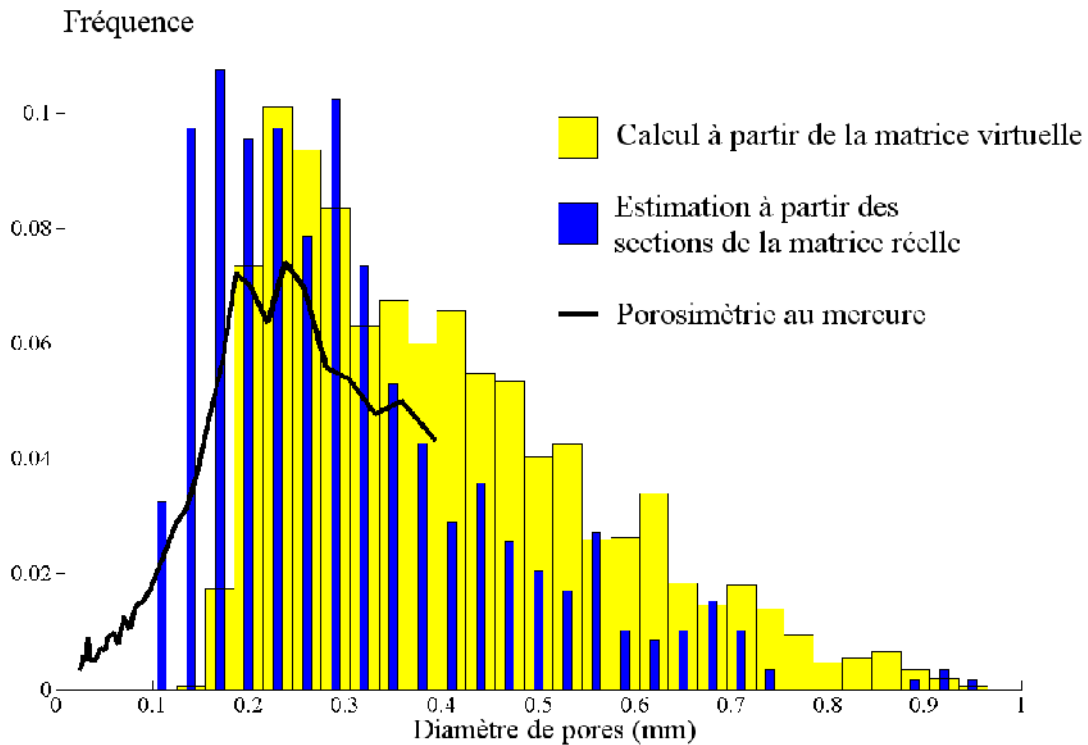
Illustration III 11: Comparaison entre la distribution de tailles de pores obtenues par calcul dans la matrice virtuelle, par calcul dans les sections de la matrice réelle, et par porosimétrie mercure.
