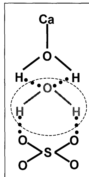
Figure 2.4 - Squelette atomique d'une molécule de \text{CaSO}_4 \cdot 2\text{H}_2\text{O} mettant en évidence une molécule d'eau très faiblement liée au reste de la molécule (d'après Mandal et Mandal, 2002)
