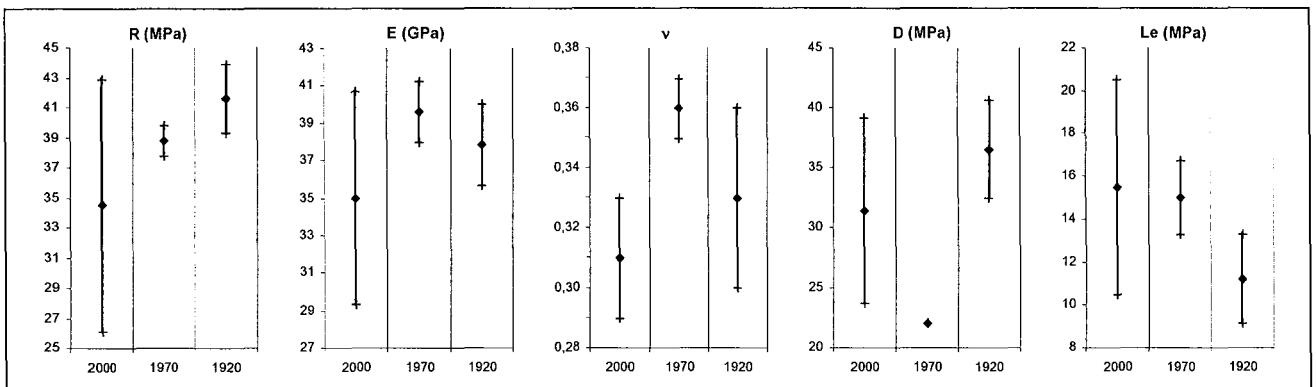
Figure 4.28 - Grozon – Dispersion de différents paramètres mécaniques en fonction de l'âge d'exploitation (valeurs moyennes et écarts-types)
