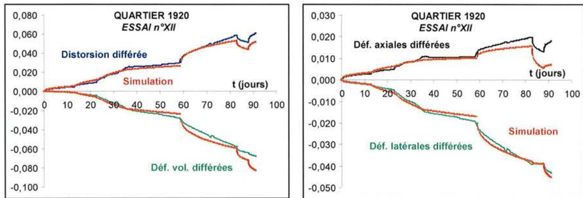
Figure 6.1.11 - Grozon – Age d'exploitation 1920 – Hygrométrie 90% Evolution de la distorsion, des déformations volumiques, axiales et latérales différées et simulation
