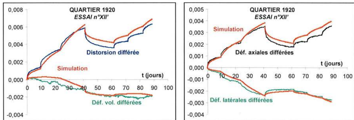
Figure 6.1.12 - Grozon – Age d'exploitation 1920 – Hygrométrie 75% Evolution de la distorsion, des déformations volumiques, axiales et latérales différées et simulation
