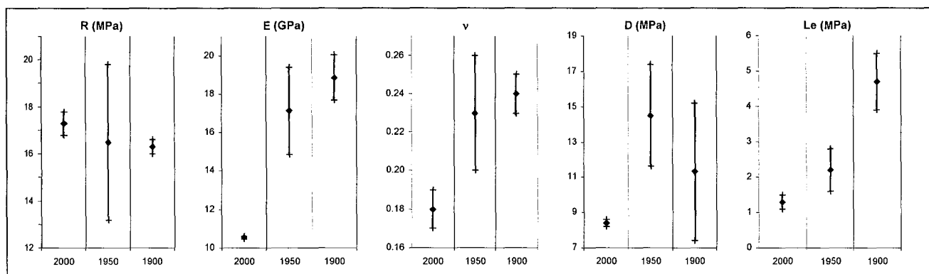
Figure 4.19 - Dispersion de différents paramètres mécaniques en fonction de l'âge d'exploitation (valeurs moyennes et écarts-types)
