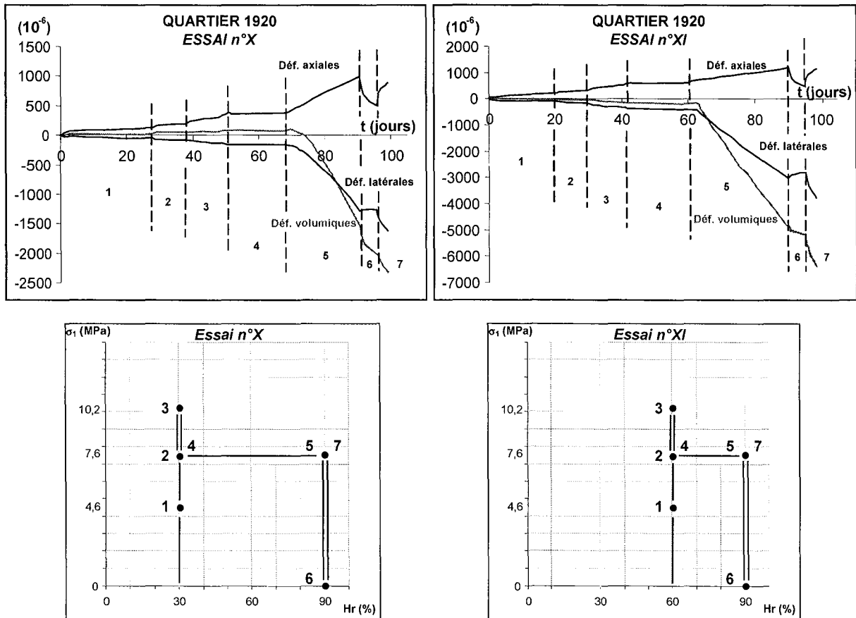
Figure 5.24 - Grozon – Age d'exploitation 1920 – Courbes déformation-temps de deux essais de fluage multiplicatif sous des hygrométries initiales de 30% et 60% (les différentes contraintes uniaxiales et hygrométries sont précisées ; les échelles des axes des abscisses et des ordonnées ne sont pas les mêmes)
