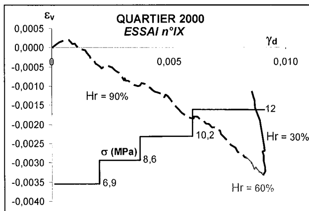
Figure 6.17 - Essai n°IX – Evolution des déformations volumiques en fonction de la distorsion différée (la contrainte et l'hygrométrie varient)
