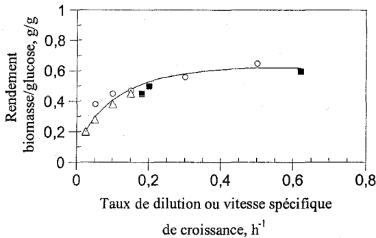
Figure III-18 : relation entre la vitesse spécifique de croissance et le rendement de conversion de glucose en biomasse pendant les cultures continues à 33°C (○) et 37°C (Δ) et discontinues à 33°C (■).
