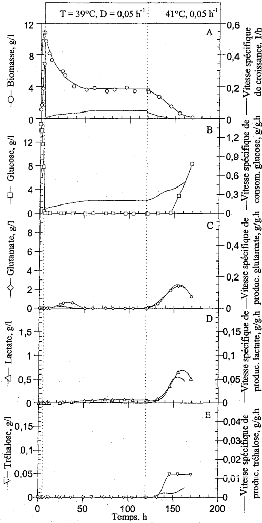
Figure III-13 : cinétiques en culture continue à 39 et 41°C et à taux de dilution de 0,05 \text{ h}^{-1} des cellules sélectionnées de la culture continue à 39°C et à taux de dilution de 0,05 \text{ h}^{-1} .
