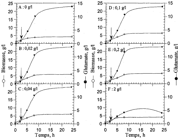
Figure V-4 : effet de différentes concentrations de palmitate sur la croissance de C. glutamicum
