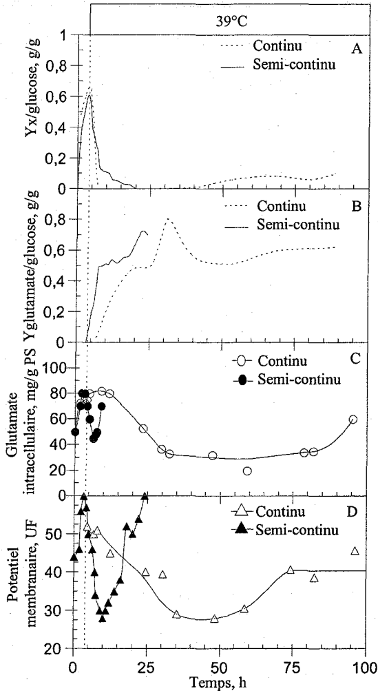
Figure III-17 : comparaison des cinétiques à 39°C de la culture continue à taux de dilution de 0,05 h -1 et semi-continue.
