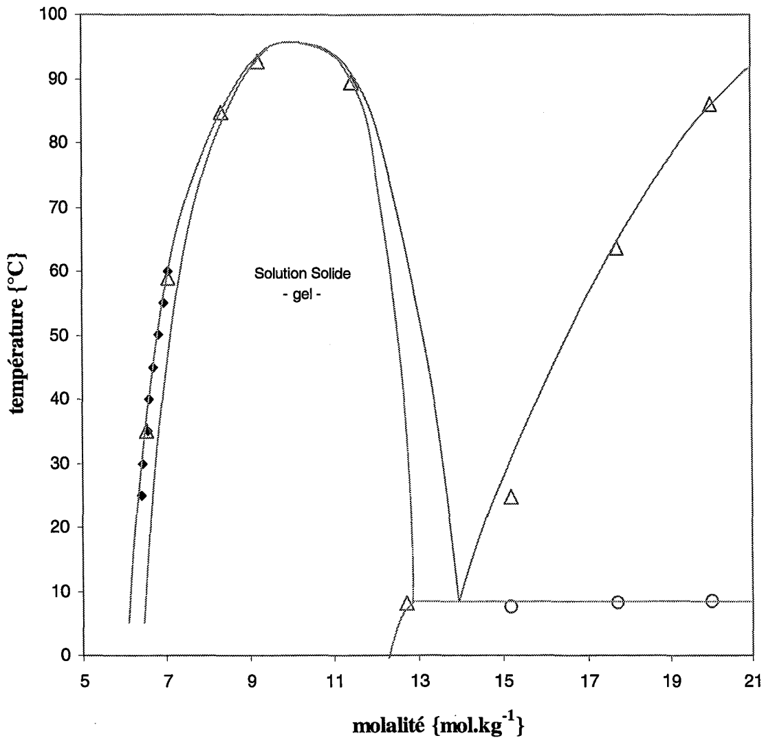
Figure IV. 9 Représentation de la molalité des solutions saturées en capronate de potassium (◆) obtenue par analyse de la phase saturée ; (Δ) et (○) obtenue par DSC
