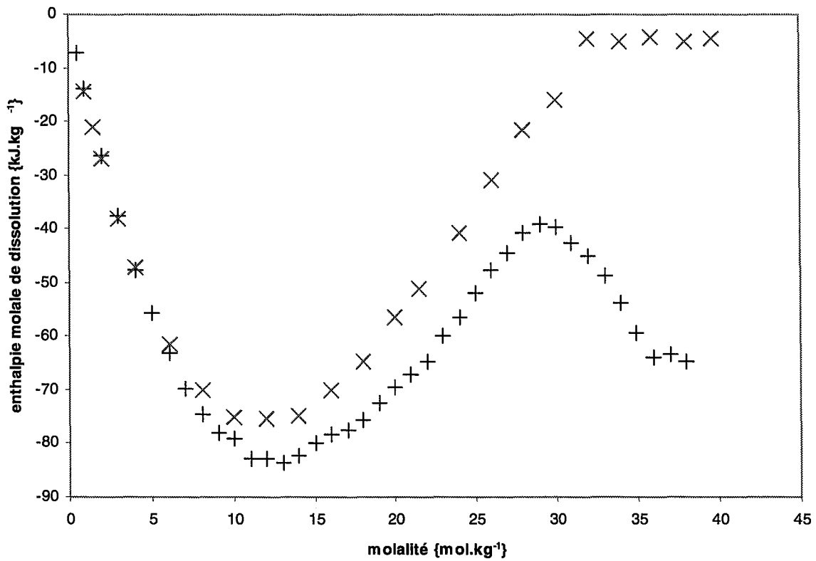
Figure II. 11 Enthalpie molale de dissolution à 25°C (+) ; à 50°C (x).
