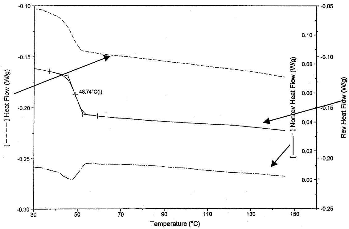
Figure II-32 : Thermogramme MDSC du copolymère Dex_{29K}Si_{80-g-60}PLA_{2K} .
