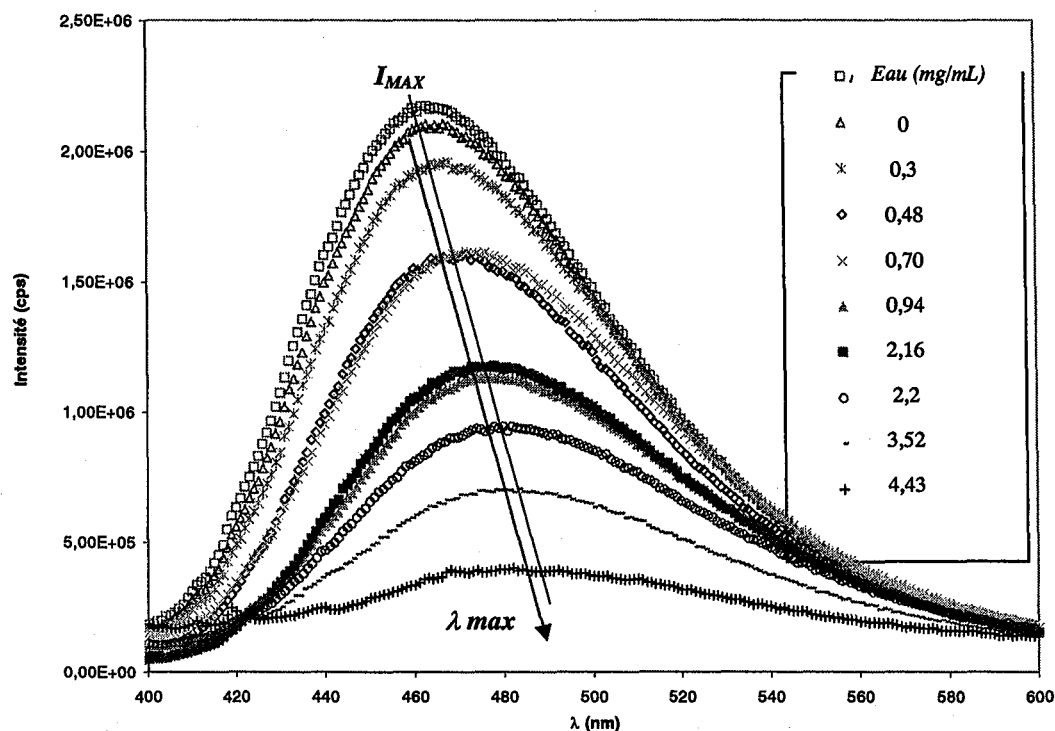
Figure III-19 : Spectres d'émission de fluorescence de l'ANS en fonction de la teneur en eau dans le système copolymère Dex_{29K}\text{-}g\text{-}18\text{-}PLA_{1,7K} /toluène/ eau, à 25°C.
