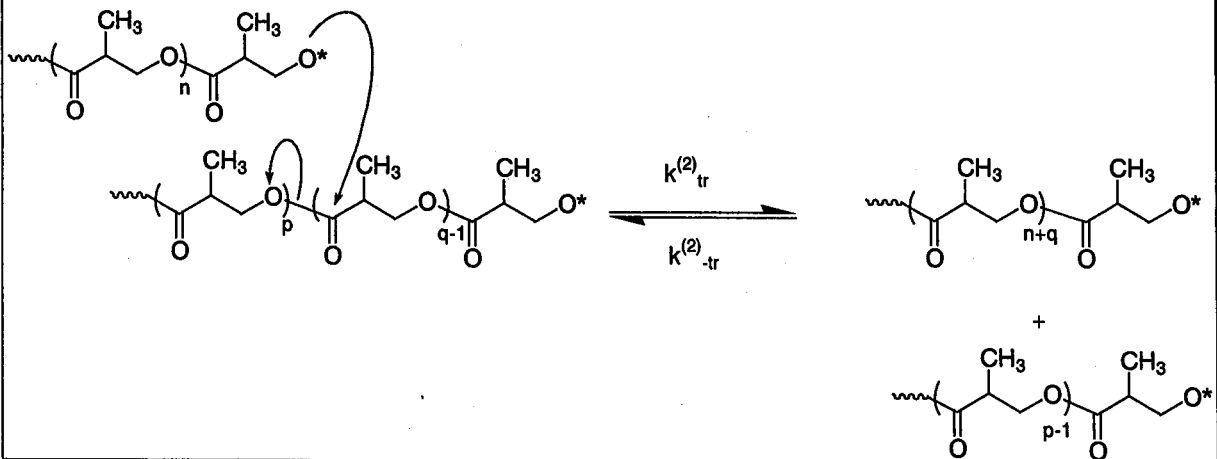
Schéma II-10 : Equilibres intervenant lors la polymérisation par ouverture du lactide.
