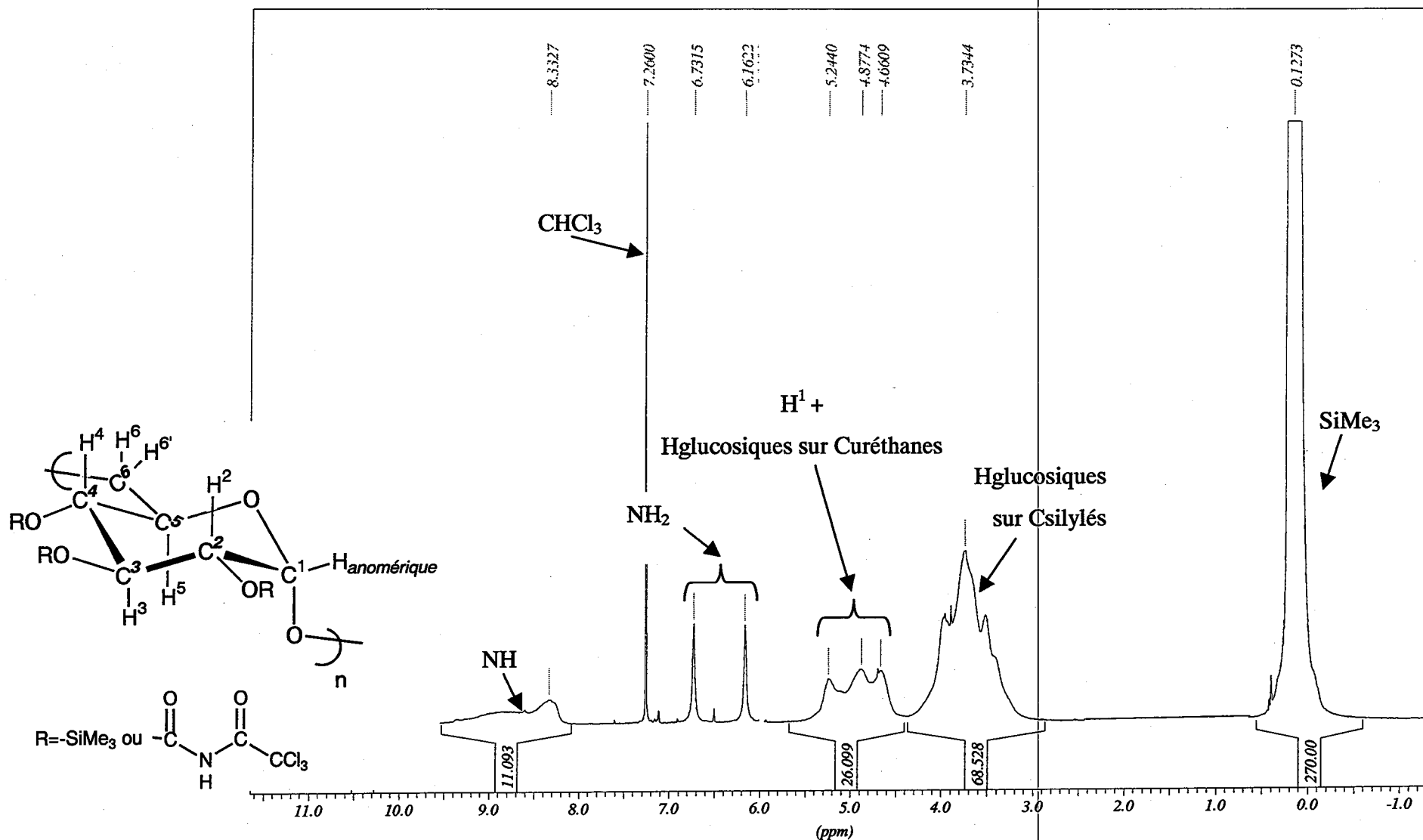
Figure II-18 : Spectre RMN 1 H d'un dextrane partiellement silylé après réaction avec le trichloroacétylisocyanate (CDCl 3 , 74% de silylation)
