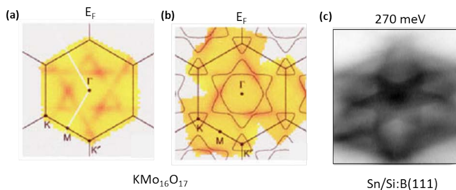
FIG 4.24 – (a) Cartographie d'intensité pour KMo_{16}O_{17} à E_F avec la zone de Brillouin et les points de symétrie ; (b) calcul dans l'approximation de liaison forte du KMo_{16}O_{17} [35] et (c) Cartographie d'intensité pour Sn/Si(111):B à 270 meV.
