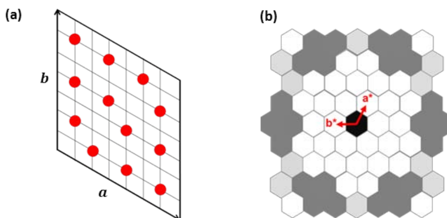
FIG. 5.7 – Calcul du facteur de structure de la surface Si(111)-7x7. (a) Modèle atomique des adatoms et (b) Distribution des intensités en différentes zones de Brillouin de la (7x7) selon le facteur de structure. Une plus grande intensité correspond aux couleurs plus foncées.
