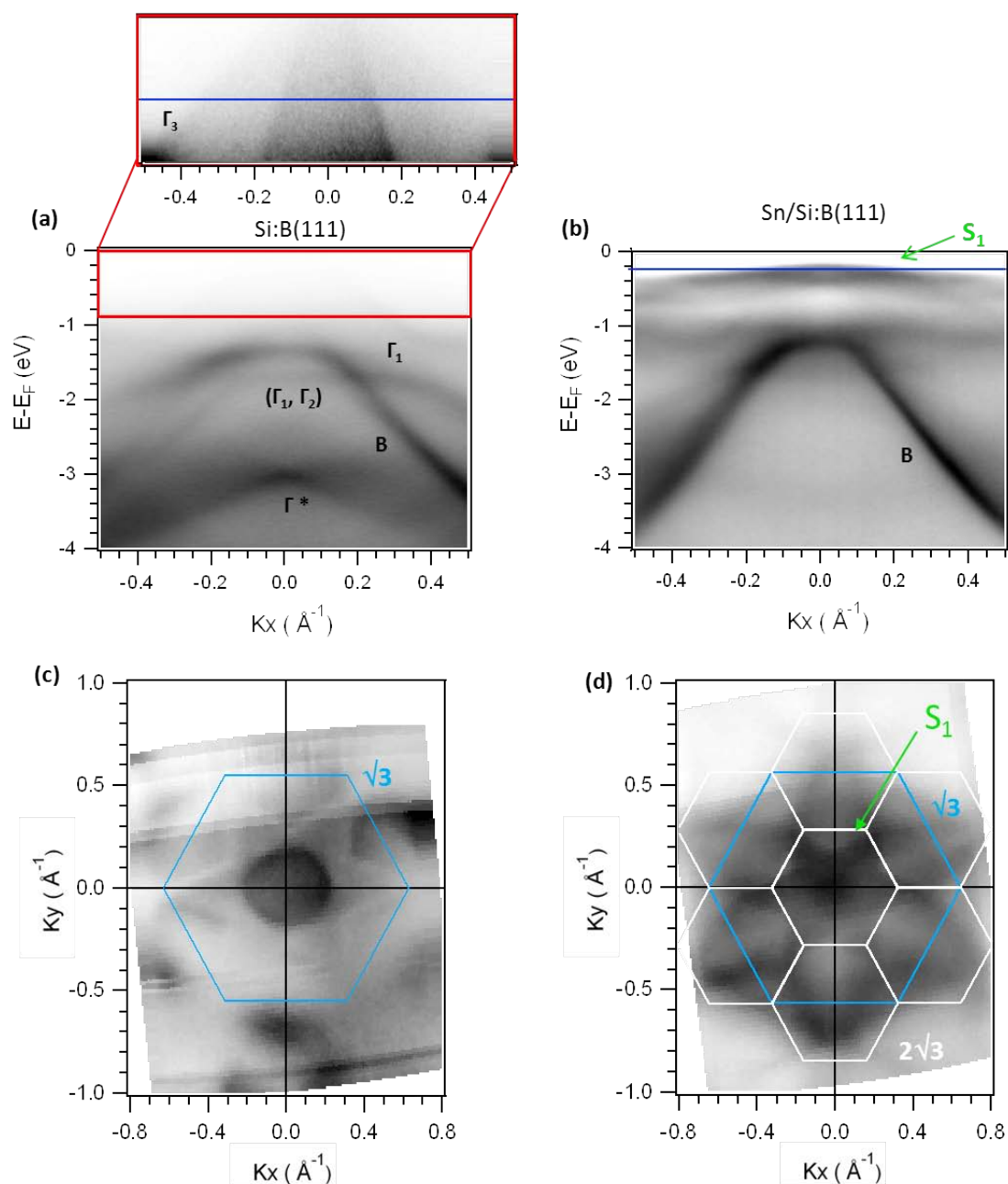
FIG 4.23 – (a-b) Structure de bandes mesurée à h\nu = 27 eV et à T = 300 K dans la direction \overline{\Gamma\bar{K}} . (a) Le substrat Si(111) :B. Les notations \Gamma_i et B indiquent les différents états de surface et la bande de volume du substrat respectivement. Le rectangle rouge indique l'endroit où nous avons changé le contraste de la figure pour montrer le continuum des bandes de volume. La ligne bleue désigne l'endroit de la coupe effectuée en c ; (b) Après un dépôt d'étain à 620 °C. La ligne bleue désigne l'endroit de la coupe effectuée en d. S_1 indique l'état de surface induit par l'étain. (c-d) Coupes isoénergétiques relatives pour chaque structure de bande à 550 et 275 meV qui correspondent à une énergie de 275 meV par rapport de la bande de volume. Dans Sn/Si(111) :B cela correspond à la coupe à travers S_1 . Ce décalage est dû à un déplacement de la bande de volume (B) après le dépôt de Sn. Les hexagones en bleu et blanc indiquent les zones de Brillouin de la reconstruction \sqrt{3} et 2\sqrt{3} respectivement. Les zones sombres correspondent à celles où l'intensité est plus grande.
