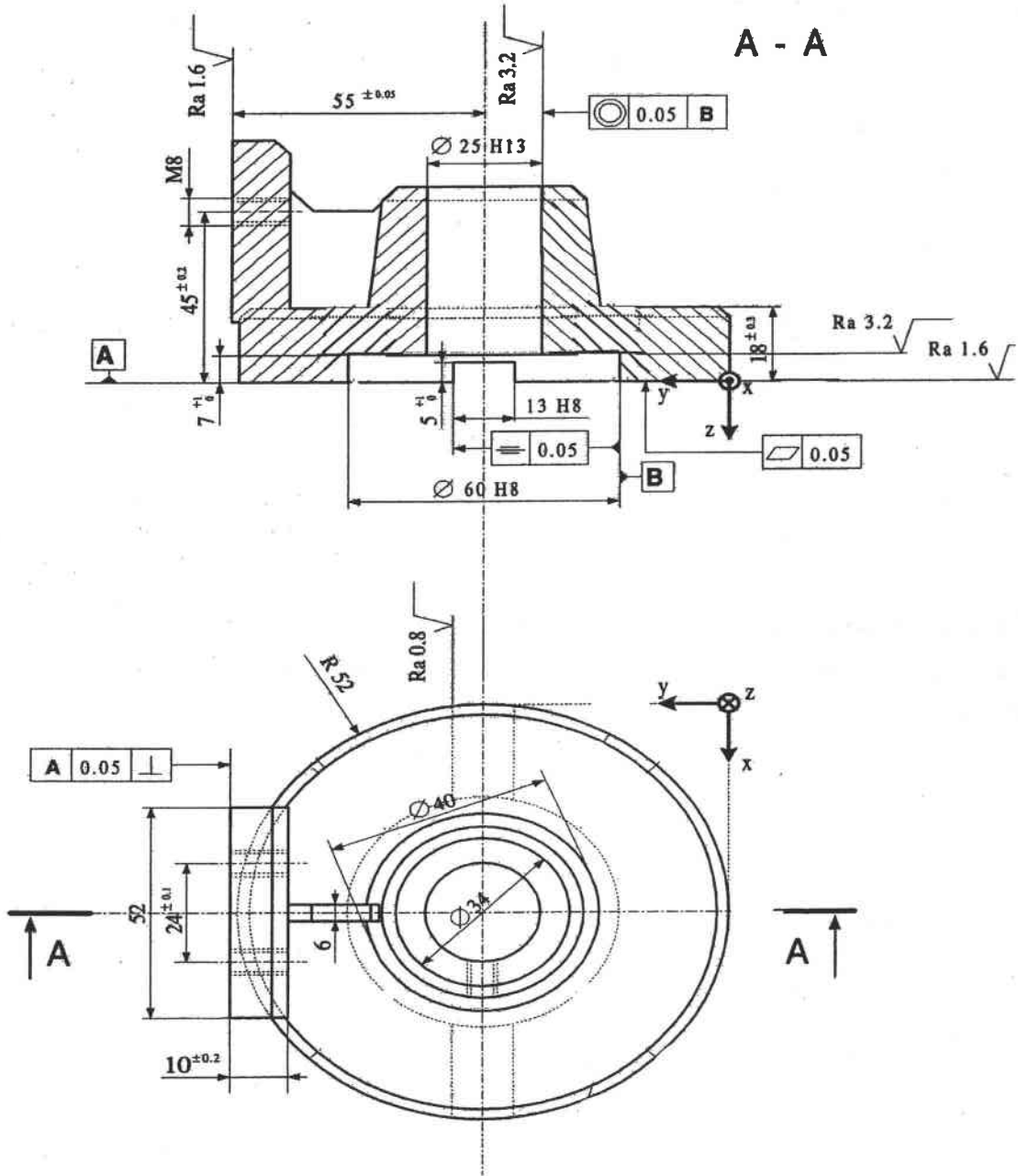
Figure 112. Dessin de définition de la pièce Termoz
