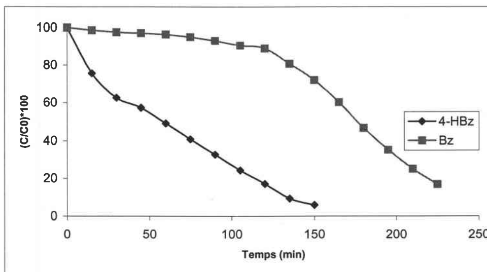
Figure 1 : Cinétique de photodégradation du mélange 4-HBz et Bz par \text{TiO}_2 P25.
