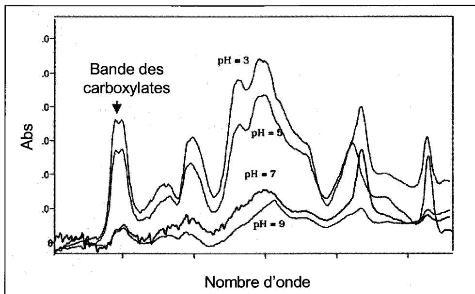
Figure 10 : Spectres DRIFT de l'acide 4-HBz adsorbé sur TiO 2 .
