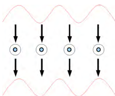
FIG. 4.3 – Illustration du principe de causalité circulaire.
