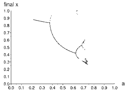
(d) Diagramme de bifurcations reconstruit sur les données de simulation avec N = 1500 fourmis logistiques, \epsilon^0 = 0.5 and m = 500
