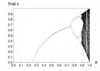
FIG. 10.1 – Diagramme de bifurcation de l'application logistique
