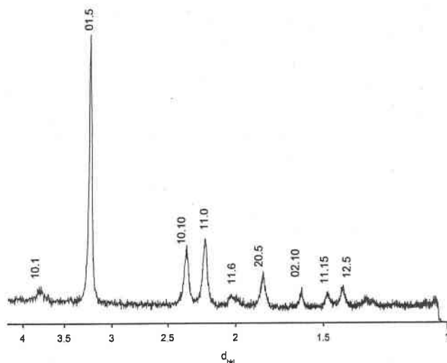
figure 13 : cliché de diffraction des rayons X réalisé sur un composé électrodéposé à partir d'une solution de rapport Bi/Te = 1 à une concentration de 2 \cdot 10^{-2} M pendant un temps de 2h, à E = -250 mV/ECS, sur un support constitué de Si / SiO 2 / 150 nm Cr / 100 nm Ni
