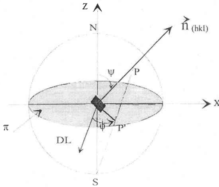
figure 8 : sphère des pôles
