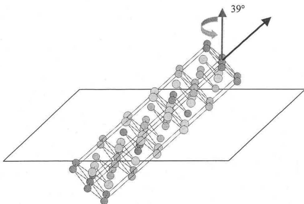
figure 42 : : position de l'axe c par rapport à la surface dans le cas d'une orientation suivant le plan {10.10}
