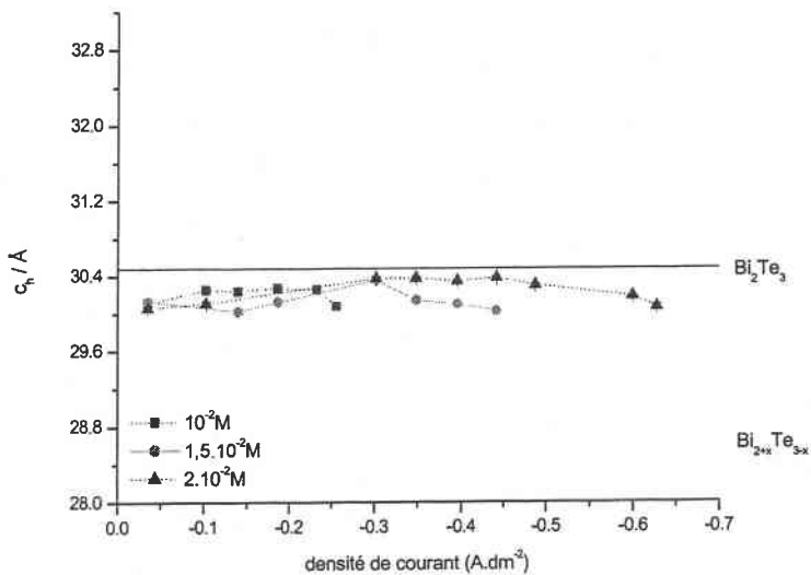
figure 35 : évolution des paramètres de maille en fonction de la densité de courant pour une solution de rapport Bi/Te = 1 à des concentrations de 10^{-2} M, 1,5.10^{-2} M et 2.10^{-2} M
