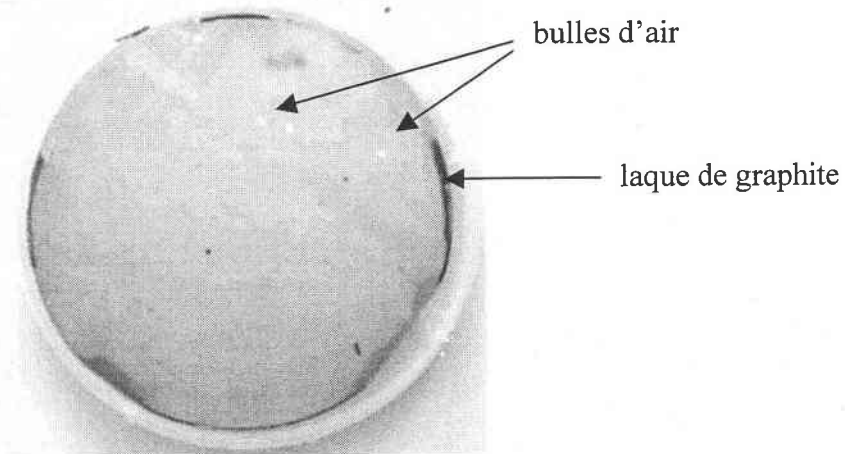
figure 26 : wafer de tellure de bismuth obtenu à partir d'une solution de rapport Bi/Te = 1 à une concentration de 2.10^{-2} M, à une densité de courant de -0,3 A.dm -2
