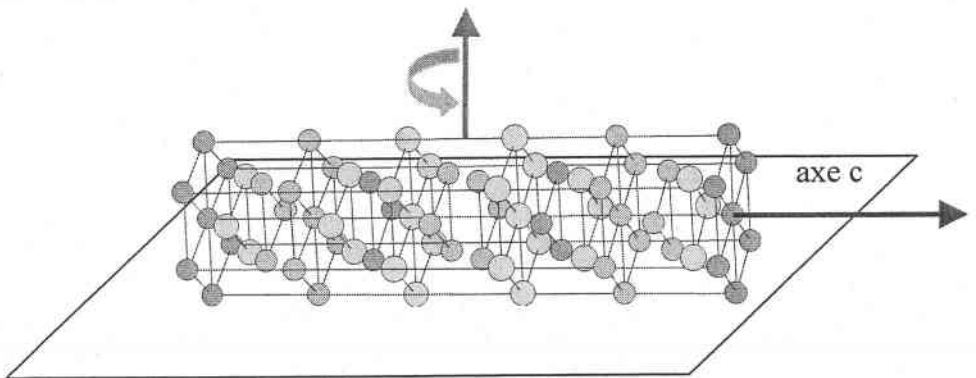
figure 41 : position de l'axe c par rapport à la surface dans le cas d'une orientation suivant le plan {11.0}
