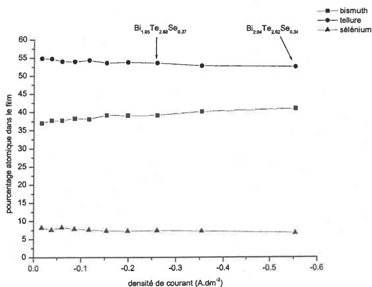
figure 17 : évolution de la stœchiométrie en fonction de la densité de courant appliquée pour un électrolyte contenant 60% Bi ( 2.10^{-2} M) – 36% Te ( 1,2.10^{-2} M) – 4% Se ( 1,3.10^{-3} M), i_{imp} = - 0,1 A ; t = 35 min
