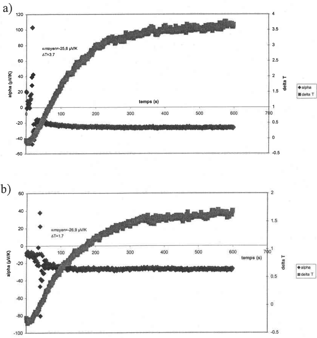
figure 24 : évolution du coefficient Seebeck pour un composé \text{Bi}_{2,05}\text{Te}_{2,95} électrodéposé à partir d'une solution de rapport Bi/Te = 1 à une concentration de 10^{-2} M, a) 1 er essai, b) essai réitéré
