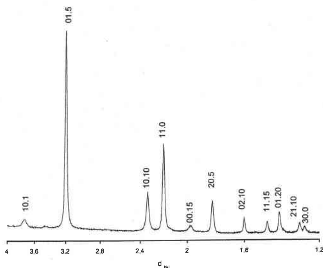
figure 5 : cliché de diffraction obtenu pour une solution contenant 70%Bi - 25% Te – 5% Se à un potentiel de -75 mV/ECS, t = 2h
