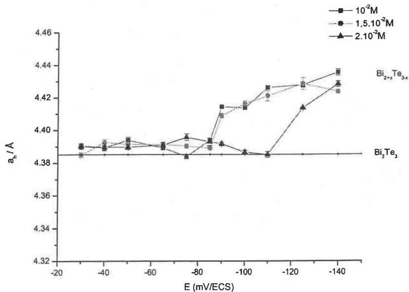
figure 15 : évolution du paramètre de maille a_h en fonction du potentiel à partir d'une solution de rapport \text{Bi}/\text{Te} = 1 pour des concentrations de 10^{-2} M ; 1,5 \cdot 10^{-2} M et 2 \cdot 10^{-2} M en bismuth
