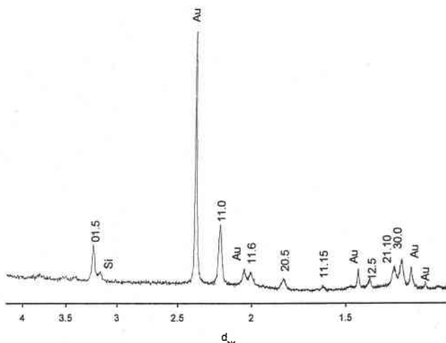
figure 22 : cliché de diffraction des rayons X réalisé sur un composé électrodéposé à partir d'une solution constituée de 60% Bi – 36% Te – 4% Se à une concentration de 2 \cdot 10^{-2} M en bismuth pendant un temps de 2h, à j = -0,28 \text{ A.dm}^{-2} , sur un support constitué Si / SiO 2 / NiCr (30 nm) / Au (70 nm)
