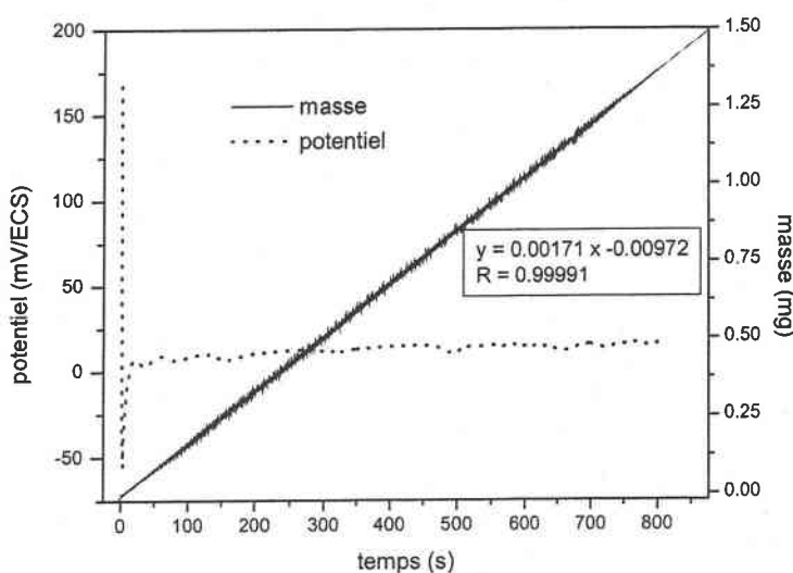
figure 33 : évolution de la prise de masse (mg) et du potentiel (mV/ECS) pour un composé électrodéposé à partir d'une solution de rapport \text{Bi/Te} = 1 à j = -0,28 \text{ A.dm}^{-2} [94]
