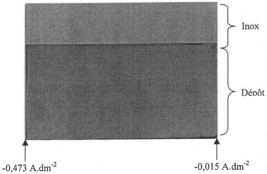
figure 27 : cellule de Hull sur une solution de rapport Bi/Te de concentration 10 -2 M, i_{imp} = - 85 mA, temps = 30 min
