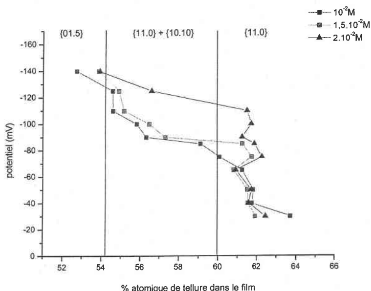
figure 20 : évolution de la texture des composés en fonction du pourcentage atomique de tellure
