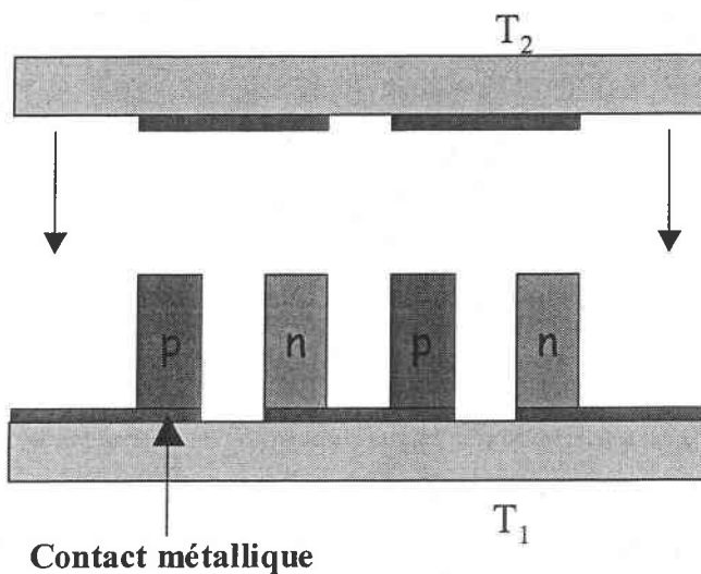
figure 2 : concept mis en place par l'équipe de Fleurial
