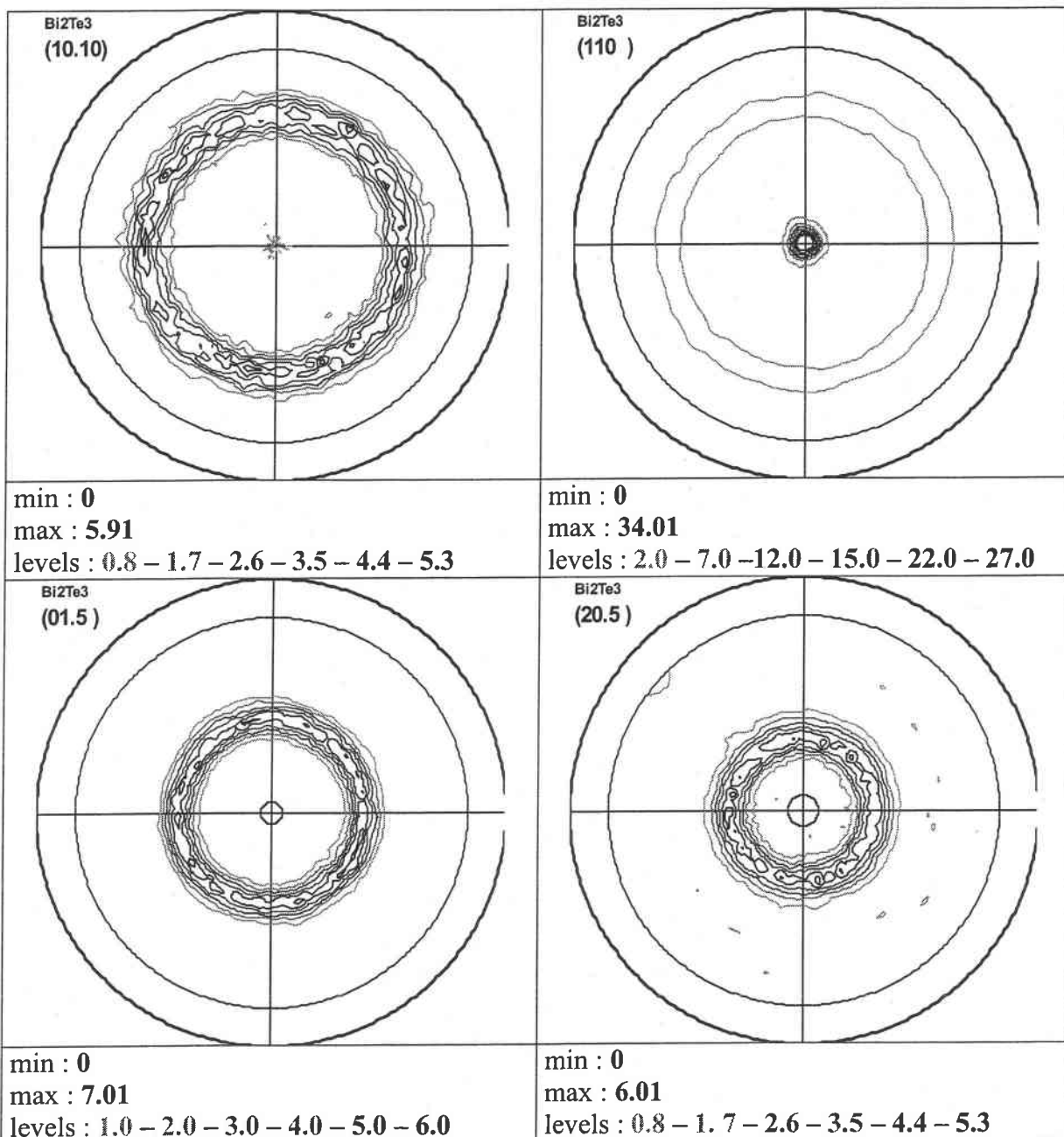
figure 37 : figures de pôles pour un échantillon électrodéposé à partir d'une solution de rapport Bi/Te = 1 et à une concentration de 1,5 \cdot 10^{-2} M, à j = -0,25 \text{ A.dm}^{-2}
