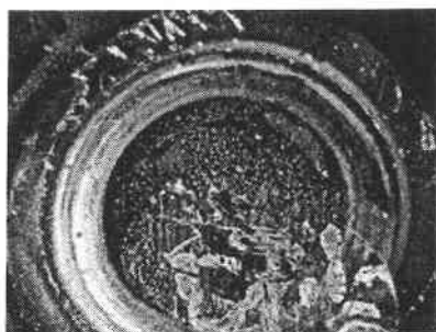
figure 16 : photographie d'un dépôt réalisé sur un substrat constitué de tungstène
