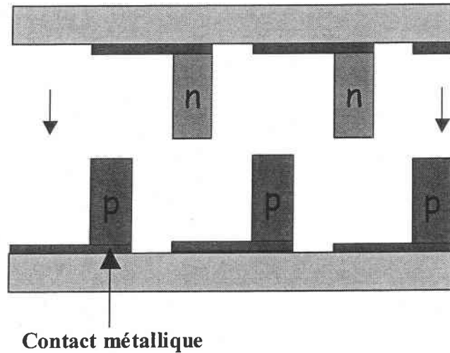
figure 3 : concept basé sur l'assemblage de deux wafers
