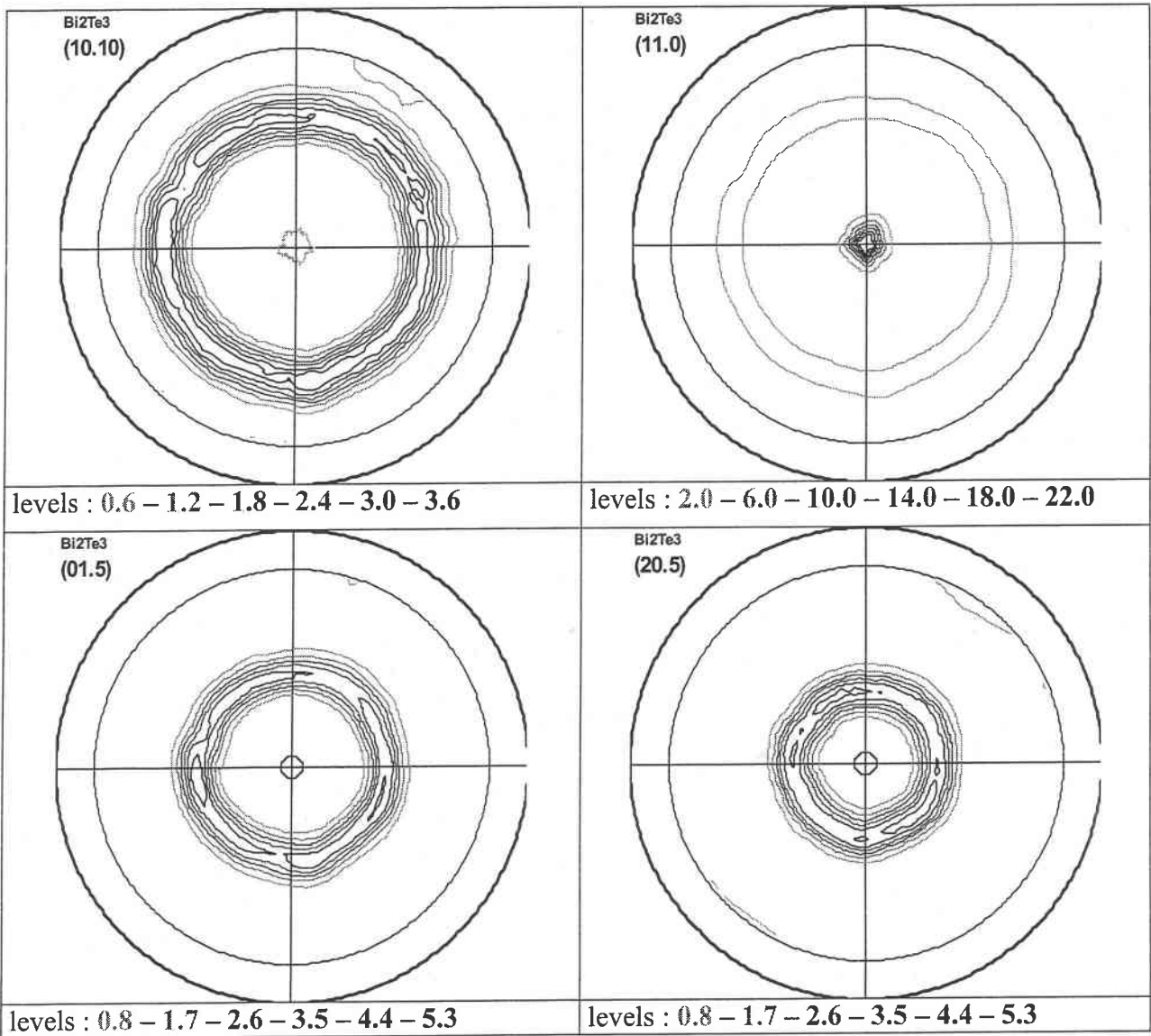
figure 14 : figure de pôles obtenue pour un composé électrodéposé à partir d'un électrolyte contenant 55% Bi ( 10^{-2} M) – 41% Te ( 7,5 \cdot 10^{-3} M) – 4% Se ( 7,3 \cdot 10^{-4} M) et à un potentiel de -105 mV/ECS
