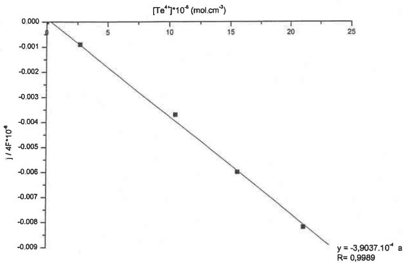
figure 10 : évolution du rapport j/4F pour différentes concentrations en tellure à un potentiel de -250 \text{ mV/ECS}
