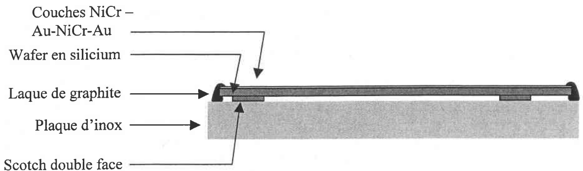
figure 25 : représentation schématique en coupe de l'ensemble de l'électrode de travail
