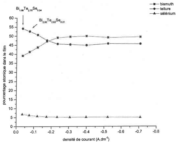
figure 18 : évolution de la stœchiométrie en fonction de la densité de courant appliquée pour un électrolyte contenant 55% Bi ( 2.10^{-2} M) – 41% Te ( 1,5.10^{-2} M) – 4% Se ( 1,4.10^{-3} M) , i_{imp} = - 0,2 A, t = 15 min
