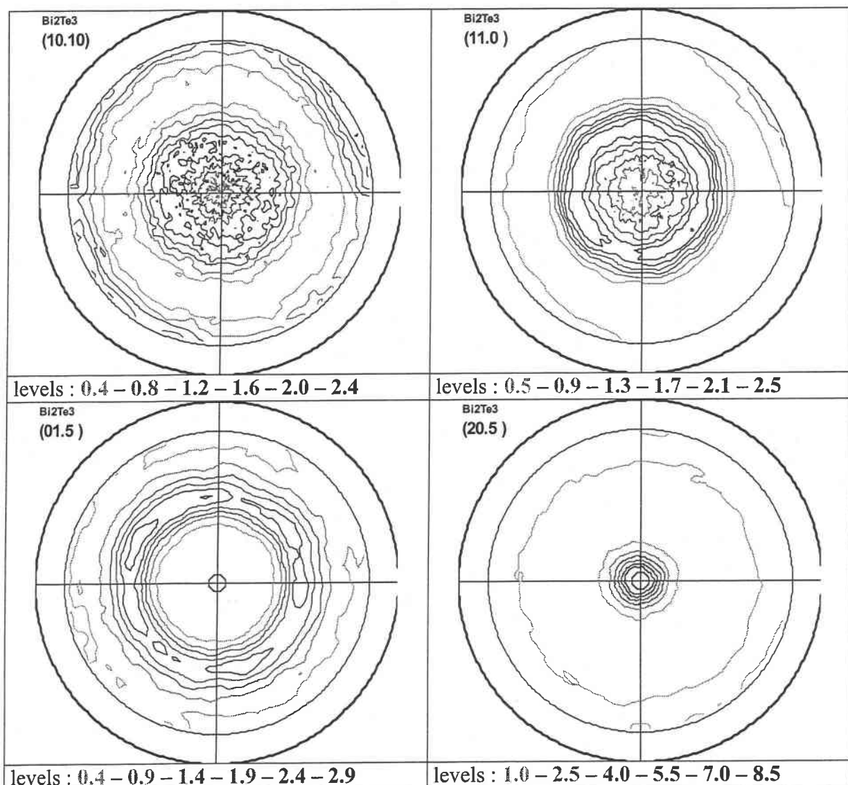
figure 22 : figures de pôles d'un dépôt obtenu à partir d'une solution de composition 60% Bi ( 2.10^{-2} M) – 36% Te – 4% Se et j = - 0,35 \text{ A.dm}^{-2}
