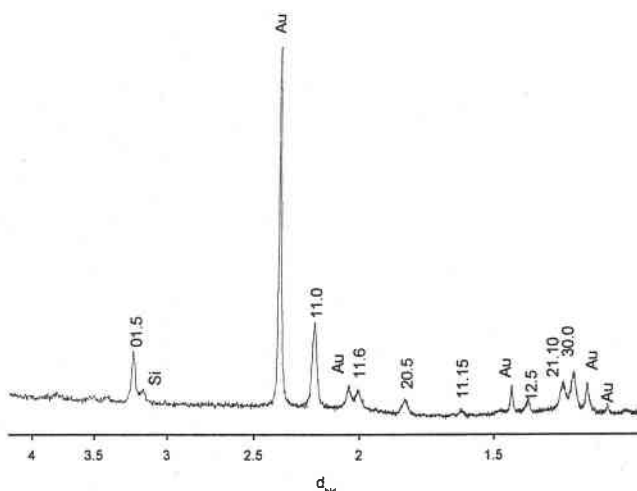
figure 22 : cliché de diffraction des rayons X réalisé sur un composé électrodéposé à partir d'une solution constituée de 60% Bi – 36% Te – 4% Se à une concentration de 2.10^{-2} M en bismuth pendant un temps de 2h, à j = -0,28 \text{ A.dm}^{-2} , sur un support constitué Si / SiO 2 / NiCr (30 nm) / Au (70 nm)
