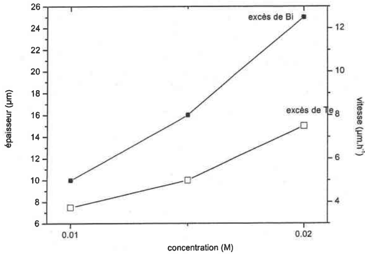
figure 22 : évolution de l'épaisseur et de la vitesse de dépôt dans le cas d'un composé électrodéposé, à partir d'une solution de rapport Bi/Te = 1, présentant un déficit en tellure et dans le cas d'un composé présentant un excès en tellure en fonction de la concentration
