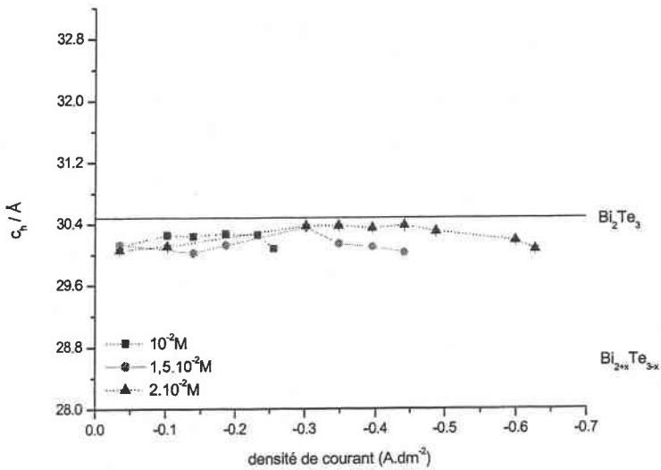
figure 35 : évolution des paramètres de maille en fonction de la densité de courant pour une solution de rapport Bi/Te = 1 à des concentrations de 10^{-2} M , 1,5 \cdot 10^{-2} M et 2 \cdot 10^{-2} M
