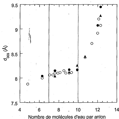
Figure 35 : Evolution de la réflexion d_{003} expérimentale en fonction du nombre de molécules d'eau par anion. Cercles : D_2O , triangles : H_2O ; symboles pleins : diffraction des neutrons ; symboles ouverts : diffraction des rayons X.
