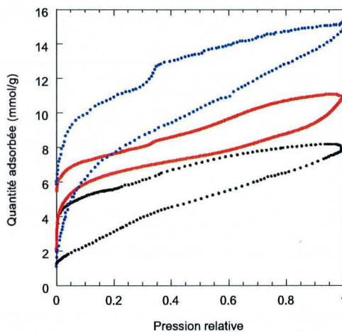
Figure 53 : Comparaison des isothermes d'adsorption d'eau des trois takovites étudiée, exprimées en nombre de molécules d'eau par anion. Noir : takovite 2SO 4 ; Rouge : takovite 4SO 4 ; Bleu : takovite 8SO 4 .
