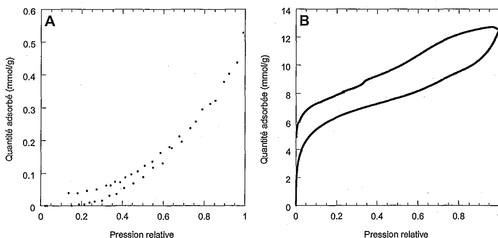
Figure 28 : Comparaison entre les isothermes d'adsorption à l'azote (A) et à l'eau (B) obtenus pour la takovite 4SO 4 .
