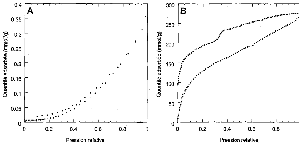
Figure 51 : Comparaison entre les isothermes d'adsorption à l'azote (A) et à l'eau (B) de la takovite 8SO4.
