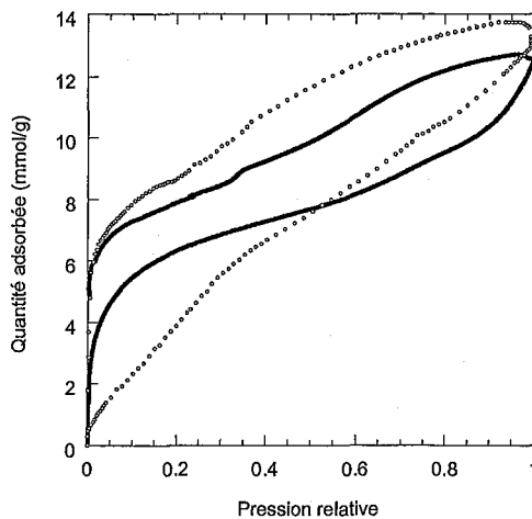
Figure 29 : Comparaison des isothermes d'adsorption d'eau des takovites 2SO4 (pointillés) et 4SO4 (trait continu).
