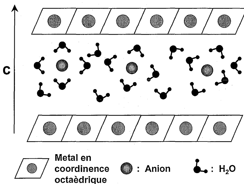
Figure 1 : Schéma de la structure théorique d'une phase HDL.
