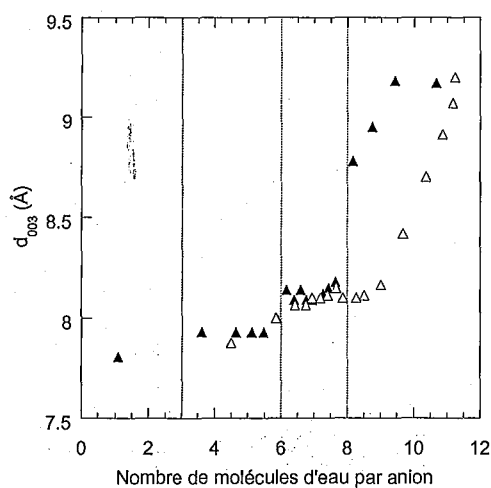
Figure 33 : Evolution de la position de la réflexion d_{003} en fonction du nombre de molécules d'eau par anion.
