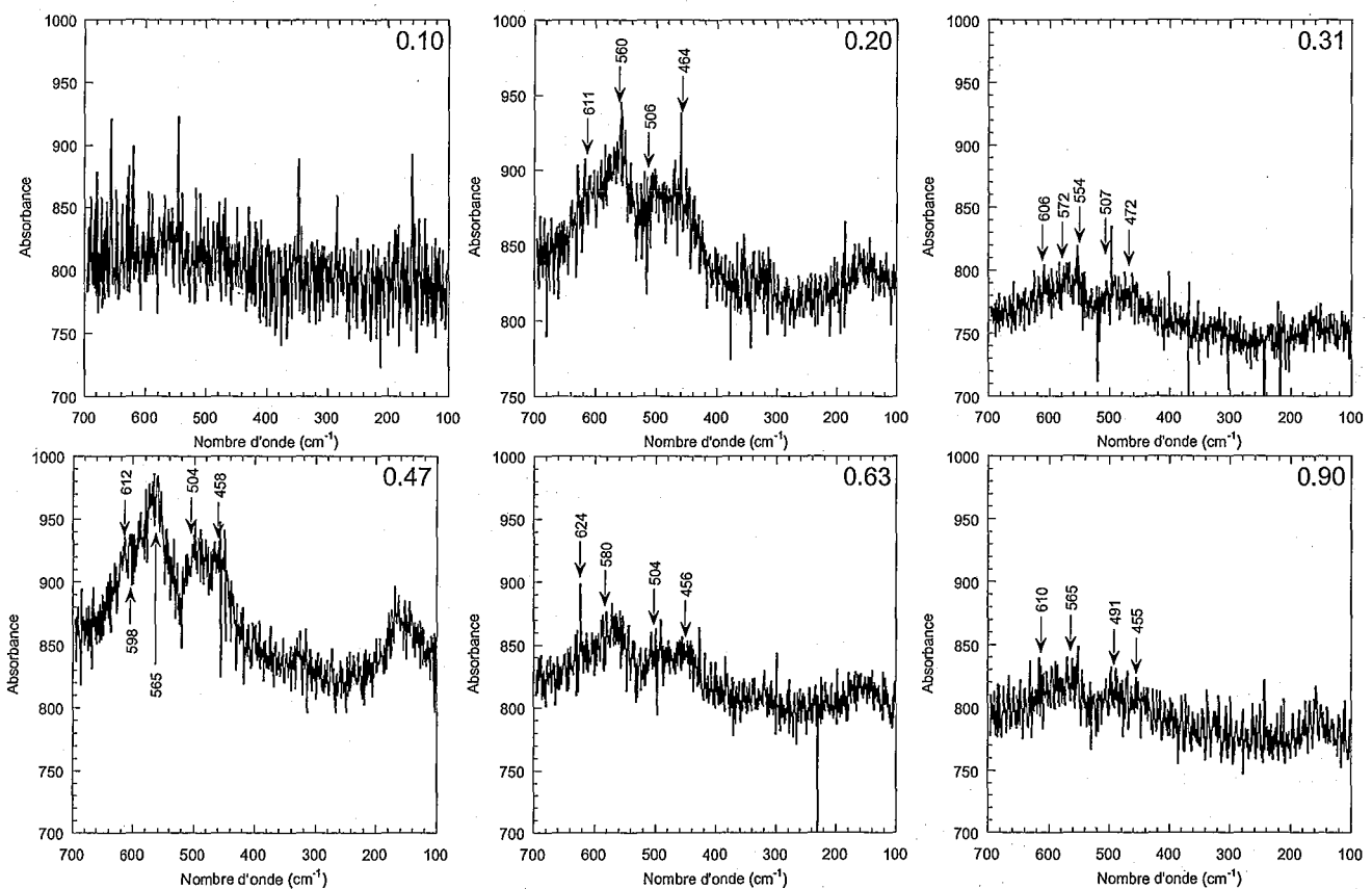
Figure 18 : Spectres Raman de la takovite 2SO_4 entre 100 et 700\text{ cm}^{-1} pour différentes pressions relatives.
