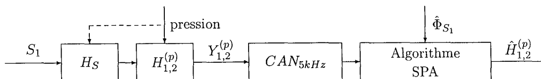
FIG. 2.13 – Protocole de mesure – estimations des fonctions de transfert \hat{H}_{1,2}^{(p)} en fonction de la pression d'appui.
