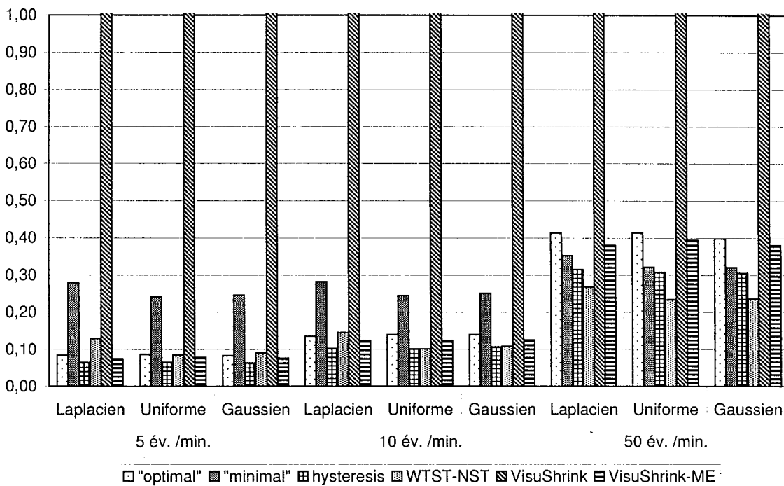
FIG. B.2 – Valeurs détaillées du critère EQM pour les 6 algorithmes testés, pour un bruit additif coloré, en fonction du type de signal et de la distribution du bruit.
