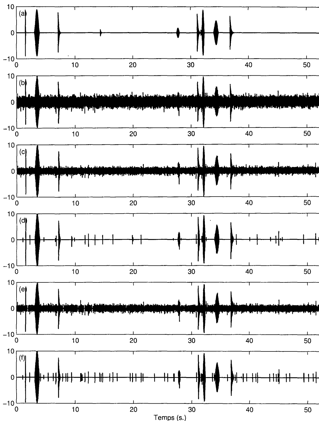
FIG. 3.22 – Résultats comparatifs du débruitage pour un bruit additif blanc, de distribution laplacienne : (a) signal d'origine ; (b) signal bruité ; signaux débruités par (c) algorithme "minimal", (d) algorithme par hystérésis, (e) WTST-NST, (f) VisuShrink . Le résultat fourni par l'algorithme "optimal" n'est pas présenté ici, car le signal est visuellement indistinct de (d). Le même argument est valable pour l'algorithme VisuShrink-ME , étant donné qu'il s'agit d'un bruit additif blanc.
