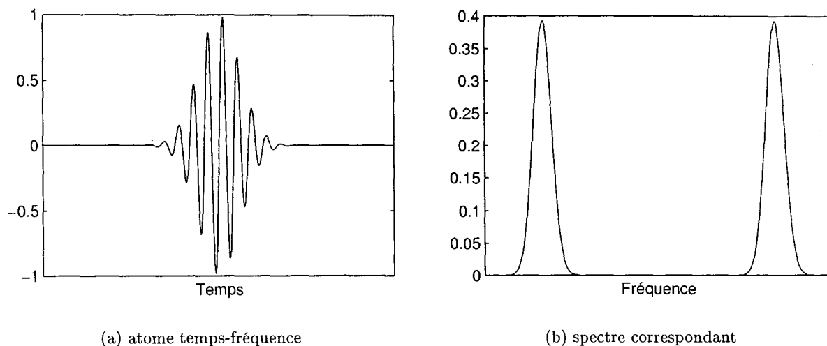
FIG. 3.4 – Exemple d'atome temps-fréquence de Gabor
