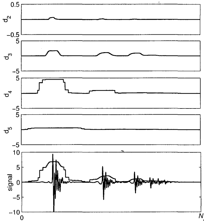
FIG. 4.5 – Envelopes des échelles de détails (pour les échelles non-nulles) et de l'événement reconstruit. L'enveloppe de l'échelle d_2 est agrandie 10 fois.
