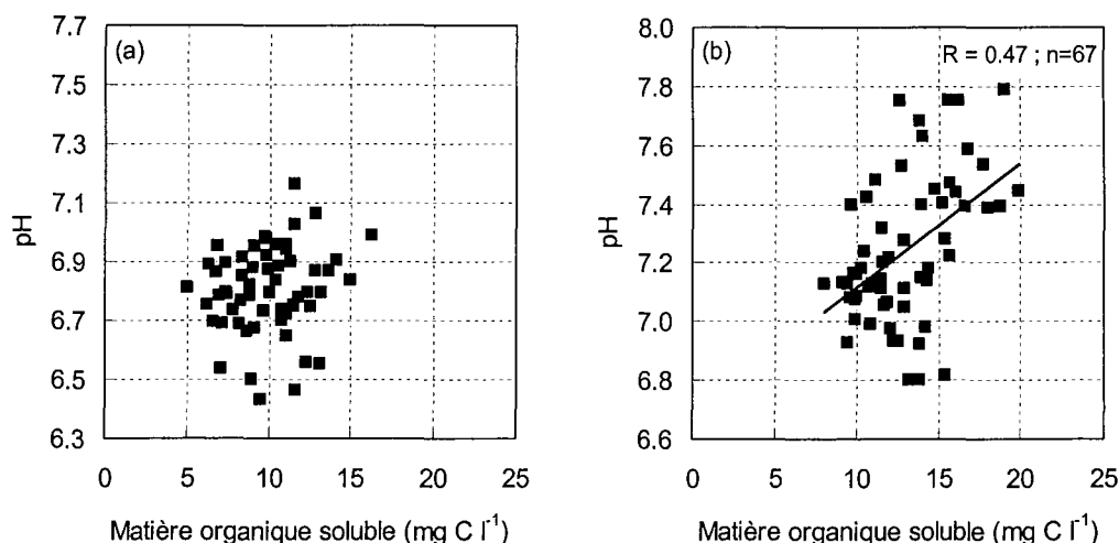
Figure 4.13 : Relation entre l'évolution du pH dans la solution du sol et la concentration des matières organiques solubles (mg C l -1 ) dans les terres non cultivées (a) et cultivées avec Thlaspi caerulescens (b) (N=67)
