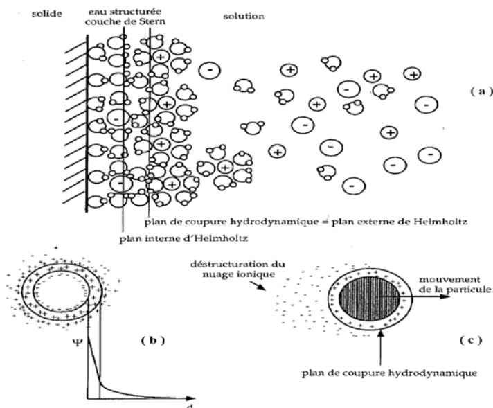
Figure 2. 8: Double couche et potentiel zêta. Cas d'une particule chargée.
