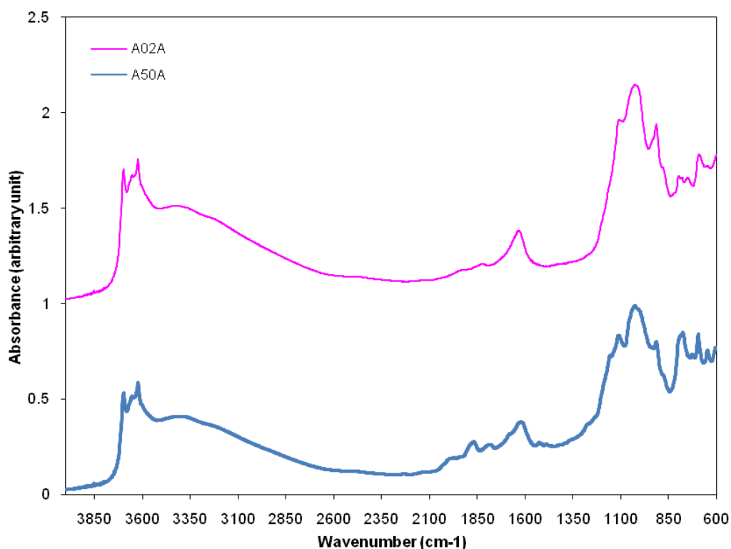
Figure 3.5 : Spectres IR des échantillons de l'argile alluviale traitée à l'acide chlorhydrique.
