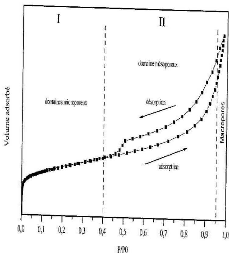
Figure 2.9 : Remplissage des différentes classes de pores le long d'une isotherme d'adsorption-désorption d'azote.
