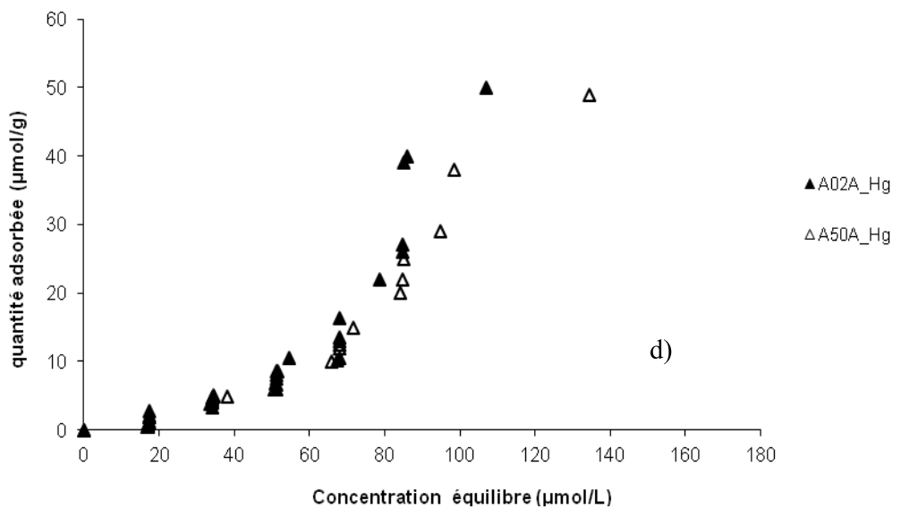
Figure 4.6 : Influence de l'activation acide sur l'adsorption des cations métalliques par la fraction argileuse (<math><2\mu\text{m}</math>) et la fraction sablonneuse (<math><50\mu\text{m}</math>).
