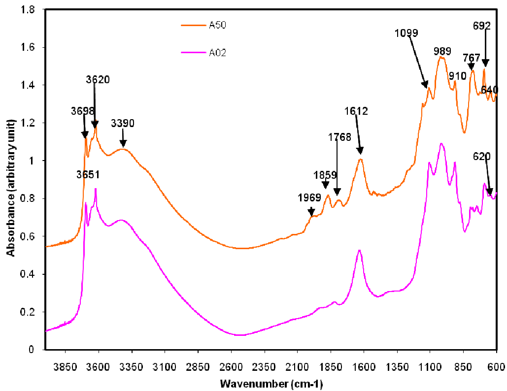
Figure 3.4 : Spectres IR des échantillons de l'argile alluviale.
