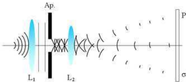
Figure 2.7 : Exemple de dispositif de diffusion en optique.
