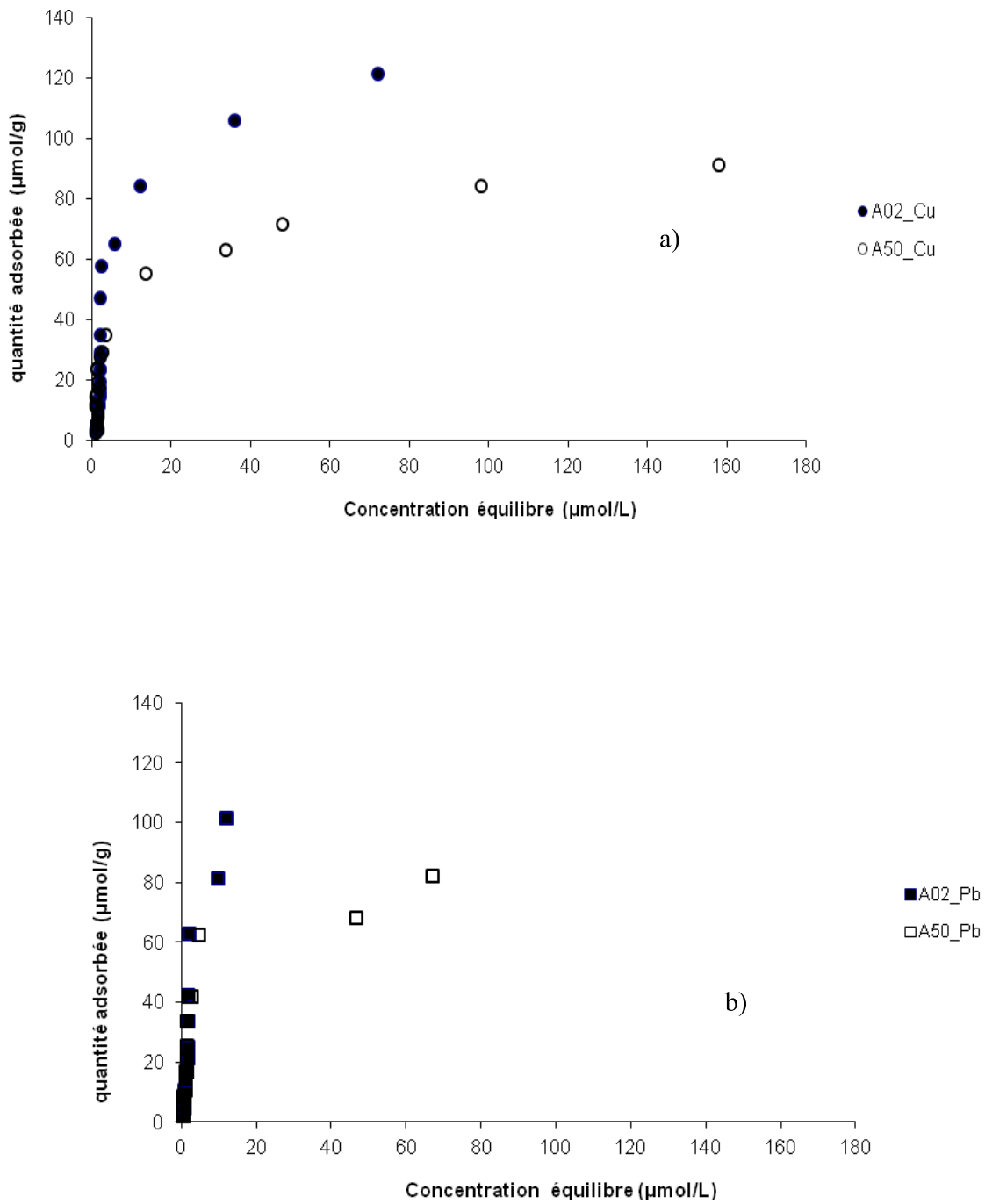
Figure 4.2 Isothermes d'adsorption du \text{Cu}^{2+} et du \text{Pb}^{2+}
