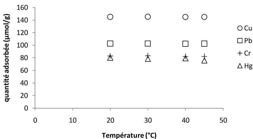
Figure 4.4: Effet de la température sur l'adsorption des 4 sels métalliques.
