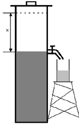
Figure 2.4 : Allonge de sédimentation
