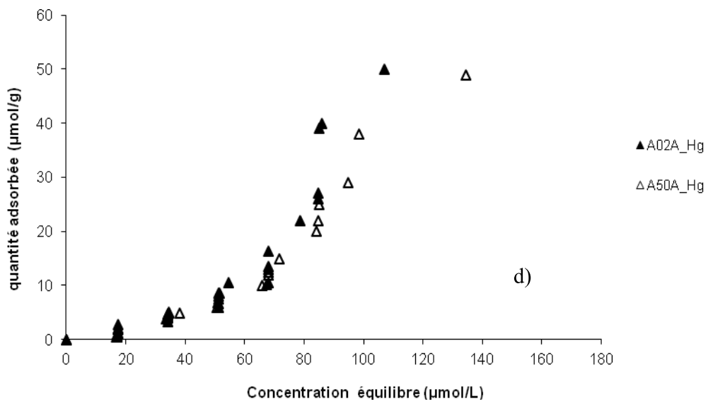
Figure 4.6 : Influence de l'activation acide sur l'adsorption des cations métalliques par la fraction argileuse (<2µm) et la fraction sablonneuse (<50µm).
