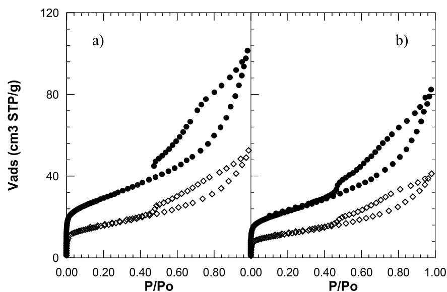
Figure 3.11 : Isotherme d'adsorption-désorption d'azote obtenue par volumétrie point par point, à 77K pour a) fraction argileuse (A02) et la fraction sableuse (A50) b) traitement acide de la fraction argileuse (A02A) et la fraction sableuse (A50A). ●: A02 ; ◇: A50
