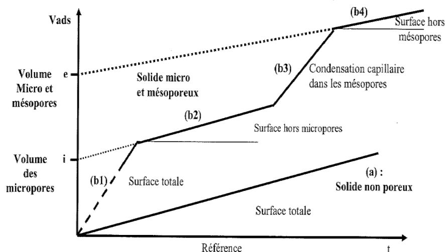
Figure 2.10 : Schéma de principe de la comparaison des isothermes par rapport à un solide de référence non poreux.
