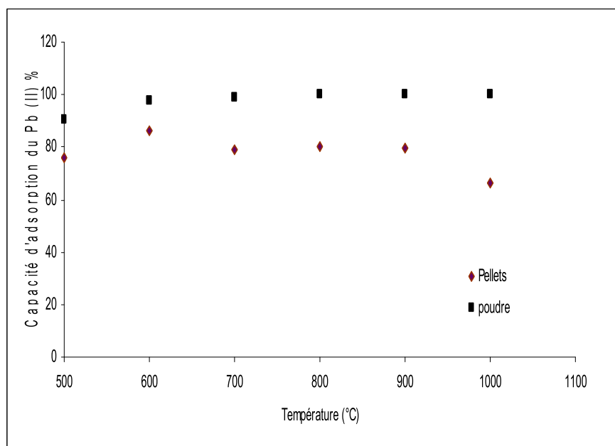
Figure 5.8 : Etude comparative de la capacité d'adsorption des boulettes et de la poudre des boulettes d'argile naturelle.
