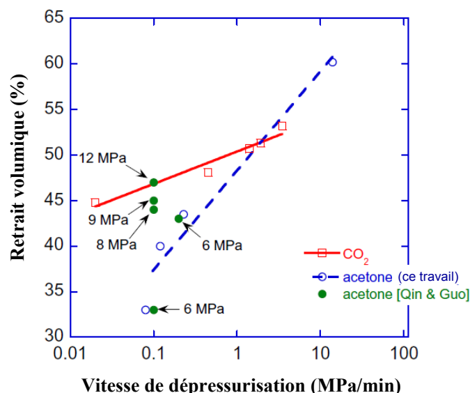
Figure 32. Impact de la vitesse de dépressurisation du CO 2 et de l'acétone sur le retrait volumique des aérogels, et comparaison avec les résultats de Qin et Guo [8].
