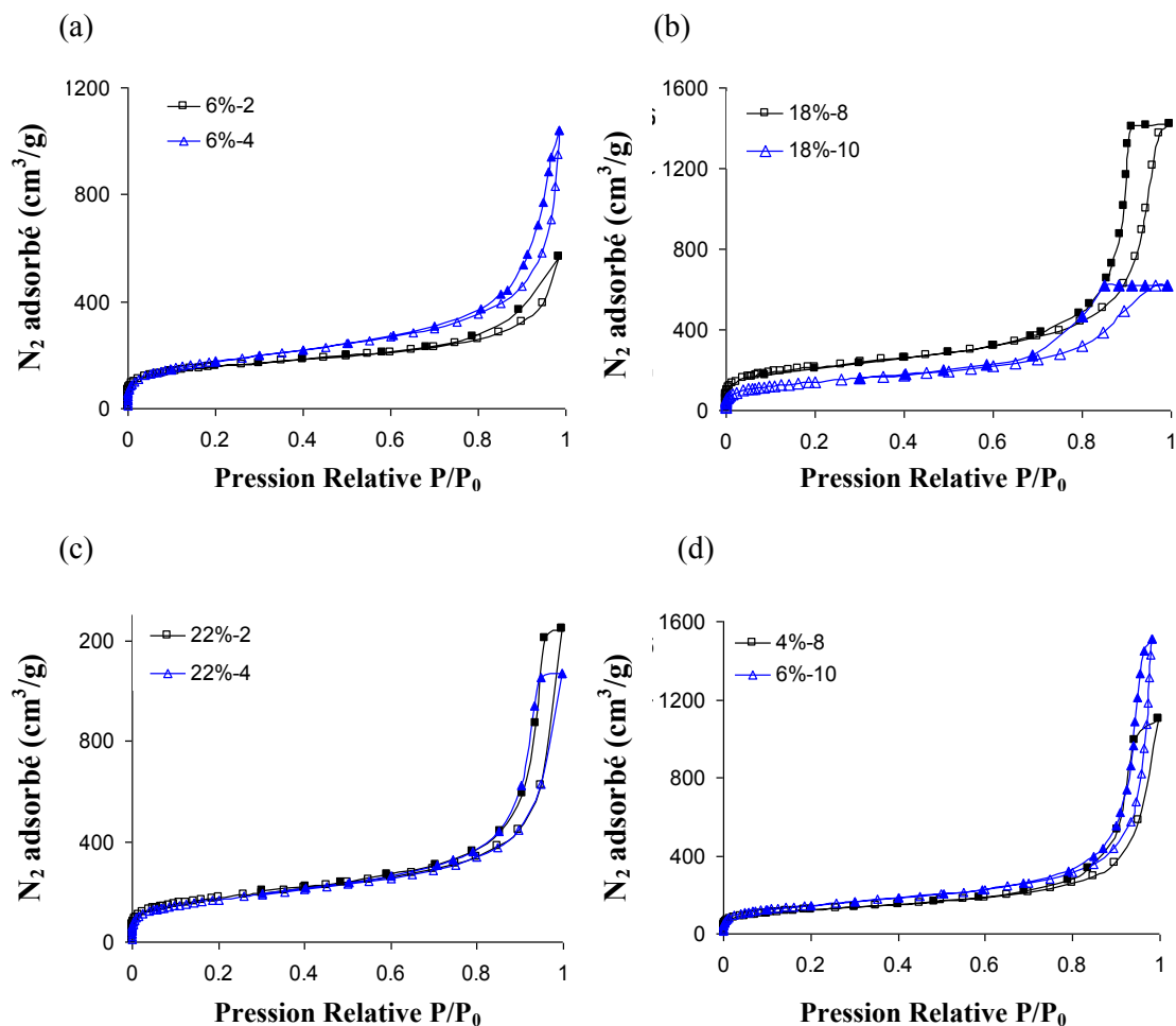
Figure 40. Isothermes d'adsorption-désorption d'azote (symboles vides et pleins, respectivement) des aérogels : (a) ATF6%-2, ATF6%-4 ; (b) ATF18%-8, ATF18%-10% ; (c) ATF22%-2, ATF22%-4 et (d) ATF4%-8 et ATF6%-10.
