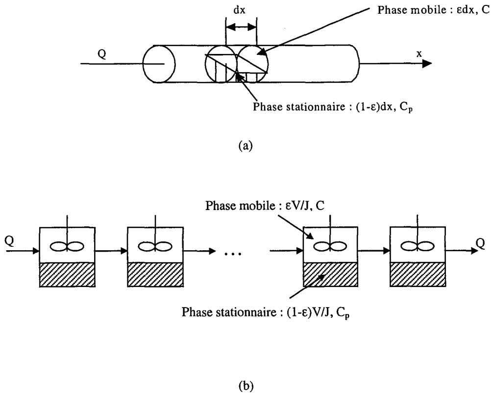
Figure 2. 3 : Représentation d'un milieu poreux selon l'approche systémique : (a): réacteur piston avec dispersion axiale ; (b) : cascade de J mélangeurs
