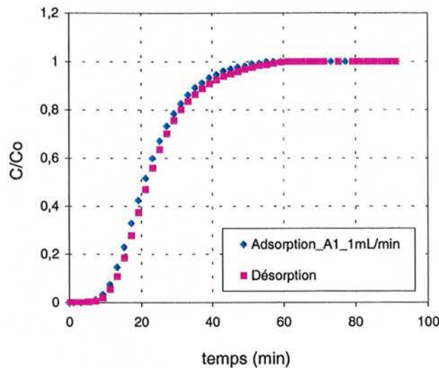
Figure 3.4 : Comparaison des fronts d'adsorption et de désorption ( 1-C/C_0 en ordonnée) pour le milieu A1 à 1 mL/min
