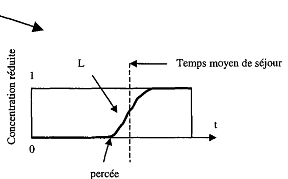
(c) : Exemple d'un front de concentration réduite d'un traceur de l'eau en sortie de colonne (abscisse L) : effet de la dispersion.
