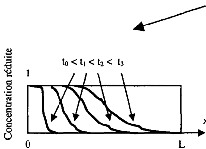
(a) : Injection d'un échelon d'un traceur de l'eau à l'entrée d'une colonne de chromatographie
