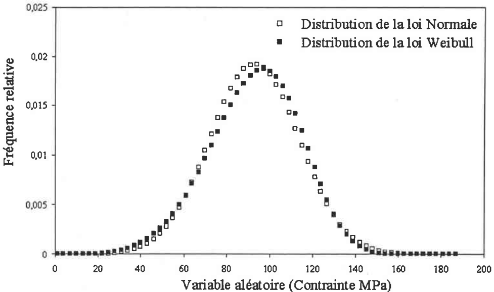
FIG. 11.1 – Comparaison de la distribution de la loi de Weibull et de la loi Normale à partir des résultats d'essais dynamiques sur cristal.
