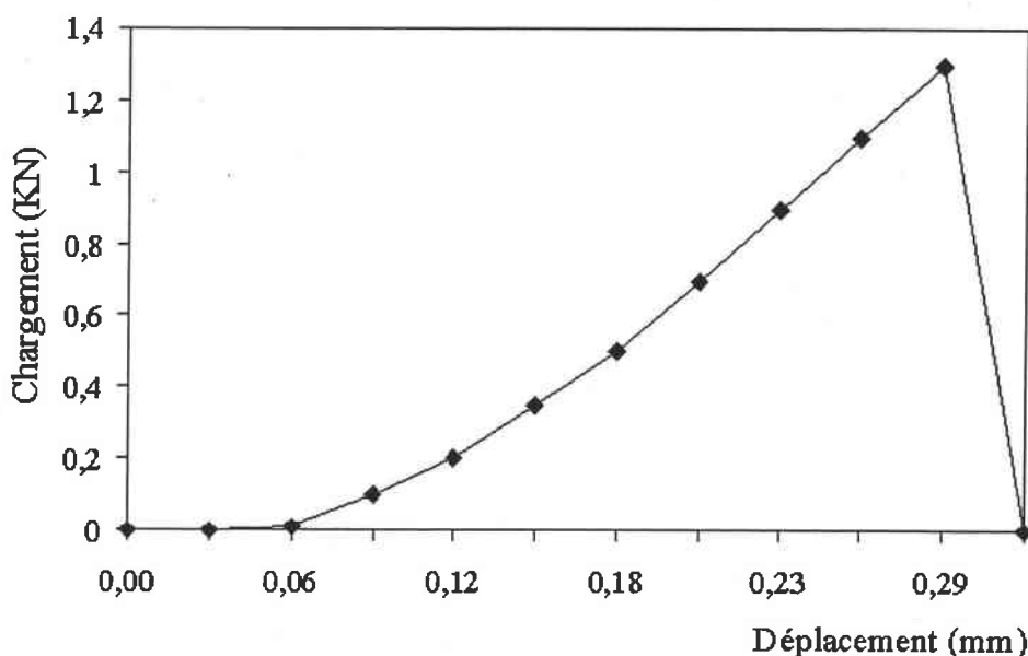
FIG. 6.2 – Courbe «charge-déplacement» obtenue sur un échantillon cristal
