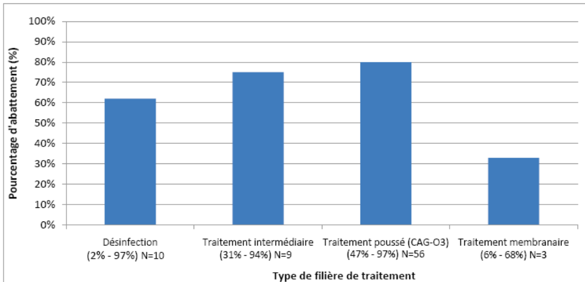
Figure I-26 : Abattements moyens des molécules en fonction des filières de traitement.
