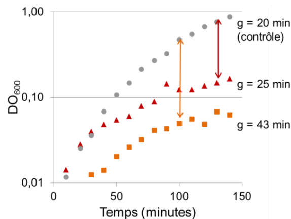
Figure II-24 : Exemple de courbes de croissance bactérienne indiquant une toxicité ( g augmentant).
