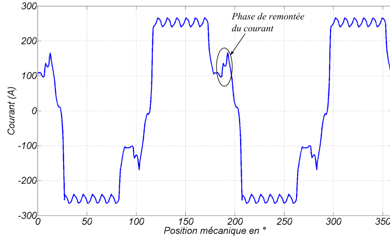
FIGURE 3.40 – Forme d’onde du courant d’une section d’induit sur un tour mécanique à 6000 \text{ tr.min}^{-1} .
