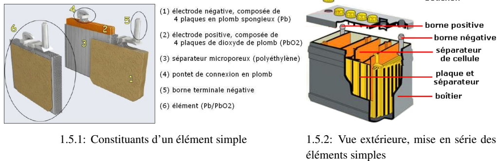
FIGURE 1.5 – Constituants d'une batterie au plomb.
