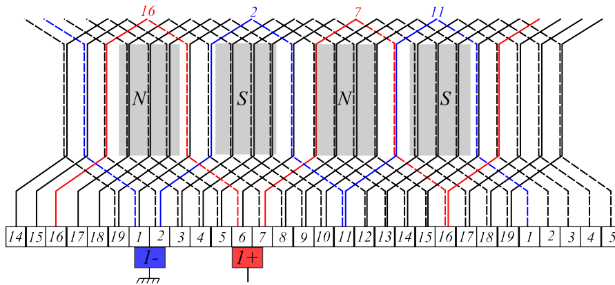
FIGURE 2.8 – Commutation d'un induct en ondulé avec 2 balais et 4 pôles.
