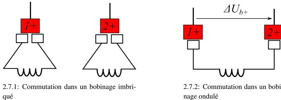
FIGURE 2.7 – Commutation sous les balais positifs (avec au moins deux balais positifs).
