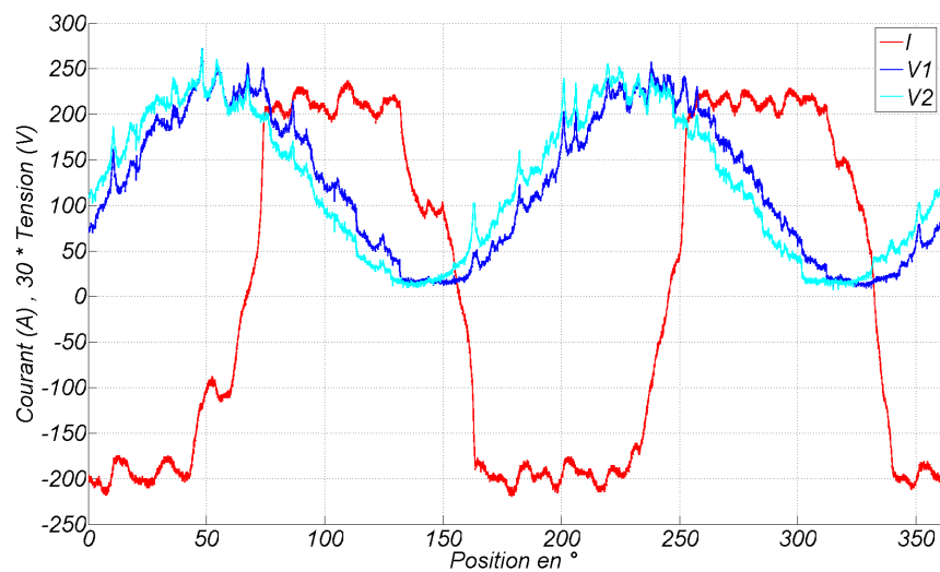
FIGURE 2.23 – Mesure du courant et de la tension d'une section d'induit sur un tour mécanique à 6000 \text{tr}\cdot\text{min}^{-1} .
