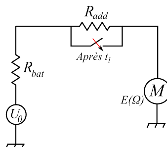
FIGURE 5.1 – Principe de diminution du courant d'appel par ajout d'une résistance.
