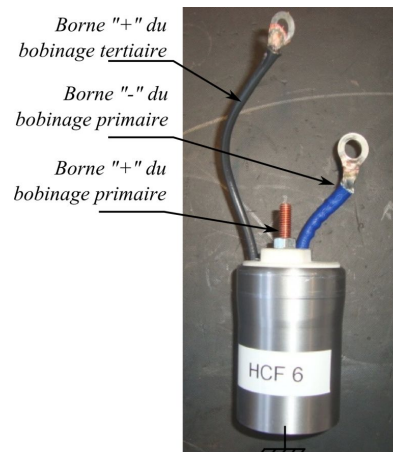
5.15.2: HCF seul, connections des bobinages
