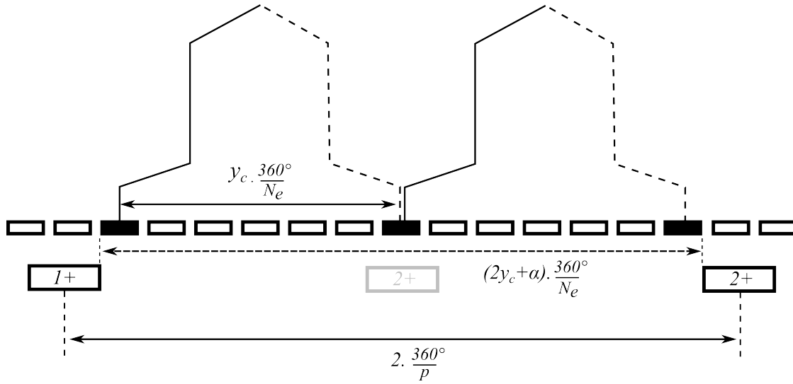
FIGURE A.4 – Schéma pour une lecture graphique de la durée de commutation dans un bobinage ondulé lorsque le nombre de balais est égal au nombre de pôles moins deux.
