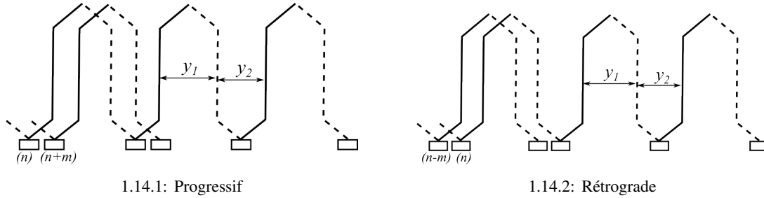
FIGURE 1.14 – Bobinage ondulé.
