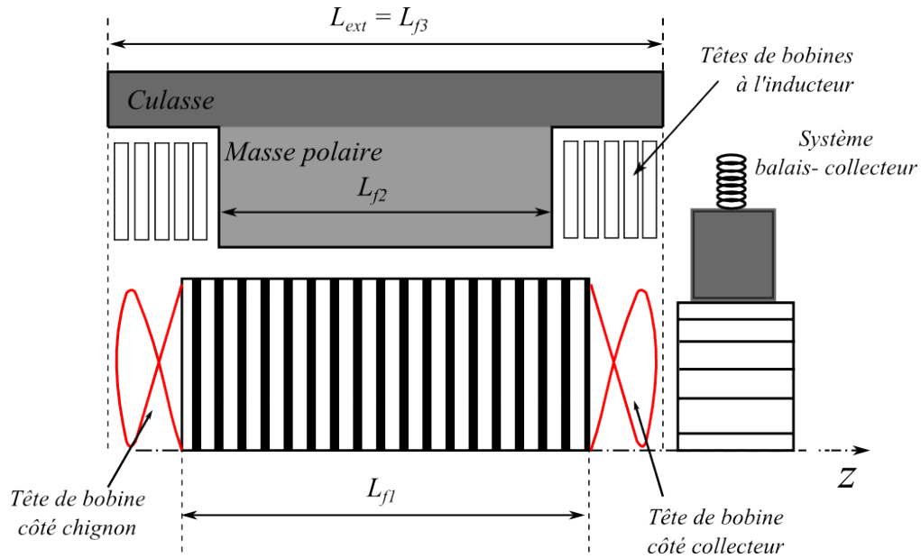
FIGURE 5.19 – Vue schématique d'une coupe longitudinale.
