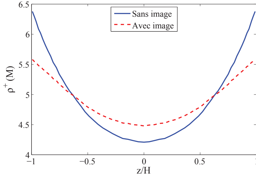
FIGURE 4.18 – Profil du cation dans le cas de contre-ion, \sigma = -0.1 \text{ C.m}^{-2} .
