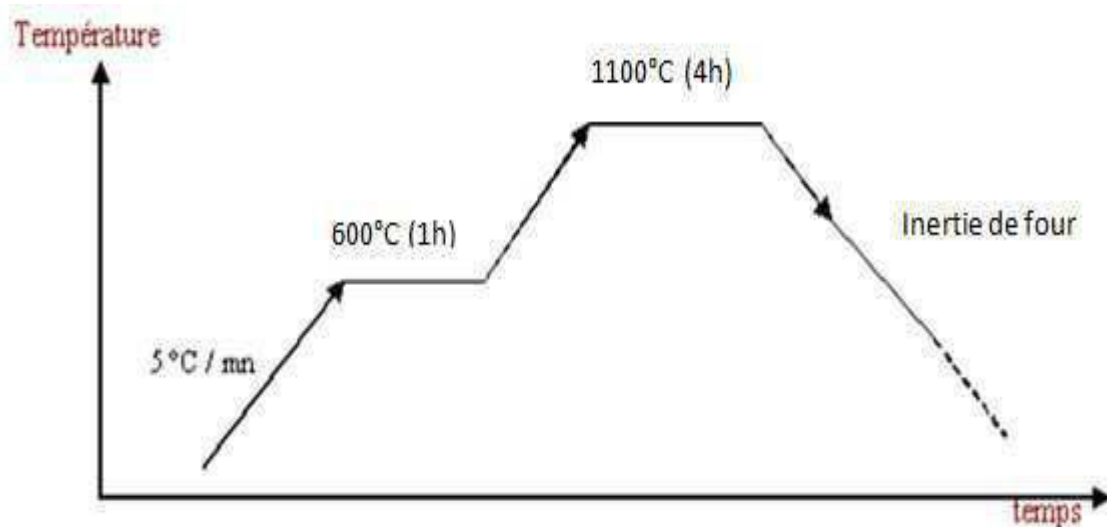
Figure III.14: Cycle de frittage des pastilles de PT:Mg x %.
