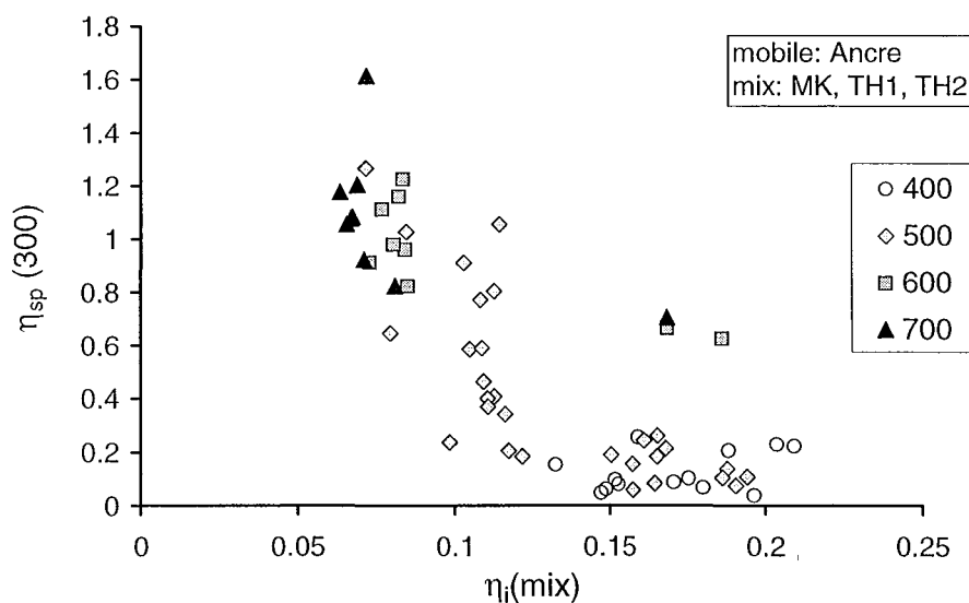
Figure IV-55. \eta_{sp}(300) en fonction de la viscosité initiale de procédé, mix MK, TH1 et TH2, à différentes vitesses de rotation.
